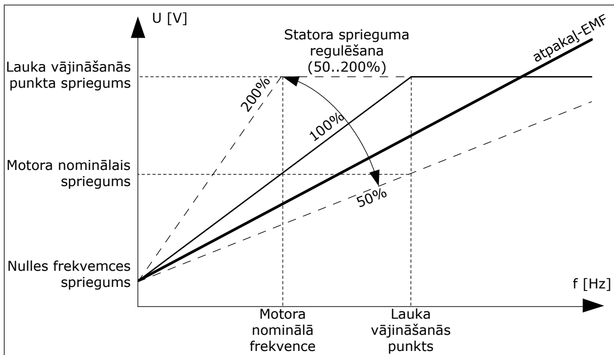
Att. 14: Statora sprieguma regulēšana
