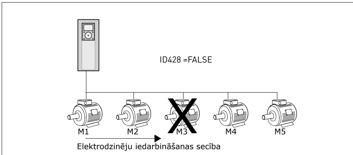
Att. 46: Bloķēšanas 2. loģika
