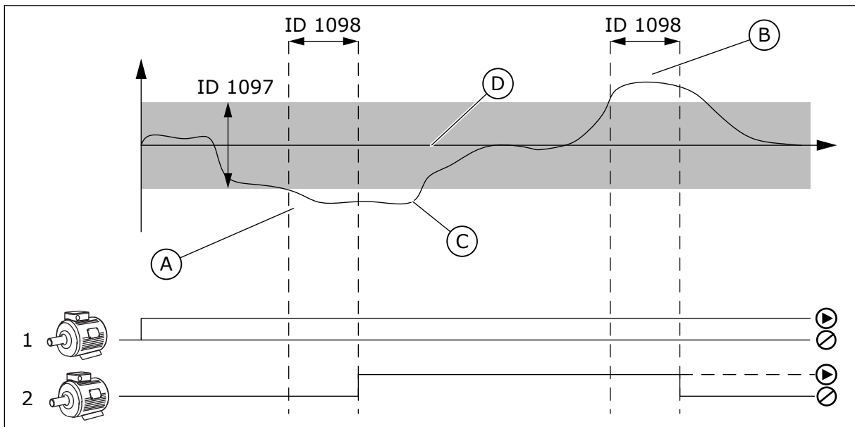
Att. 50: Papildu sūkņu sāksšana vai apturēšana (P3.14.8 = joslas platums, P3.14.9 = joslas platuma aizkave)
