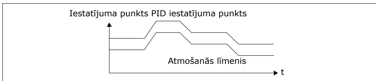
Att. 39: Atmošanās režīms: relatīvais iestatījuma punkts
