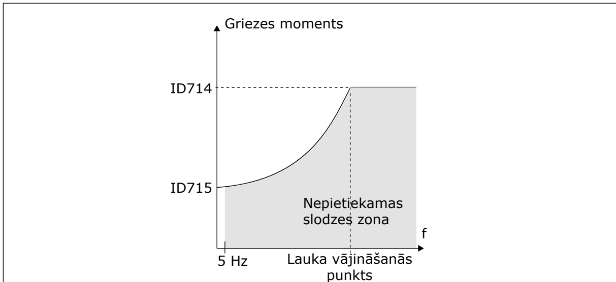
Att. 31: Minimālās slodzes iestatīšana
