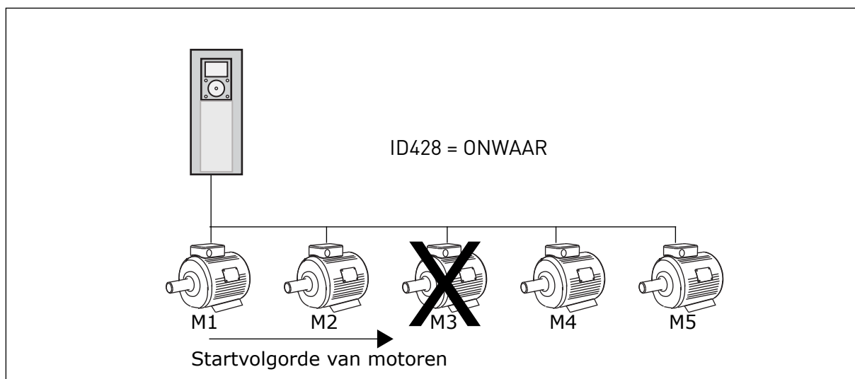
Afb. 46: Vergrendelingslogica 2
