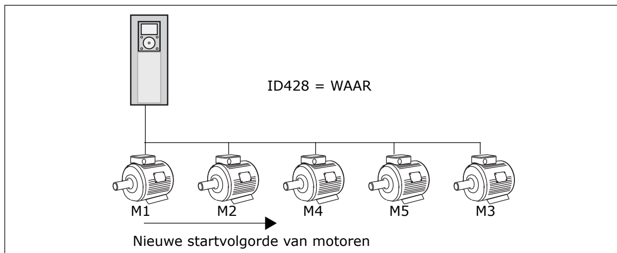
Afb. 47: Vergrendelingslogica 3
