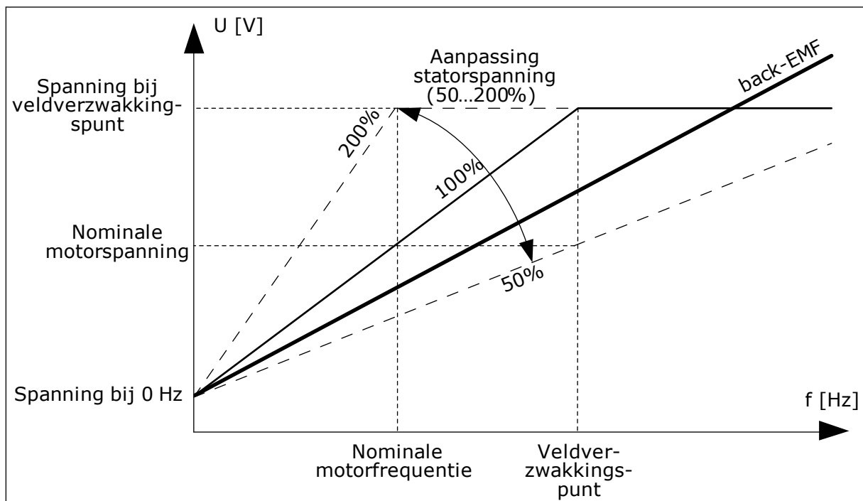
Afb. 14: Aanpassing van de statorspanning
