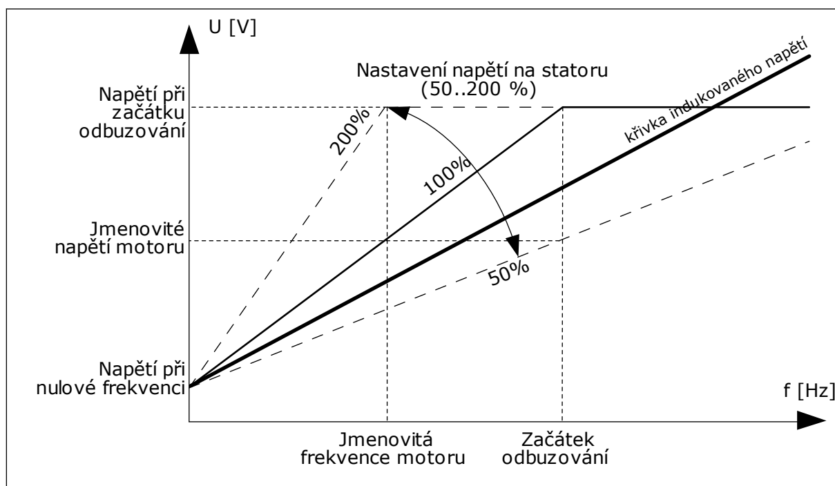
Obr. 14: Nastavení napětí na statoru
