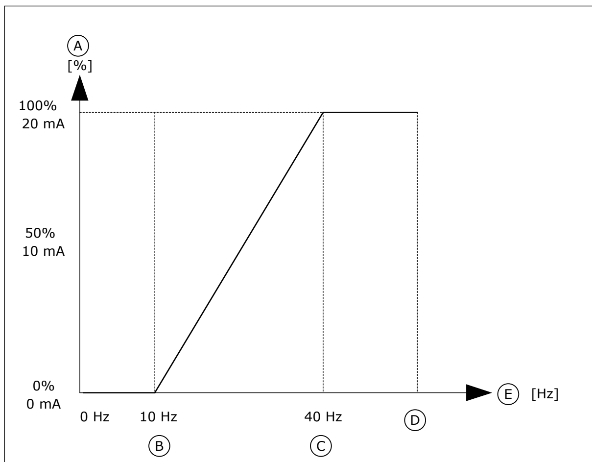
Obr. 25: Měřitko signálu A01
