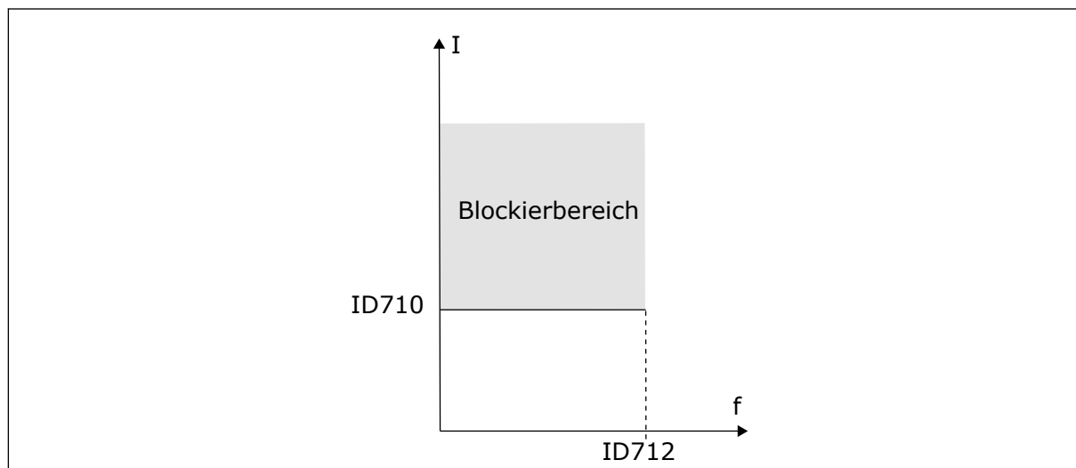
Abb. 59: Die Blockierschutzeinstellungen
