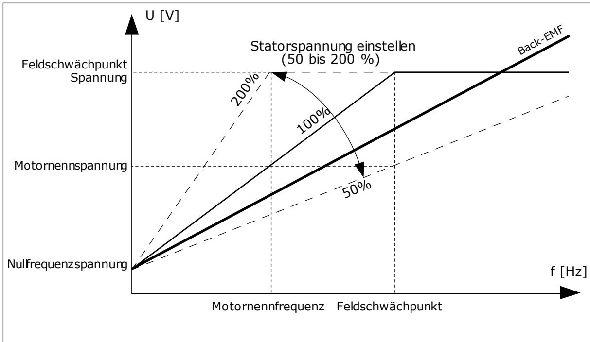
Abb. 22: Die Einstellung der Statorspannung
