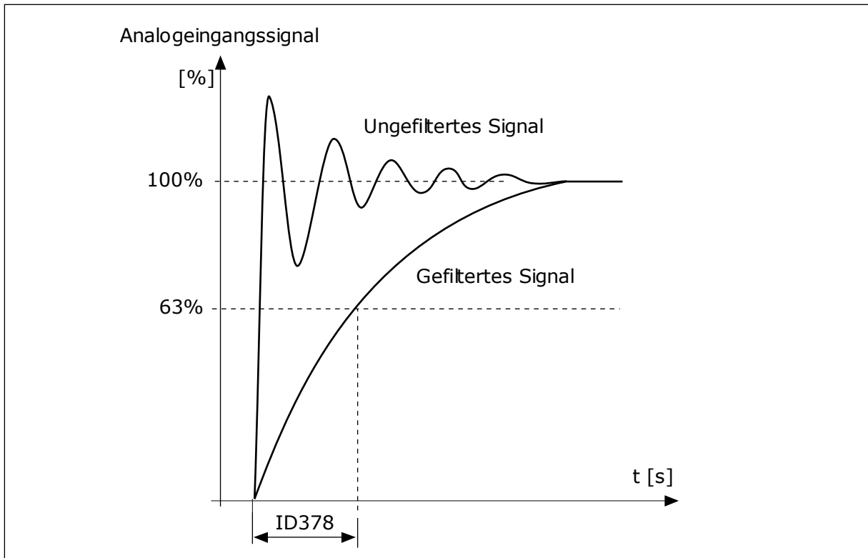
Abb. 47: Die AI1-Signalfilterung
