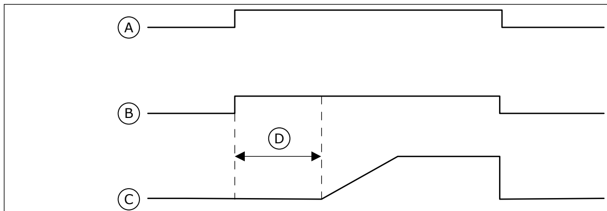
Abb. 93: Die Funktion „Ansaugpumpe“
