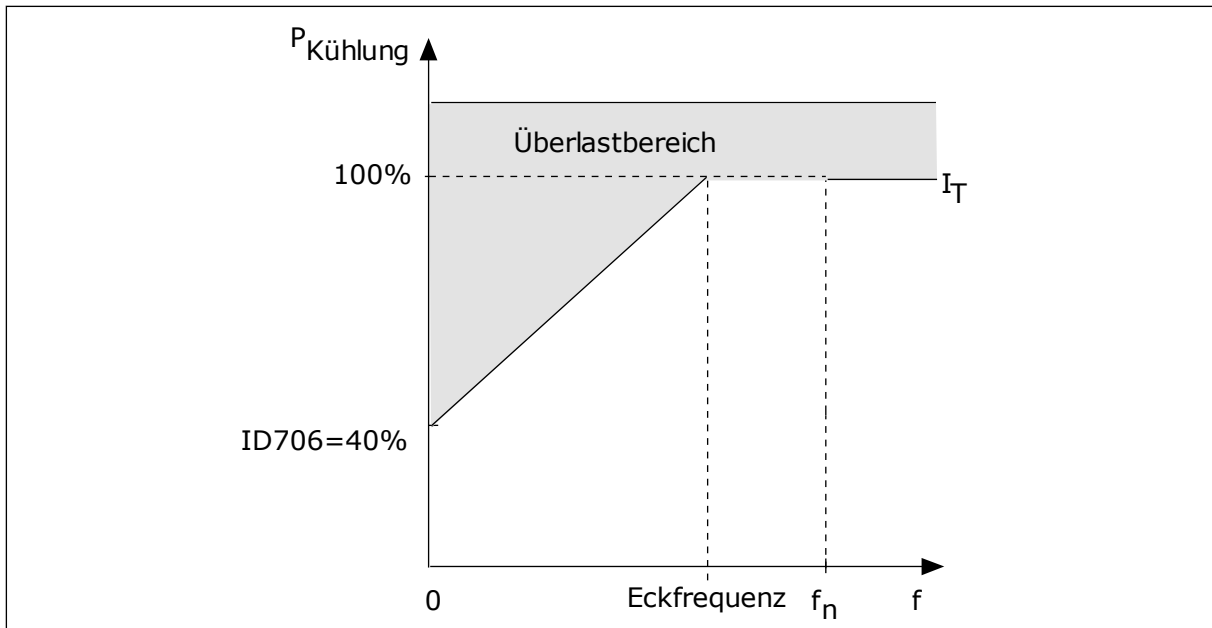
Abb. 56: Die I_T -Kurve des thermischen Motorstroms
