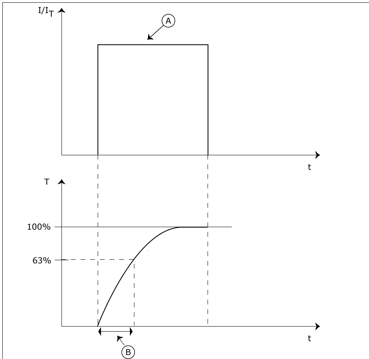
Abb. 57: Die Motor-Temperaturzeitkonstante
