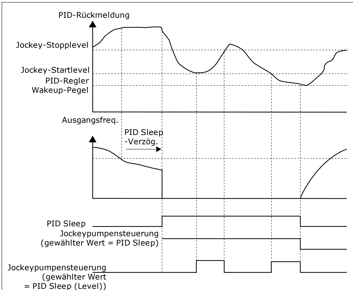
Abb. 92: Die Funktion „Jockeypumpe“
