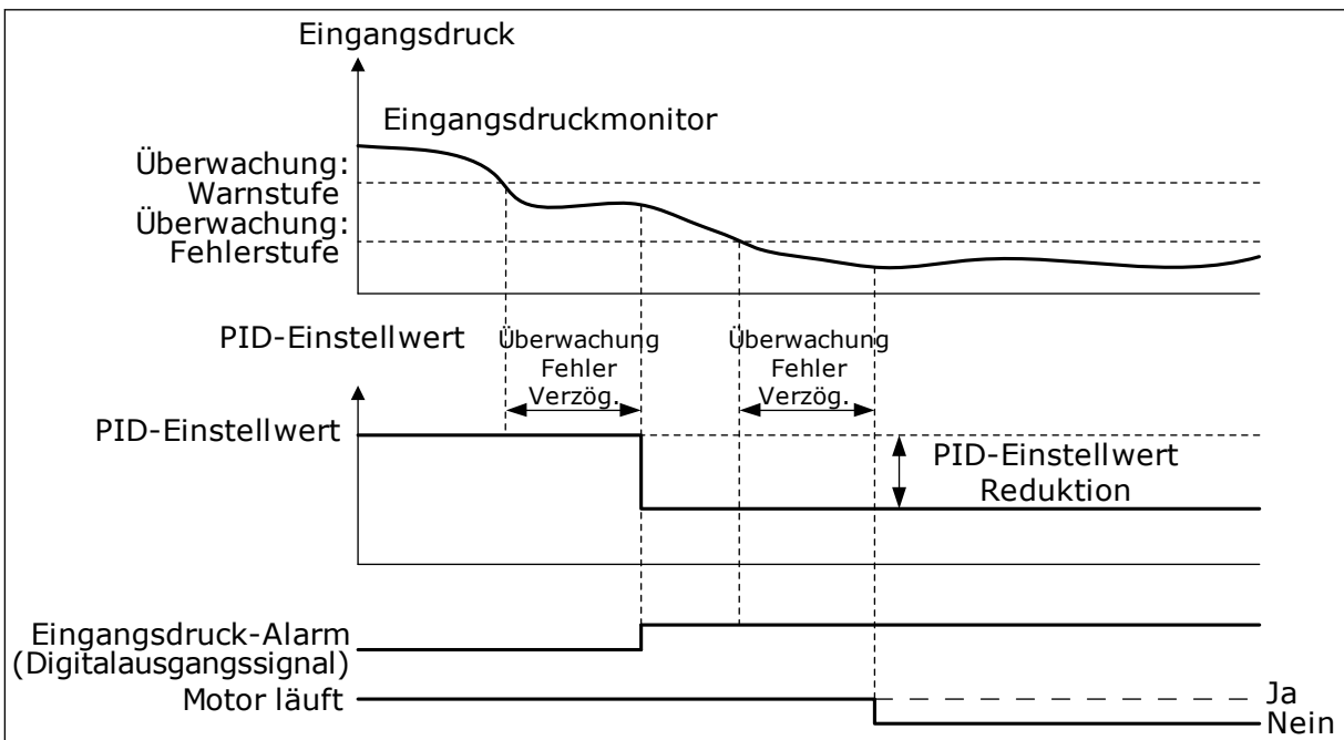
Abb. 79: Funktion „Eingangsdruküberwachung“
