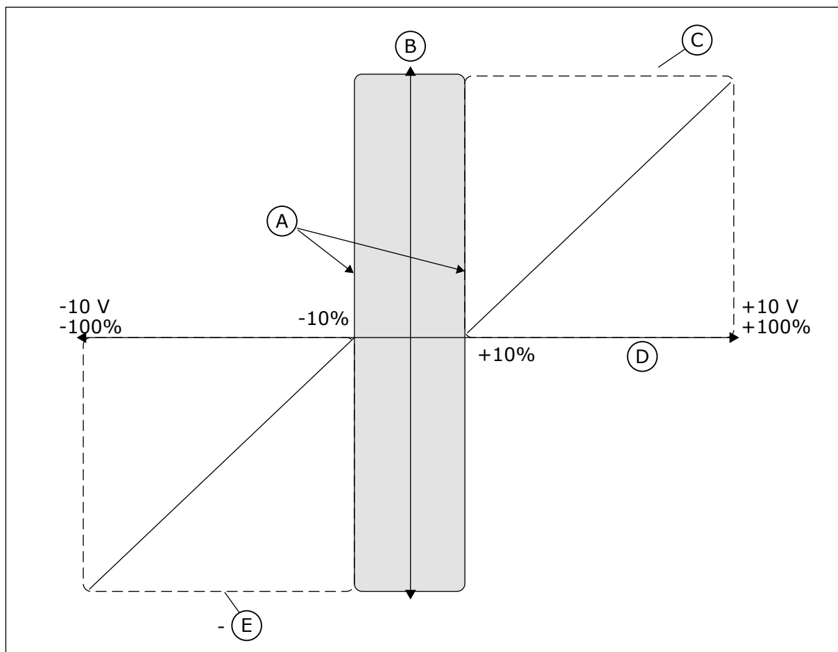
Abb. 38: Die Joystick-Funktion
