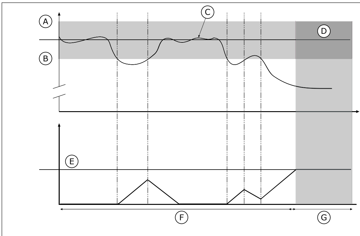
Abb. 74: Die Funktion „Rückmeldungsüberwachung“
