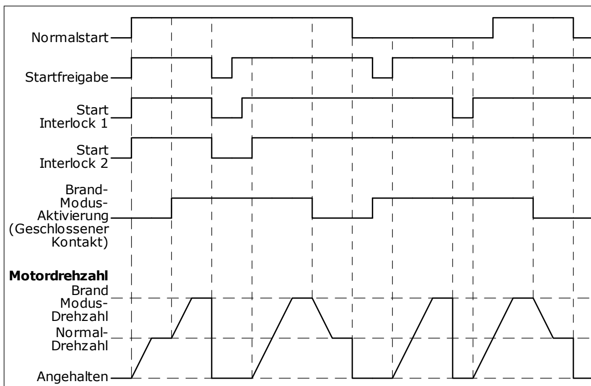
Abb. 87: Die Brand-Modus-Funktion
