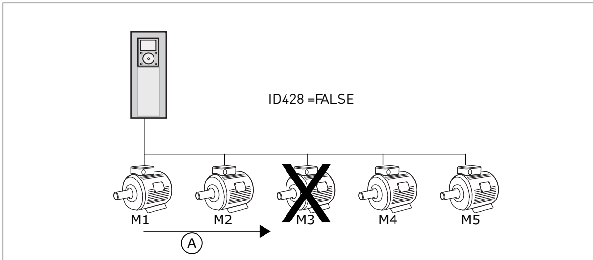
Kuva 82: Lukituslogiikka 2
