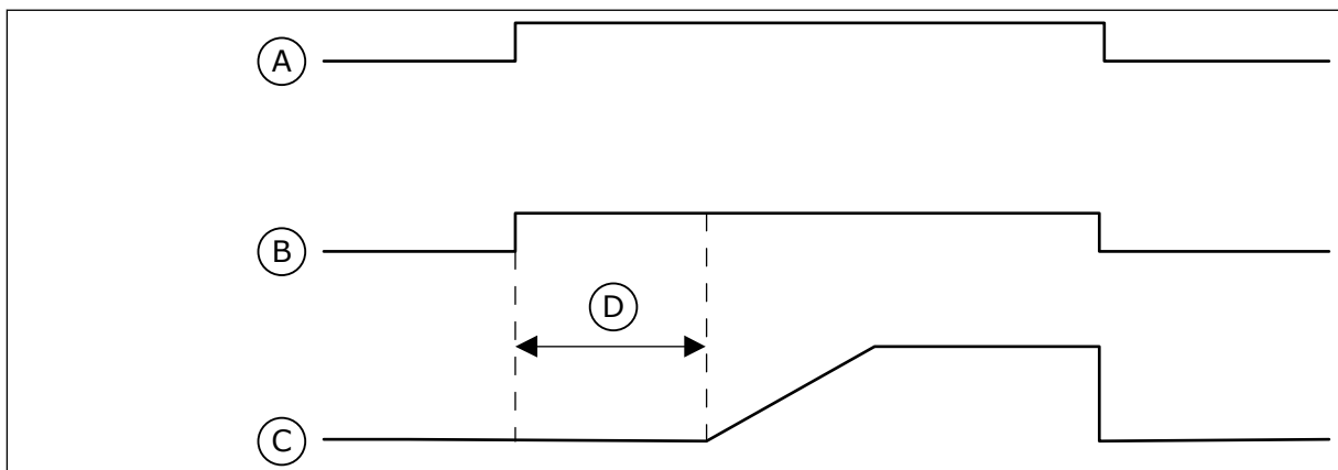
Kuva 93: Siemenvesipumpputoiminto
