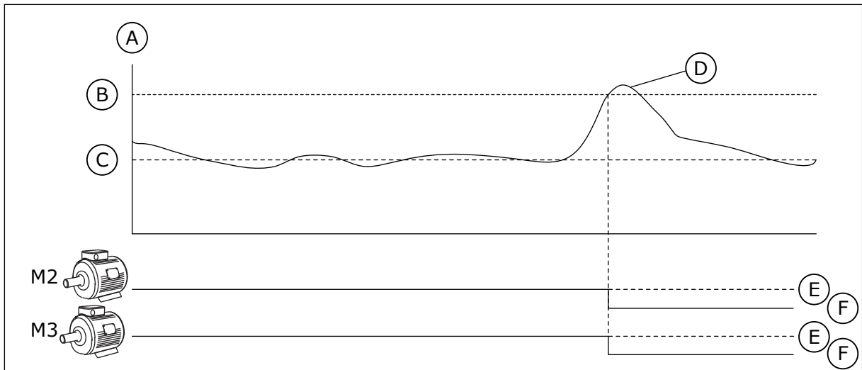
Kuva 86: Ylipaineen valvontatoiminto
