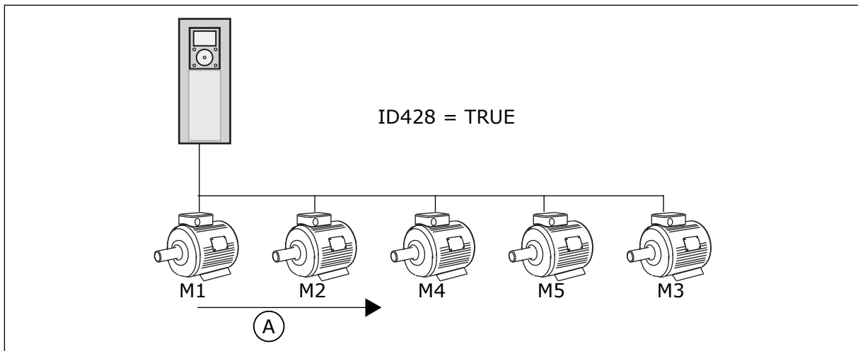
Kuva 83: Lukituslogiikka 3
