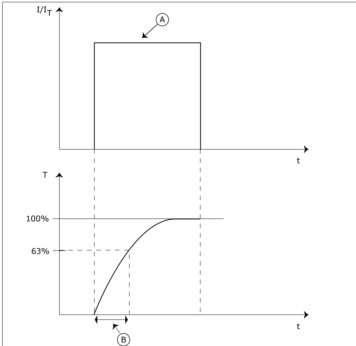
Рис. 57: Тепловая постоянная времени двигателя
