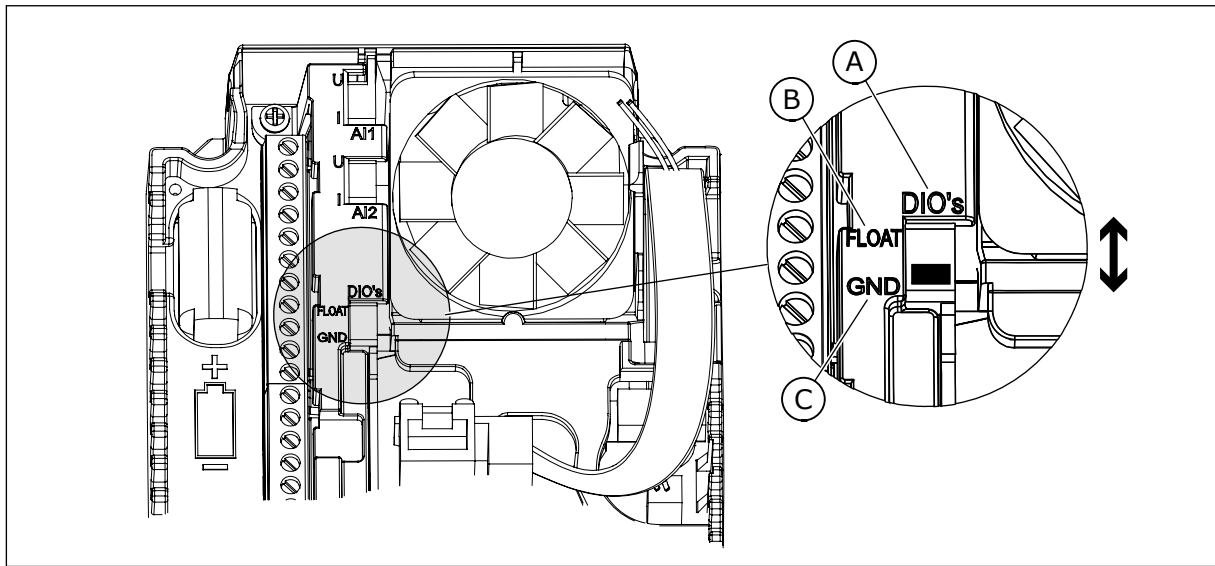
Рис. 11: DIP-переключатель
