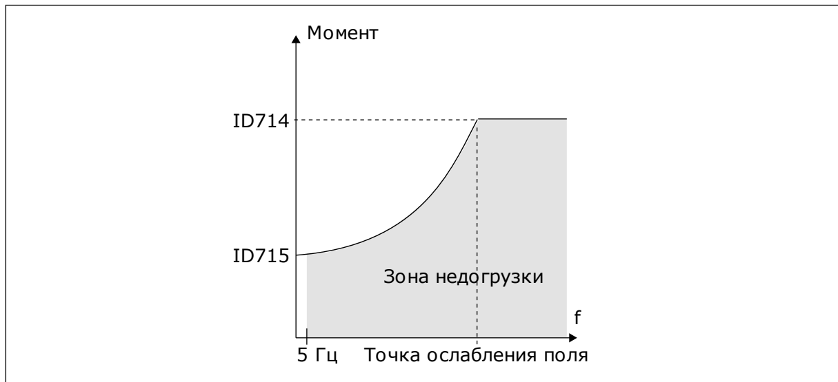
Рис. 60: Настройка минимальной нагрузки
