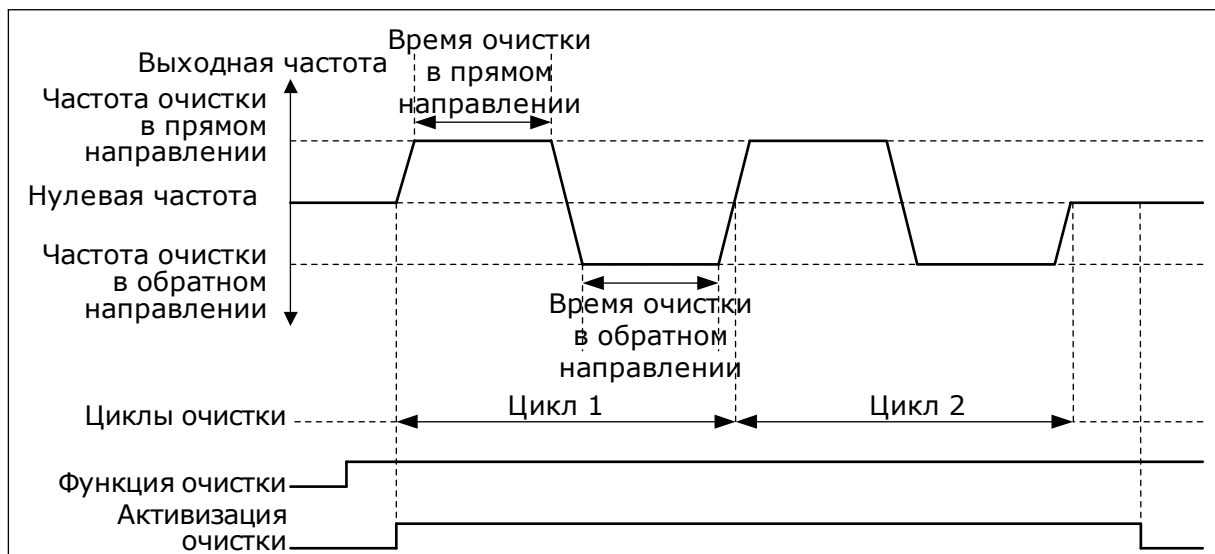
Рис. 91: Функция автоматической очистки
