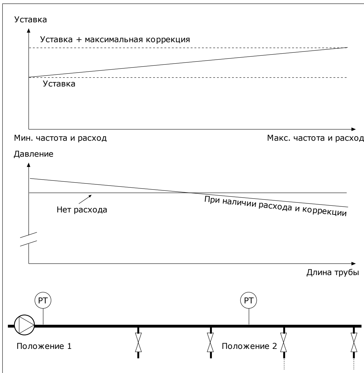
Рис. 76: Уставка 1, обеспечивающая компенсацию падения давления
