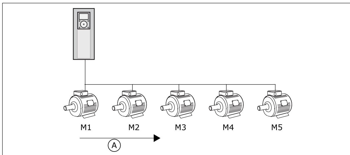
Рис. 81: Логика блокировки 1
