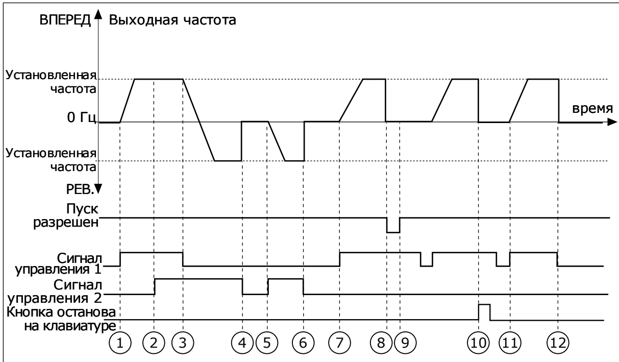
Рис. 30: Логика пуска/останова I/O A = 2
