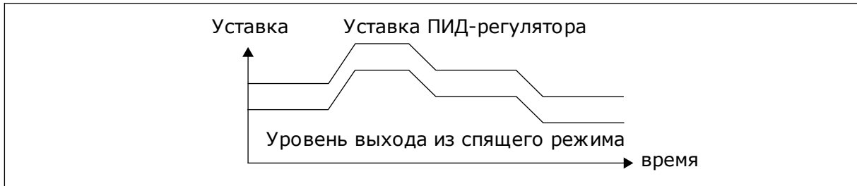
Рис. 73: Режим выхода из спящего режима: относительная уставка
