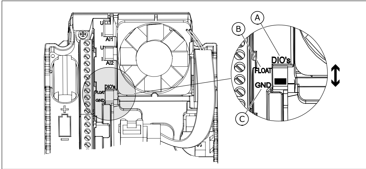
Рис. 9: DIP-переключатель
