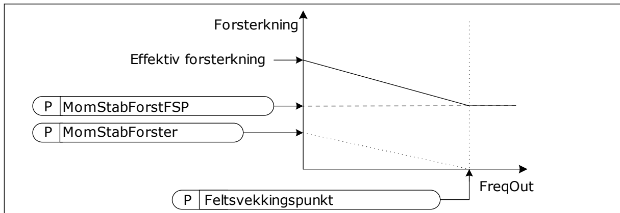
Fig. 26: Forsterkningen for momentstabilisator
