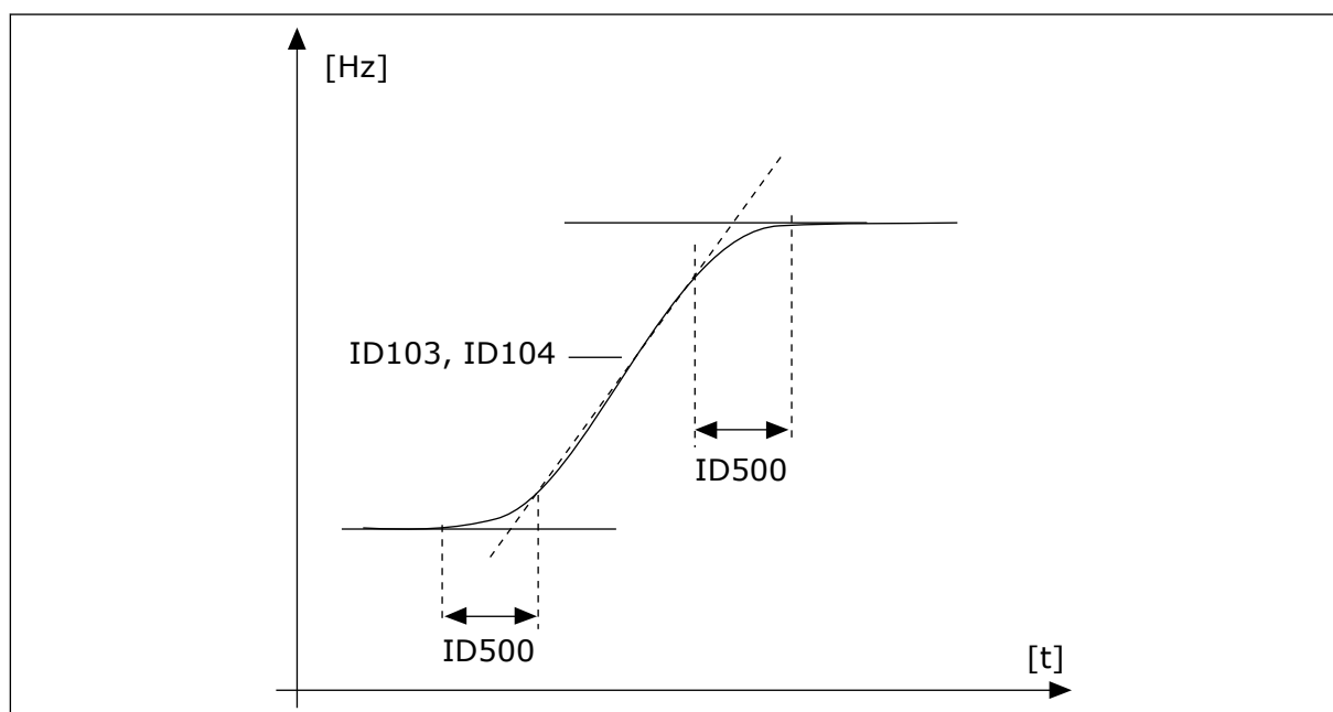
Fig. 40: Akselerasjons-/deselerasjonskurven (S-formet)
