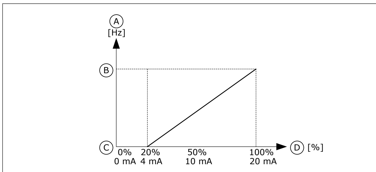
Fig. 49: Område for det analoge inngangssignalet, valg 1
