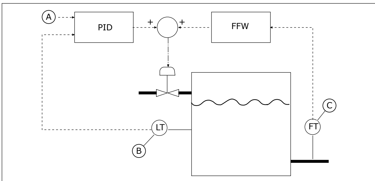
Fig. 71: Fremkoblingskontrollen
