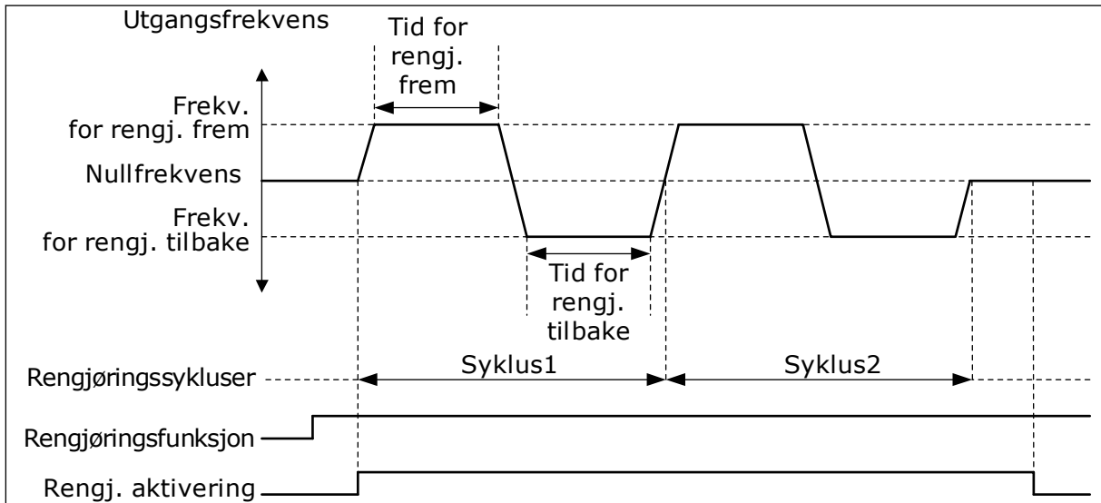
Fig. 91: Autorengjøringsfunksjonen
