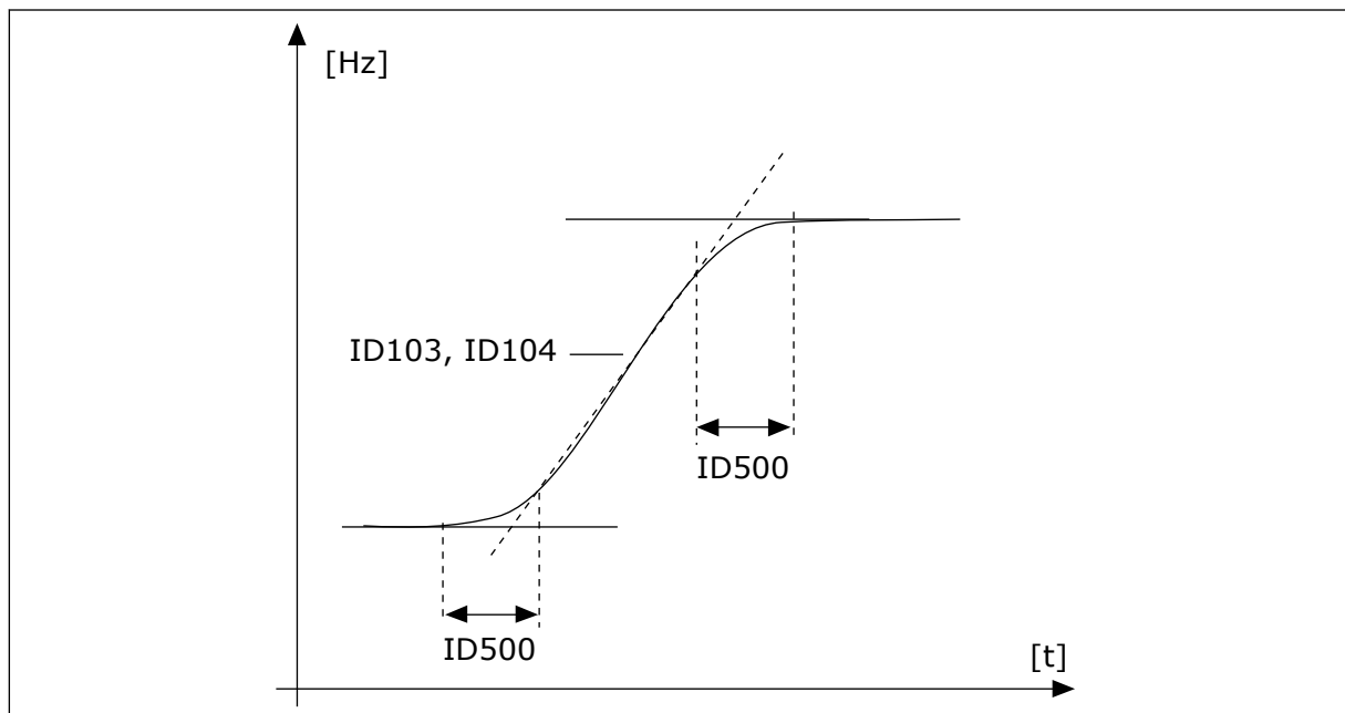
Fig. 41: Akselerasjons-/deselerasjonskurven (S-formet)
