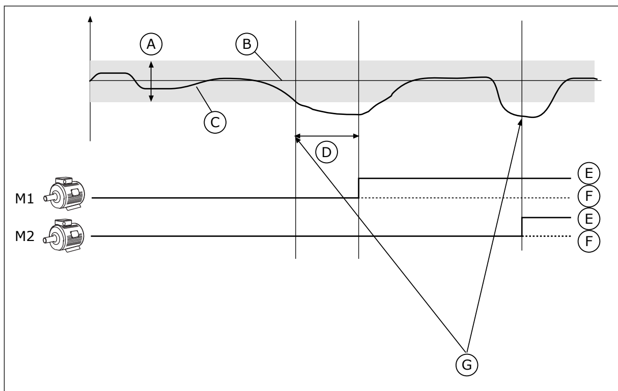
Fig. 80: Multipumpefunksjonen
