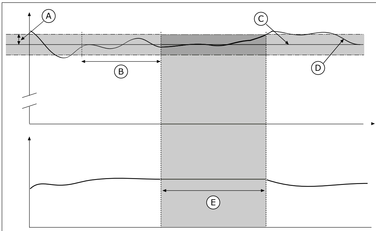
Fig. 70: Dødbåndsfunksjonen
