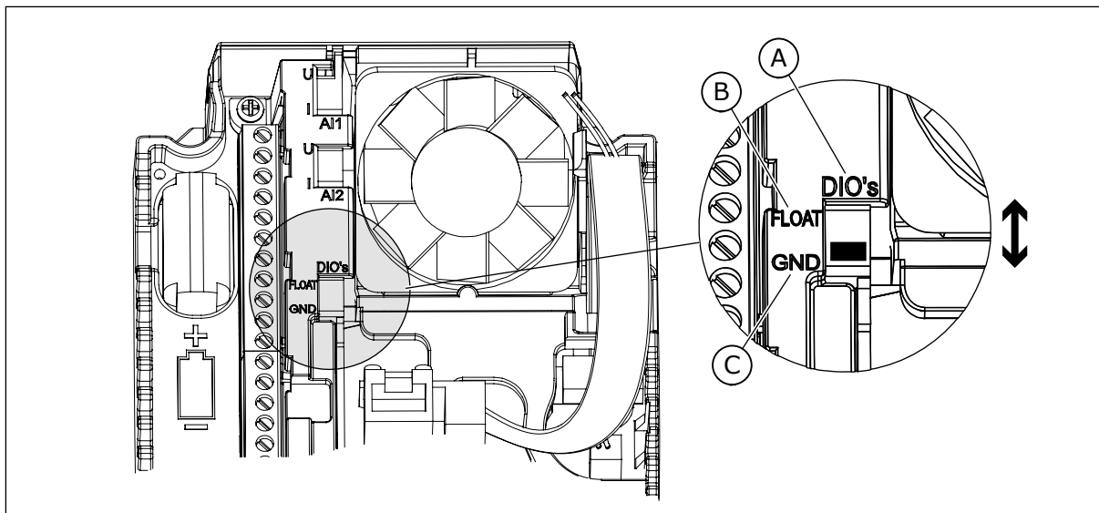
Fig. 9: DIP-bryteren
