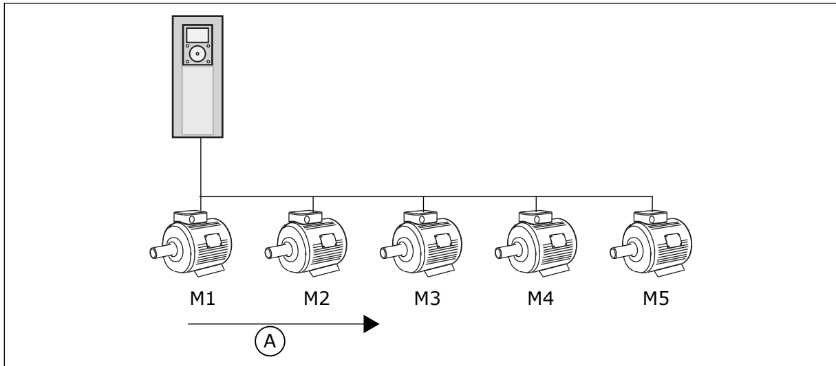
图 81: 互锁逻辑 1
