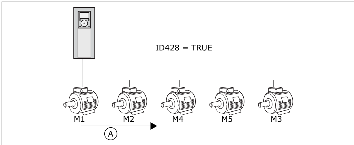
图 83: 互锁逻辑 3
