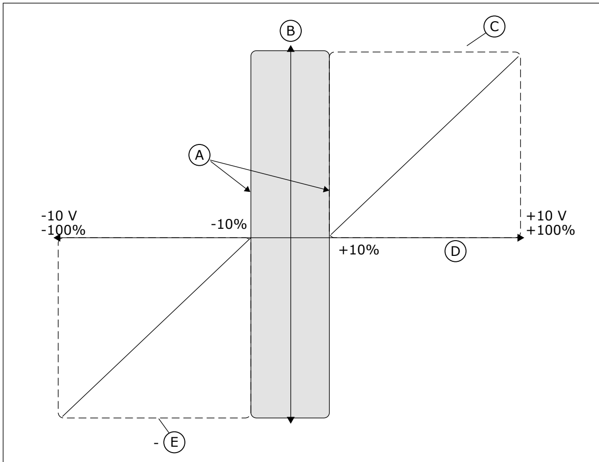
图 38: 操纵杆功能
