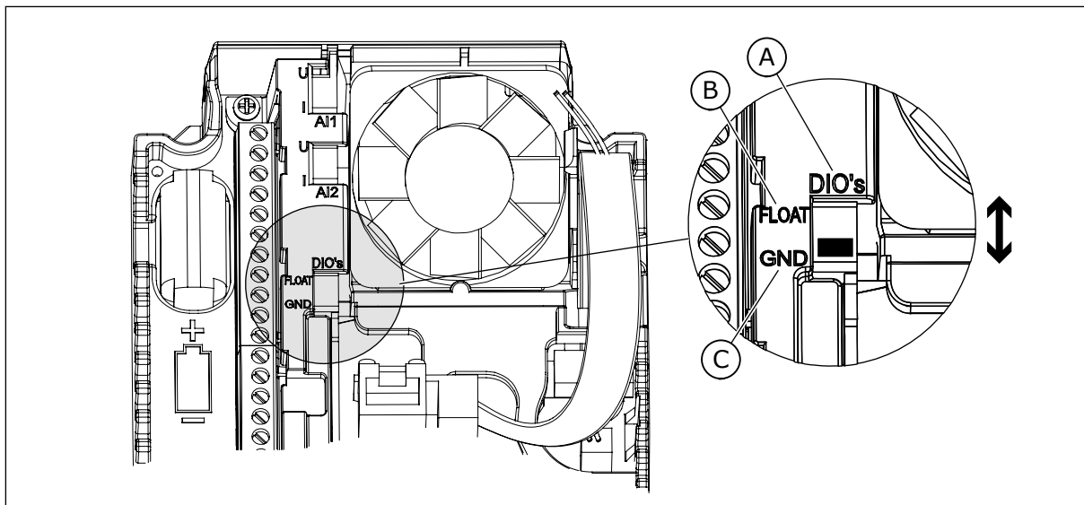
图 11: DIP 开关
