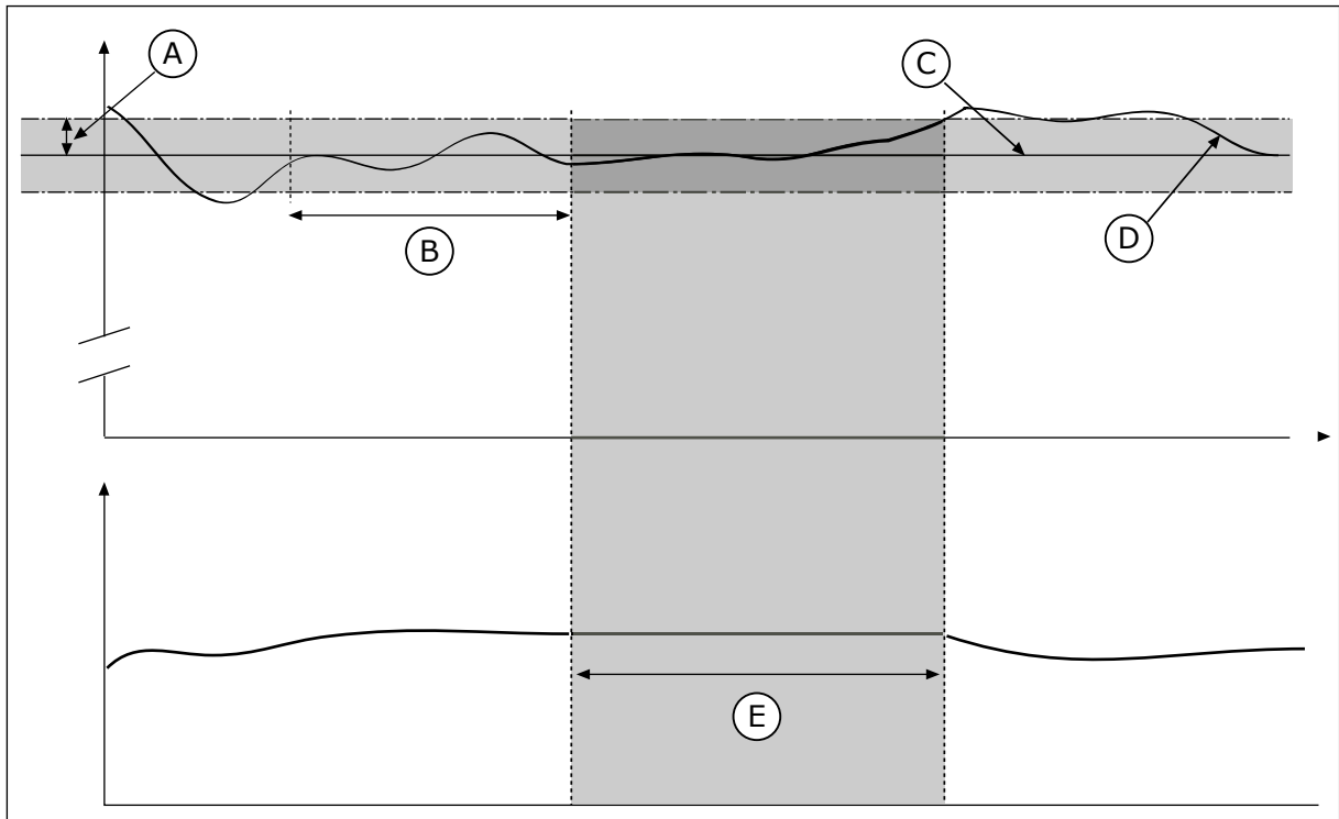
图 70: 死区功能
