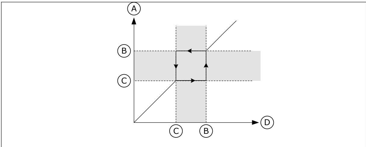
图 54: 禁止的频率
