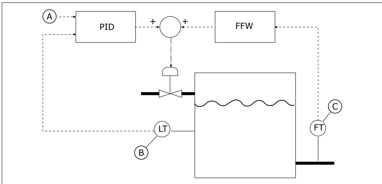
图 71: 前馈控制
