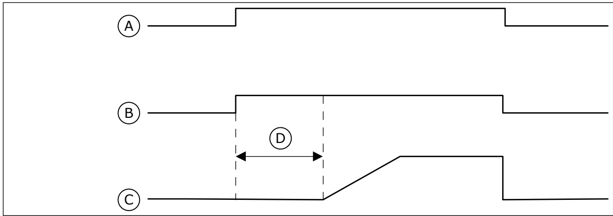
图 93: 注给泵功能
