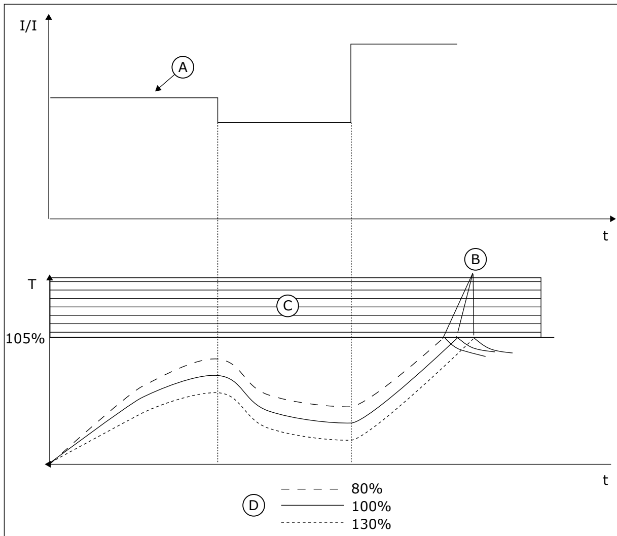
图 58: 电机温度的计算
