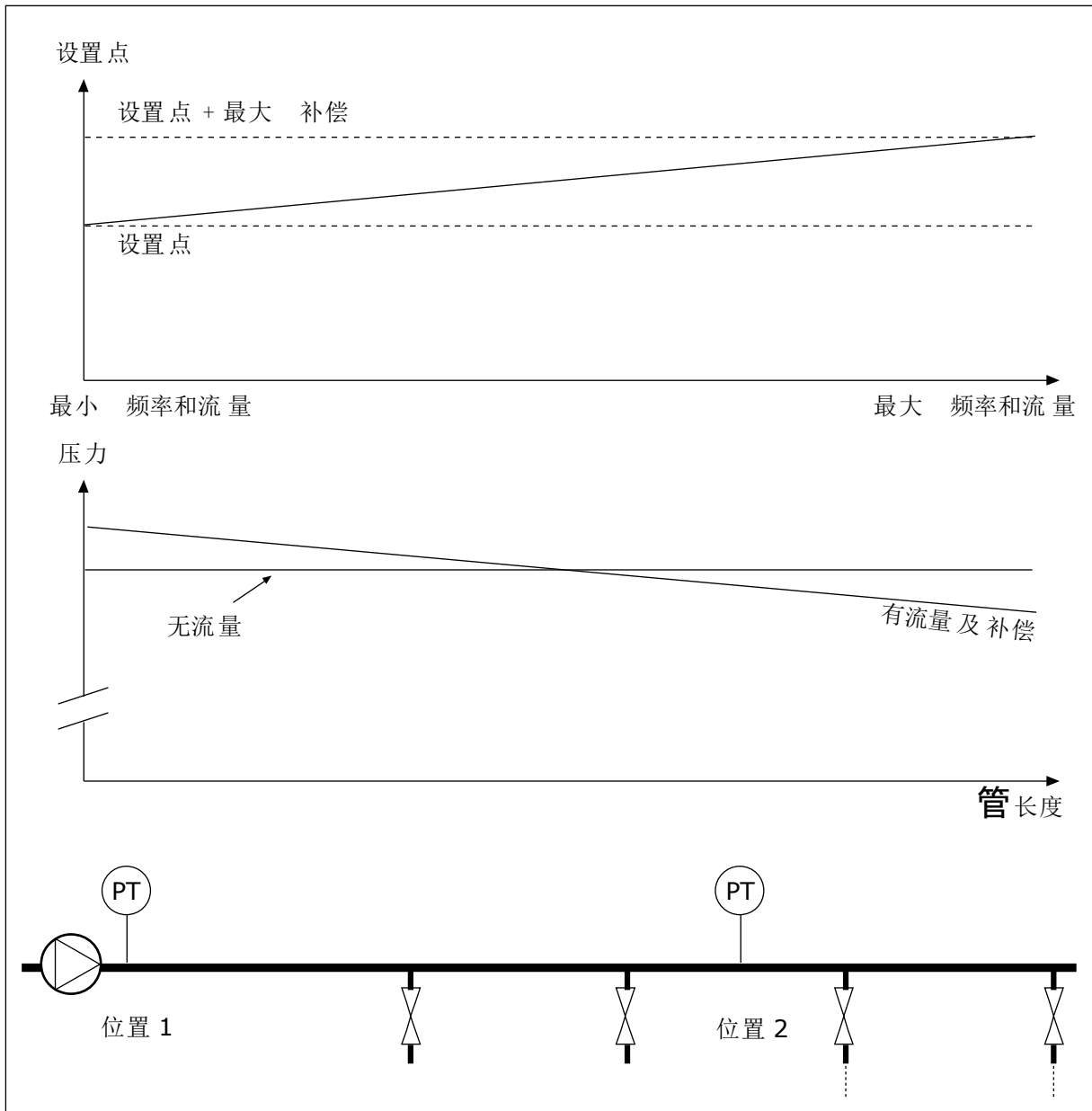
图 76: 压力损失补偿的启用设置点 1
