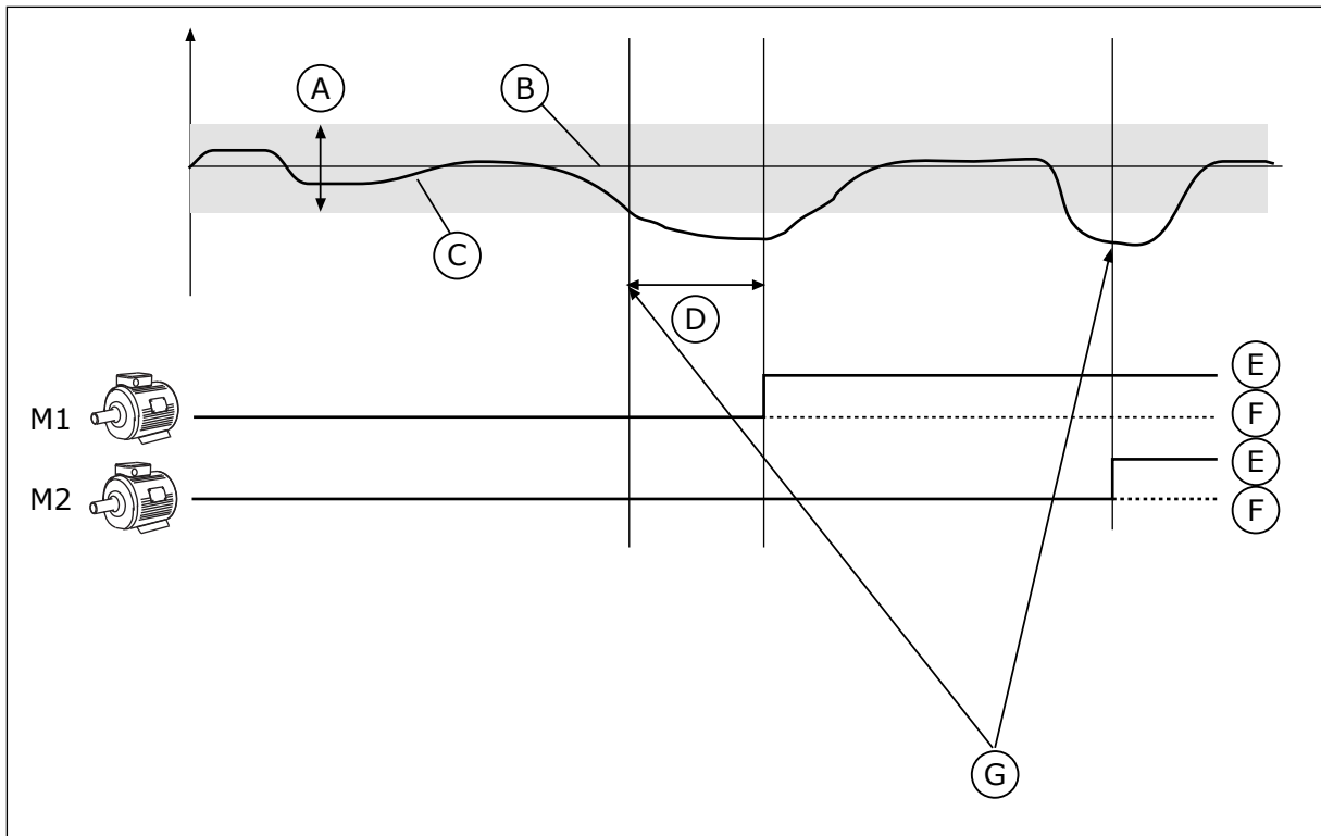
图 80: 多泵功能
