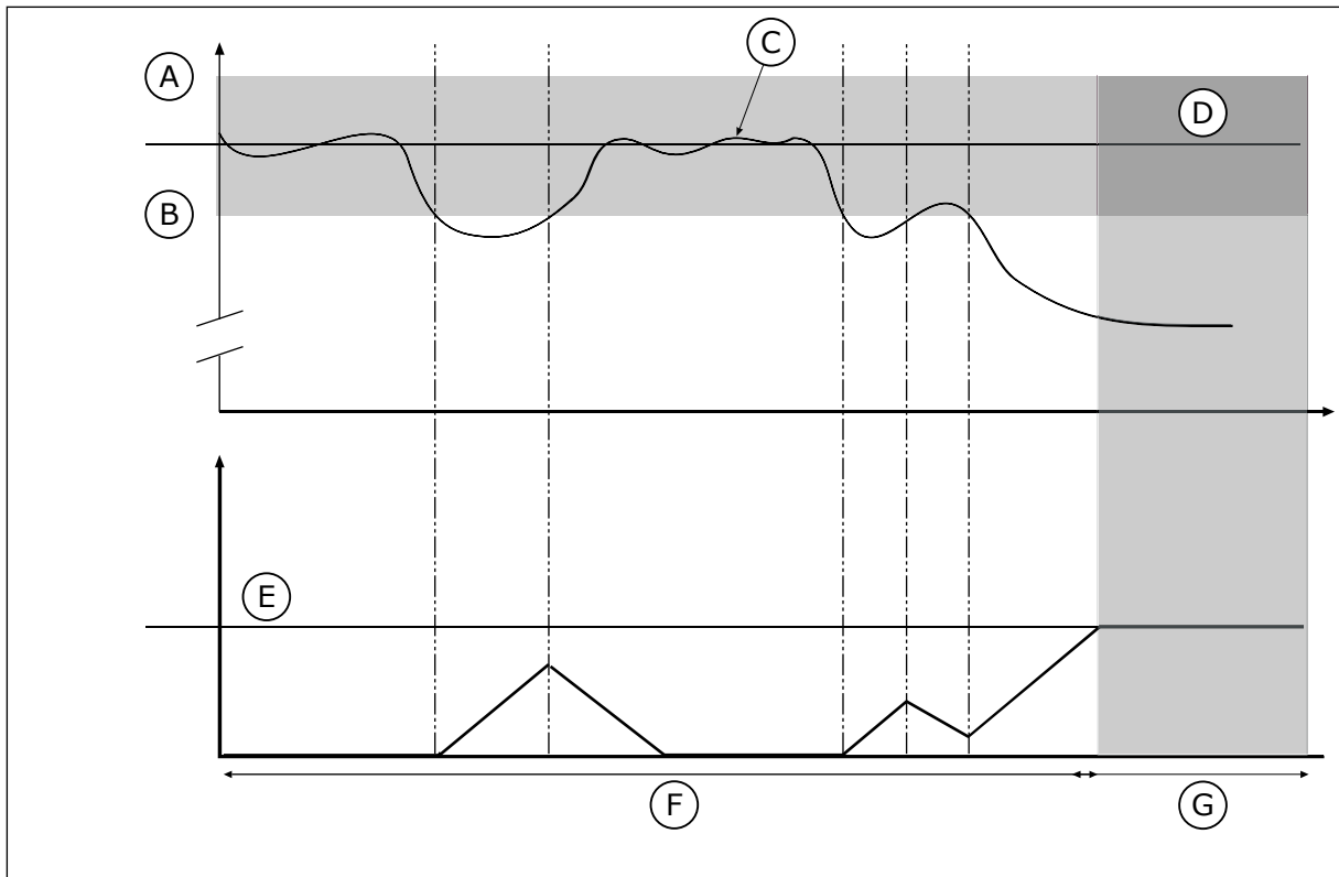
图 74: 反馈监控功能
