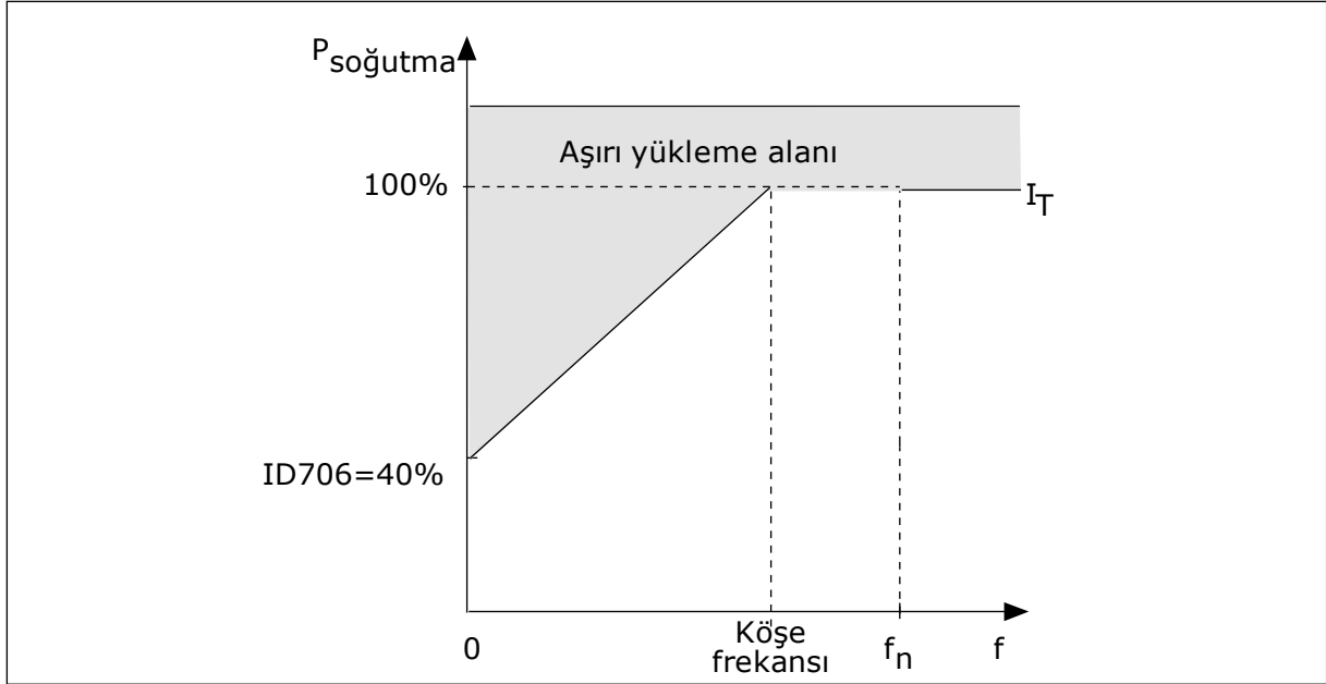
Şekil 56: Motor termal akımı I_T eğrisi
