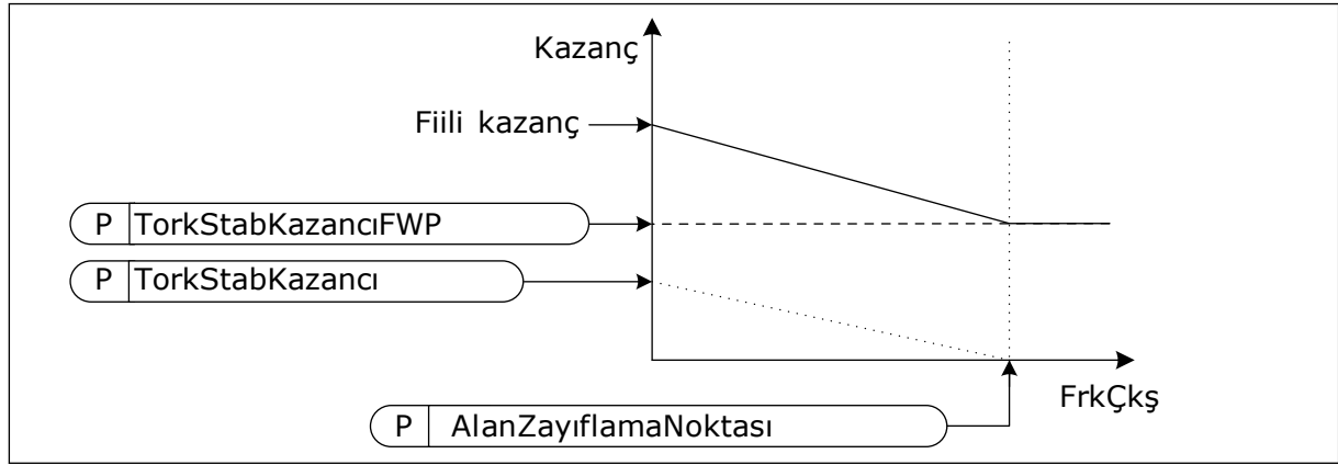
Şekil 26: Tork stabilizatörü kazancı
