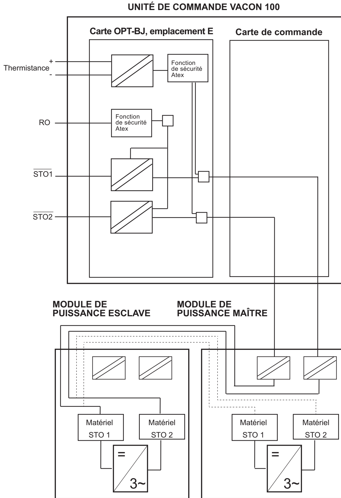
Figure 10. Principe STO avec carte OPTBJ et carte de commande Vacon 100 MR12
