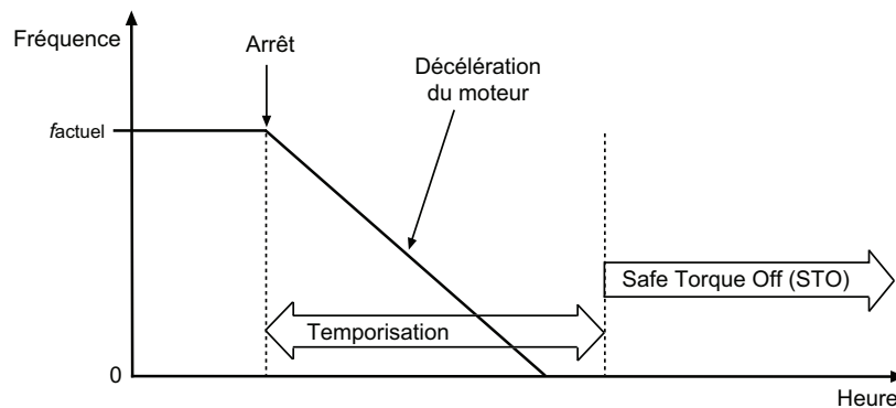
Figure 6. Principe de la fonction Safe Stop 1 (EN 61800-5-2, SS1 type c)
