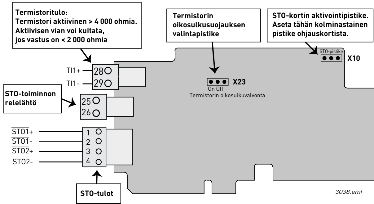
Kuva 1. OPTBJ-kortin osasijoittelu
