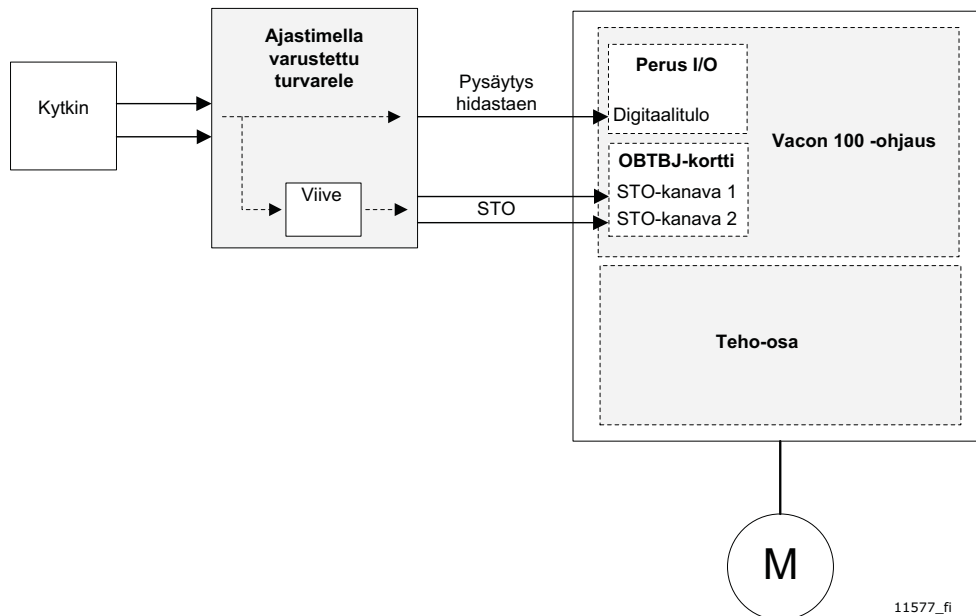
Kuva 8. SS1-toiminnon kytkentäperiaate
