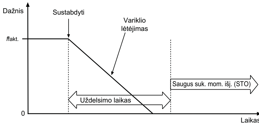
6 pav. 1 saugaus sustabdyimo principas (EN 61800-5-2, SS1 C tipas)
