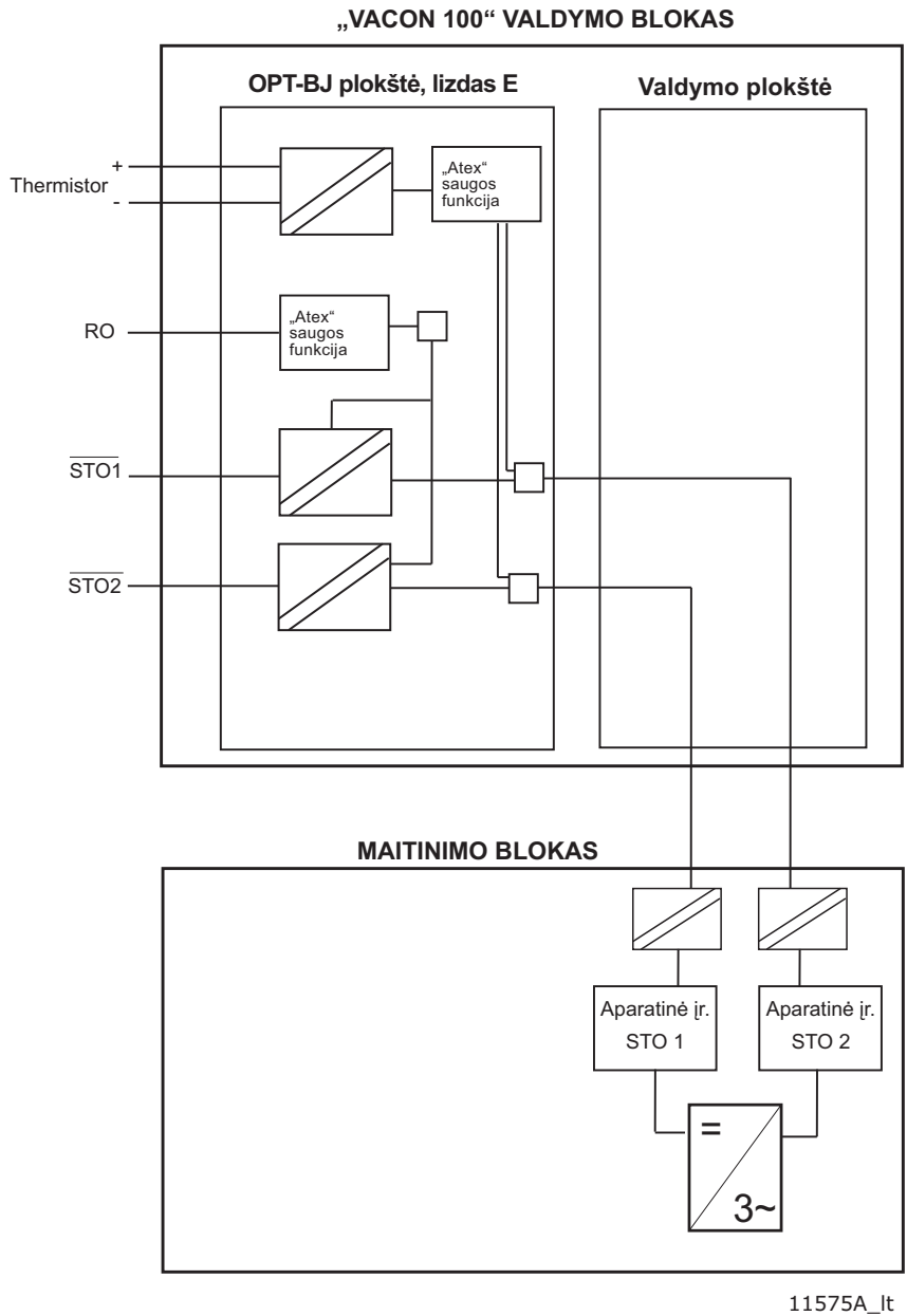
9 pav. Termistoriaus veikimo principas „Vacon 100“ dažnio keitiklyje su OPTBJ plokšte, MR4-10
