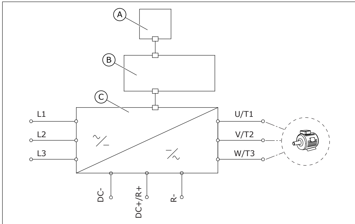
Bild 35: Principschema
