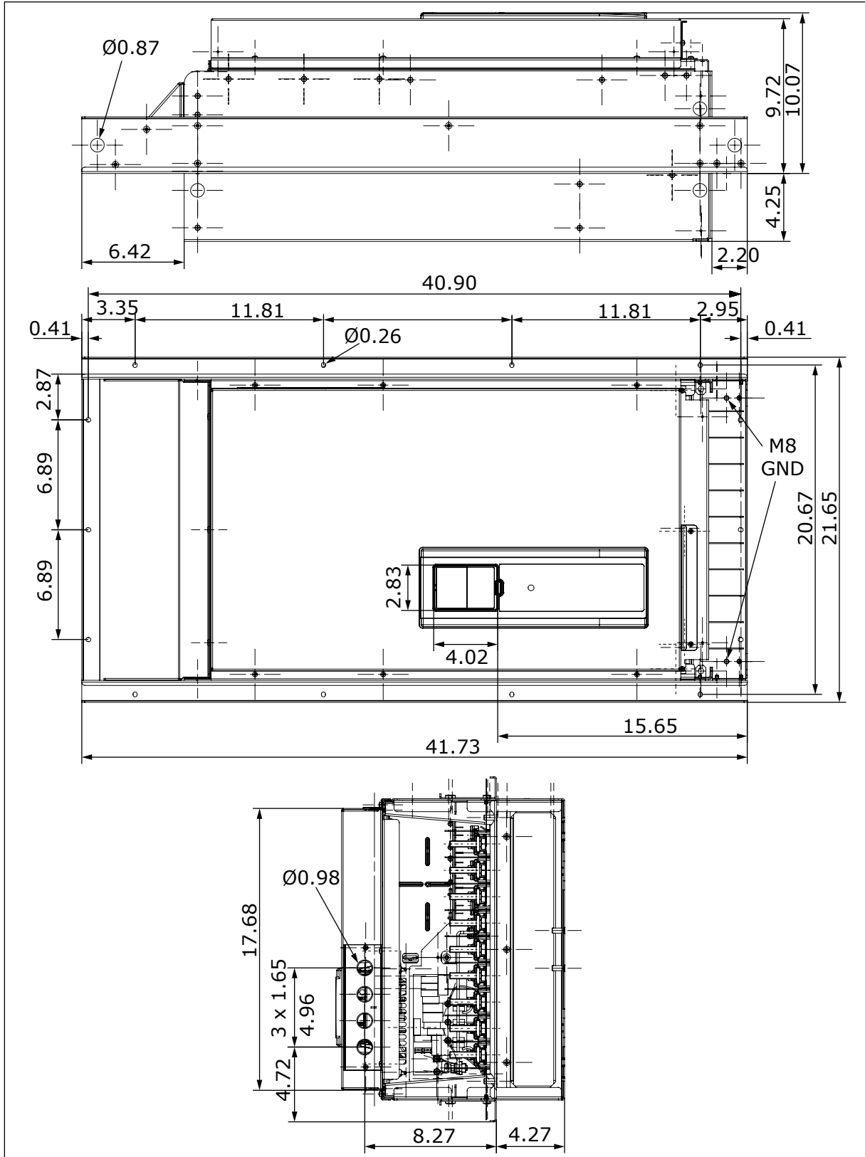
Bild 32: Frekvensomriktarens mått, flänsmontering, MR9 [tum]
