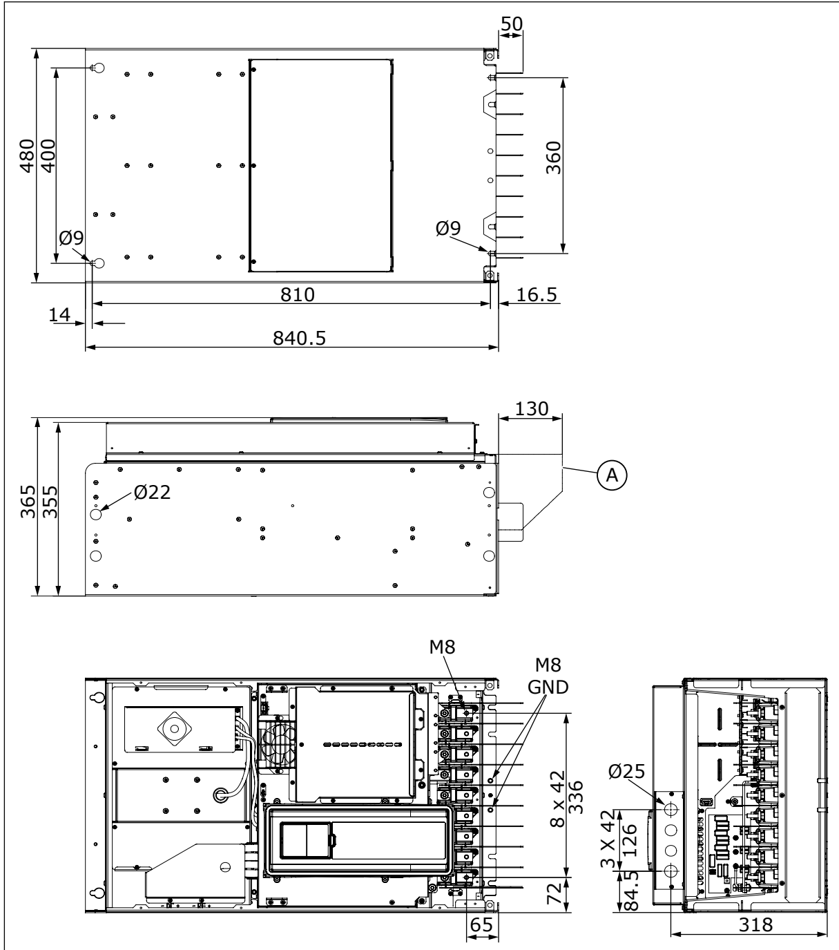
Σχ. 9: Οι διαστάσεις του ρυθμιστή στροφών AC, MR9, IP00 [mm]
