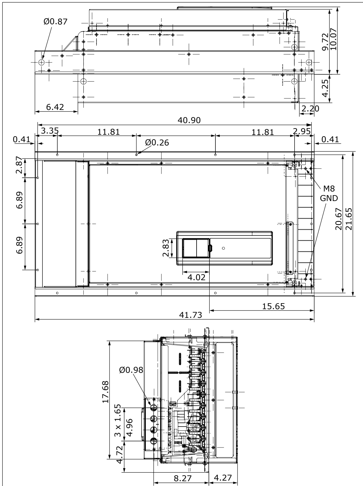
Ábra 32: A frekvenciaváltó méretei, peremes szerelés, MR9 [in]
