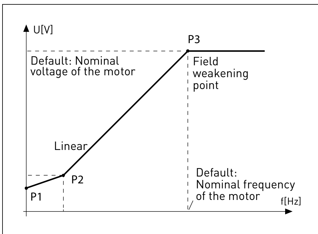
Figura 15. Curva programmabile.
