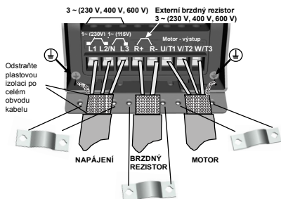
Obr. 11: Připojení napájení Vacon 20, MI2-MI3
