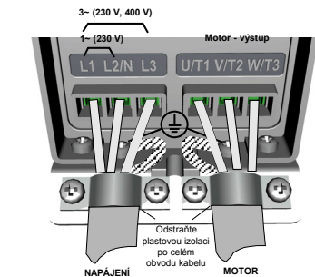
Obr. 10: Připojení napájení Vacon 20, MI1
