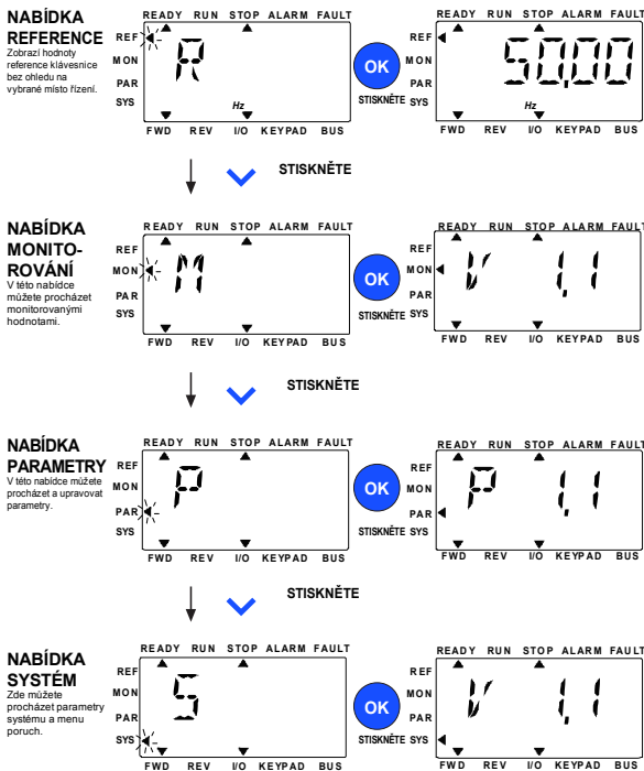
Obr. 19: Hlavní menu jednotky Vacon 20
