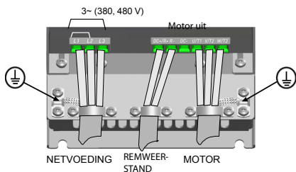
Figure 13: Netvoedingsluitingen Vacon 20, MI5
