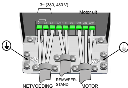
Figure 12: Netvoedingsluitingen Vacon 20, MI4
