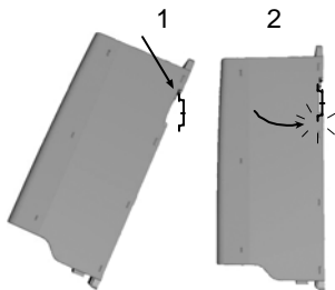
Joonis 3: DIN-rööbaskinnitus, MI1 kuni MI3
