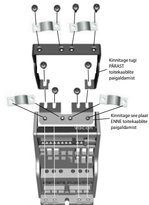
Joonis 5: PE-plaadi ja API kaablite kinnitamine, MI1 kuni MI3
