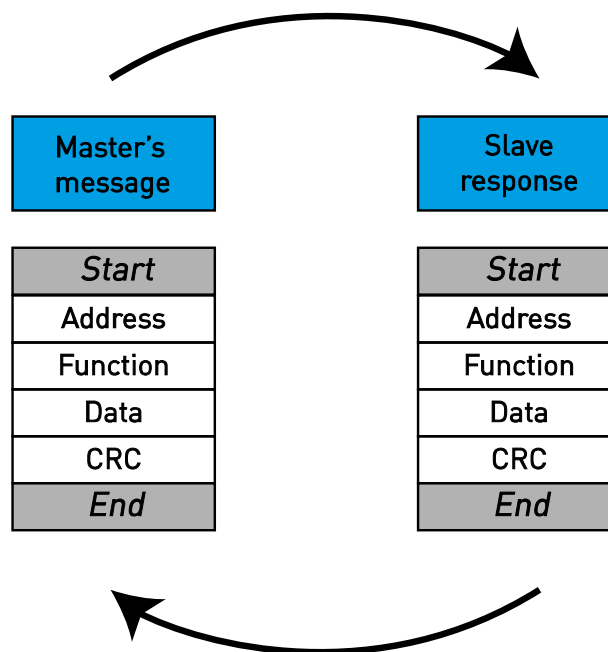
Figura 39. Struttura fondamentale del messaggio Modbus.
