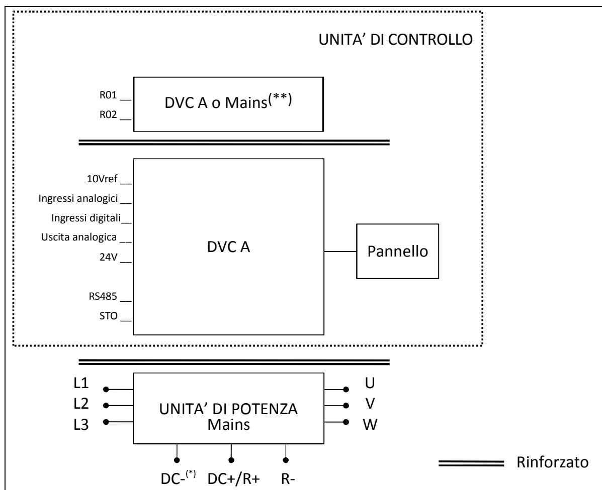
Figura 3. Sistema di isolamento (versione trifase).
