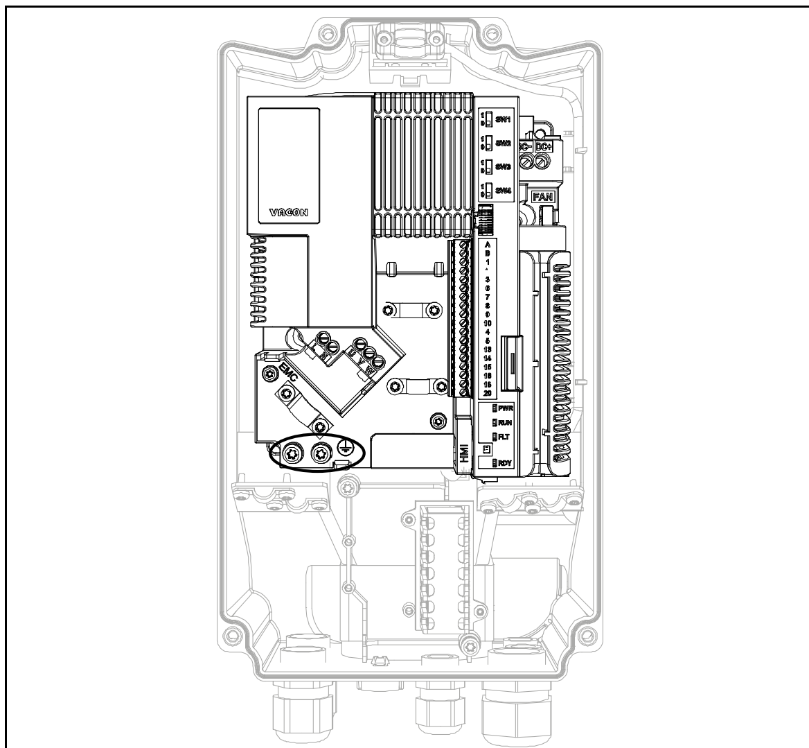
Figura 2. Collegamenti per la protezione di terra (versione monofase).
