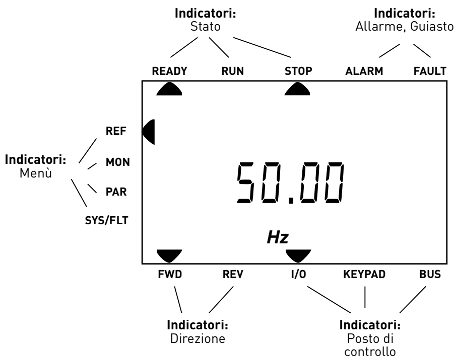
Figura 52. Display del pannello.
