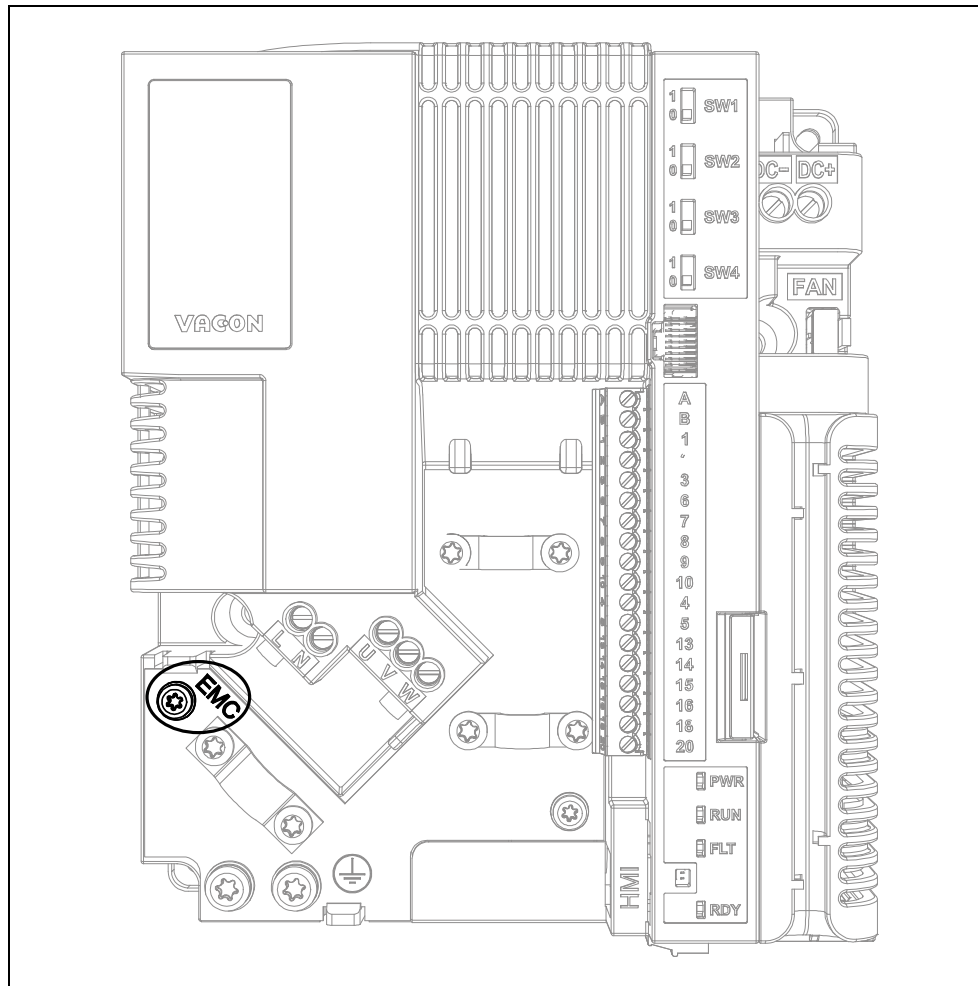
Figura 43. Cambio della classe EMC nell'unità di controllo MU2(versione monofase).
