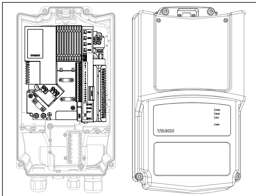
Figura 29. Coperchio anteriore dell'inverter aperto: unità di controllo MU2 (versione mono-fase).
