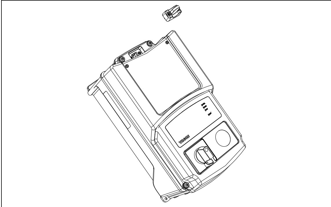
Figura 48. Rimozione del tappo HMI dall'inverter.
