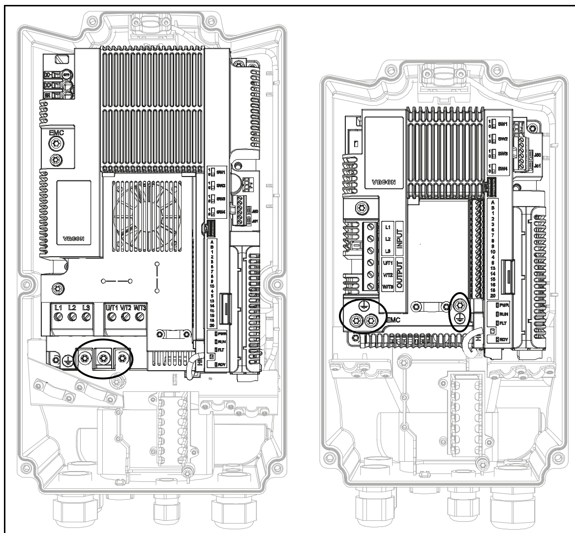
Figura 1. Collegamenti per la protezione di terra (versione trifase).
