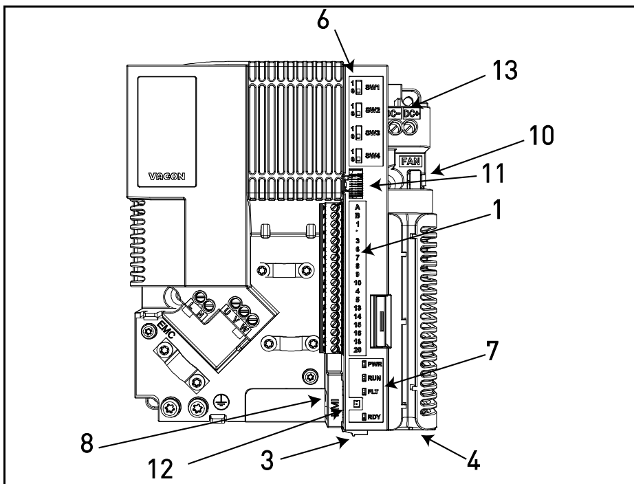
Figura 32. Posizione dei componenti nell'unità di controllo del MU2 (versione monofase).
