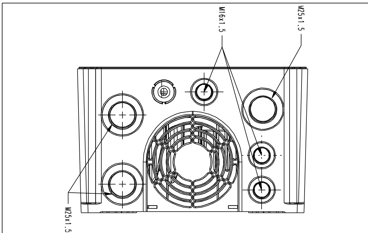
Figura 24. Ingresso cavi, MU3.
