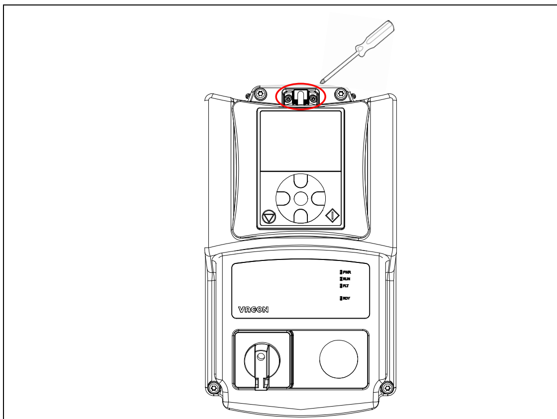
Figura 50. Stringere le due viti del cavo del pannello all'involucro dell'inverter (massima coppia di serraggio 0.5 Nm). Pannello montato sull'inverter.
