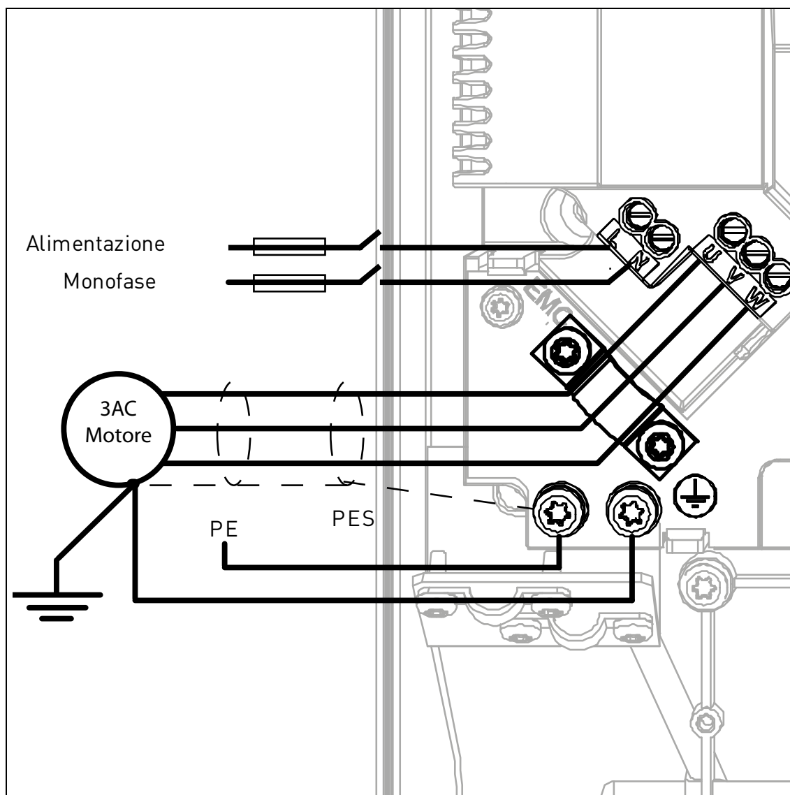
Figura 19. Collegamenti di potenza, MU2 versione monofase.
