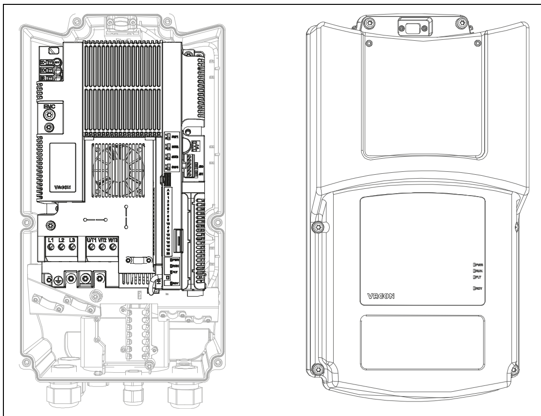
Figura 30. Coperchio anteriore dell'inverter aperto: unità di controllo MU3.
