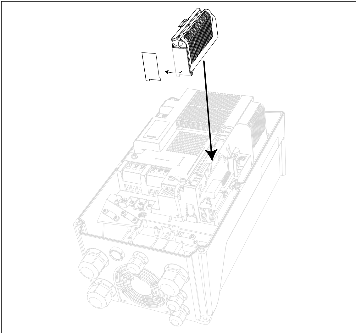
Figura 61. Montaggio del coperchio dello slot opzionale: rimuovere l'apertura in plastica per i morsetti della scheda opzionale.
