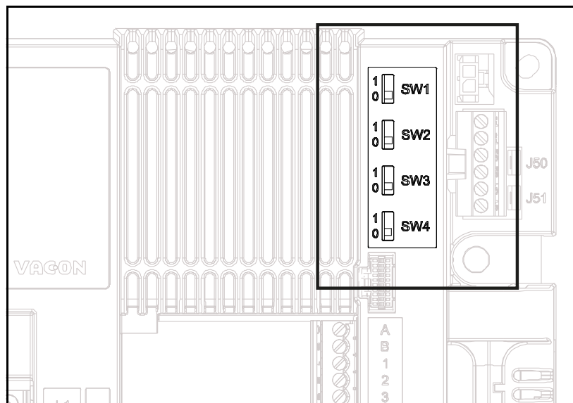
Figura 38. Dip switch sull'unità di controllo.
