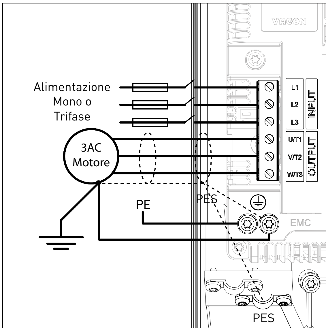
Figura 18. Collegamenti di potenza, MU2 versione trifase.
