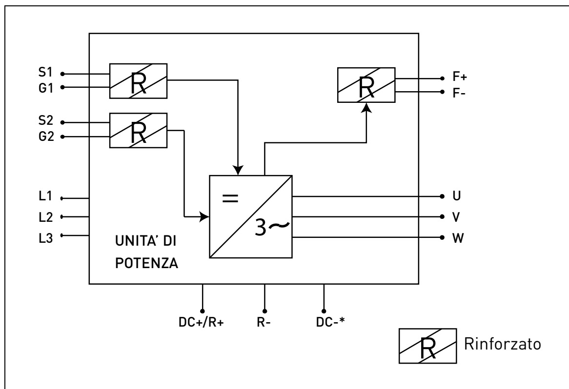
Figura 70. Schema funzionale del STO. (*) Solo per MU3.
