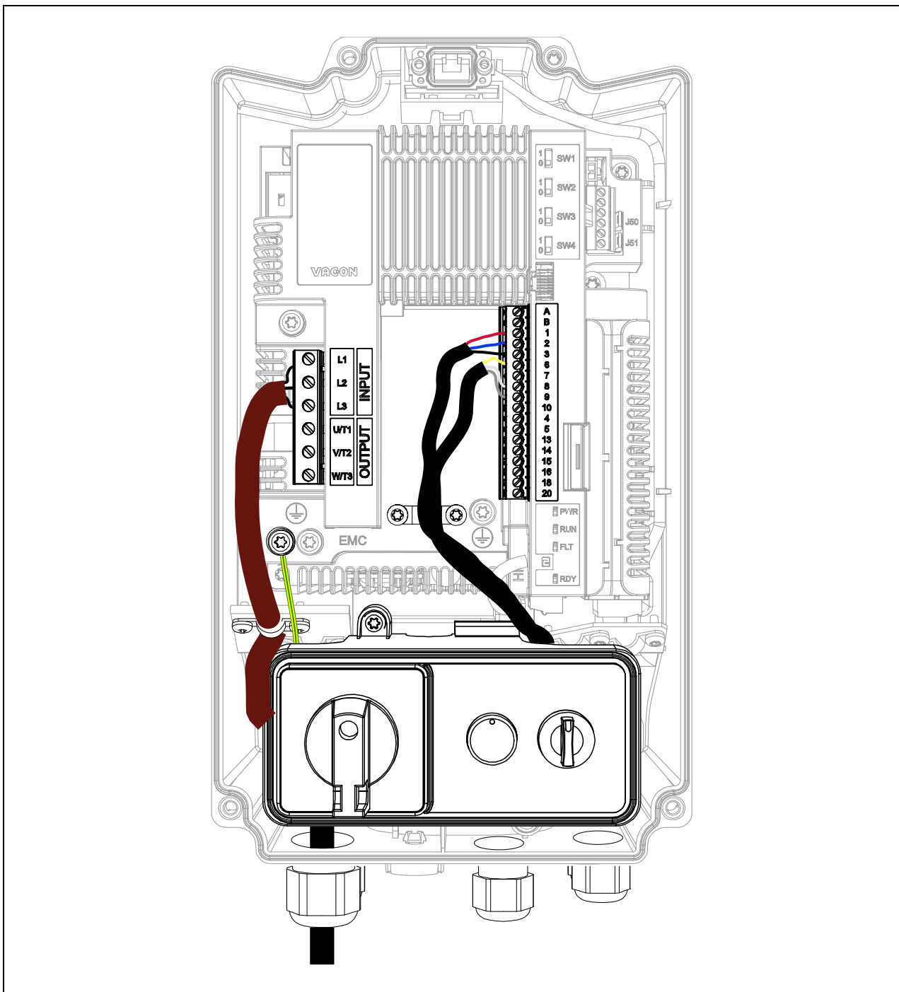
Figura 68. Pannello operatore collegato (esempio MU2 versione trifase).
