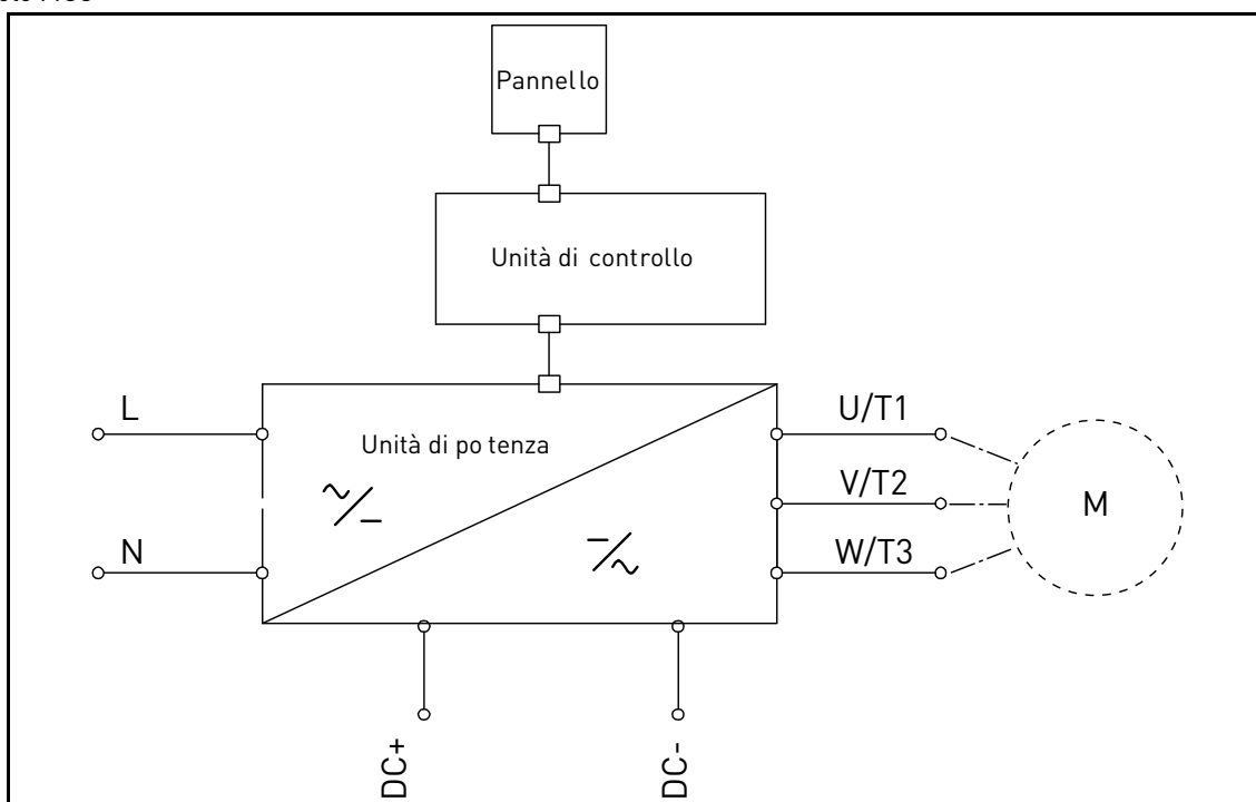
Figura 16. Schema dei collegamenti (versione monofase).
