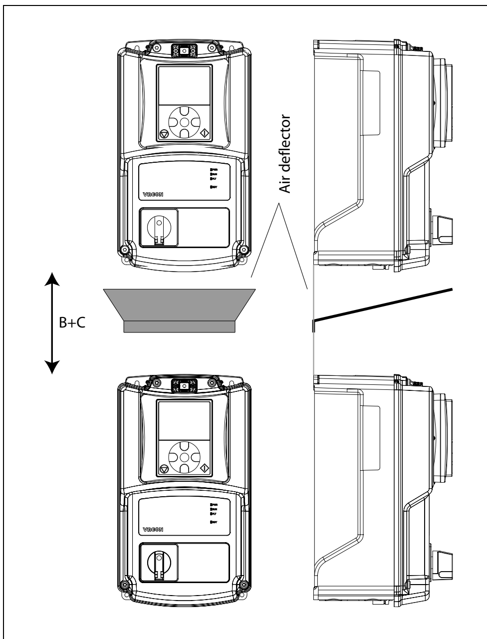
Figura 14. Spazio d'installazione necessario in caso di montaggio sovrapposto degli inverter.
