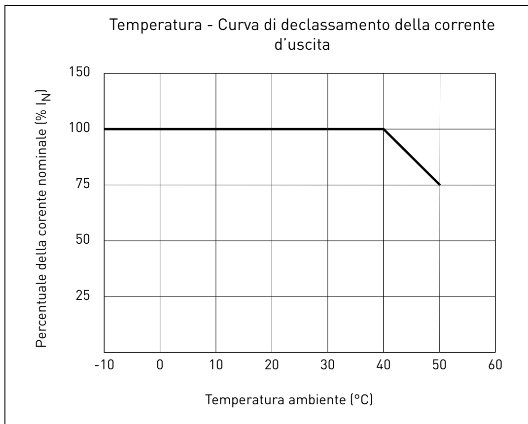
Figura 5. Curva di declassamento corrente di uscita/temperatura.
