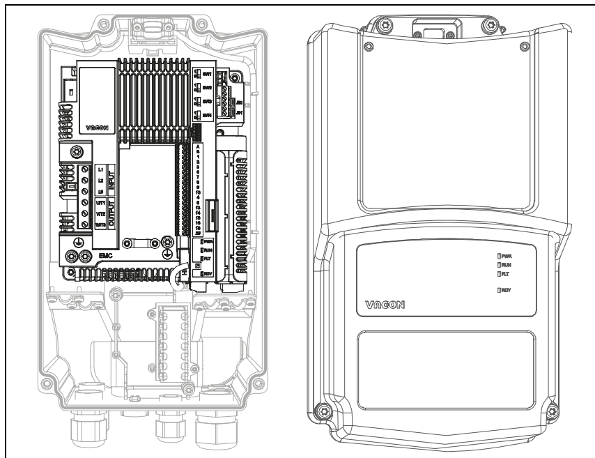
Figura 28. Coperchio anteriore dell'inverter aperto: unità di controllo MU2 (versione trifase).
