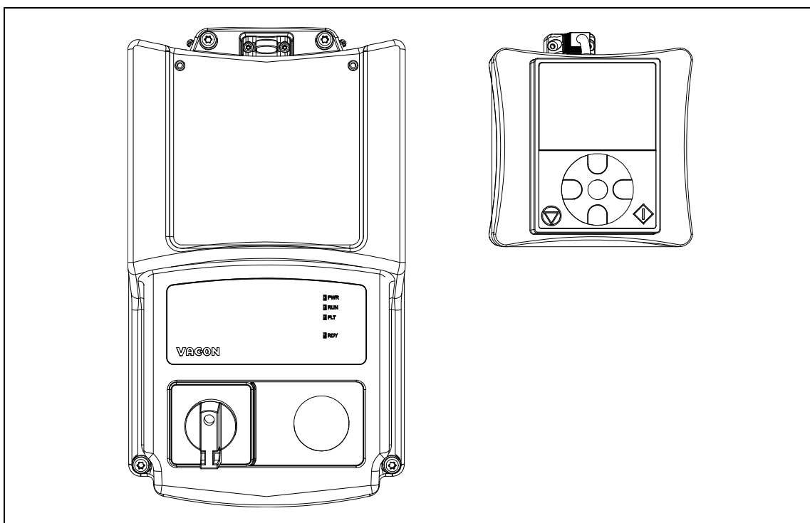
Figura 47. L'inverter e l'opzione kit pannello. L'opzione kit pannello include: pannello e cavo.
