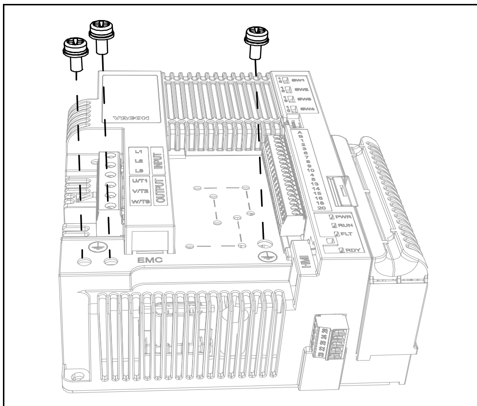
Figura 41. Cambio della classe EMC nell'unità di controllo MU2.
