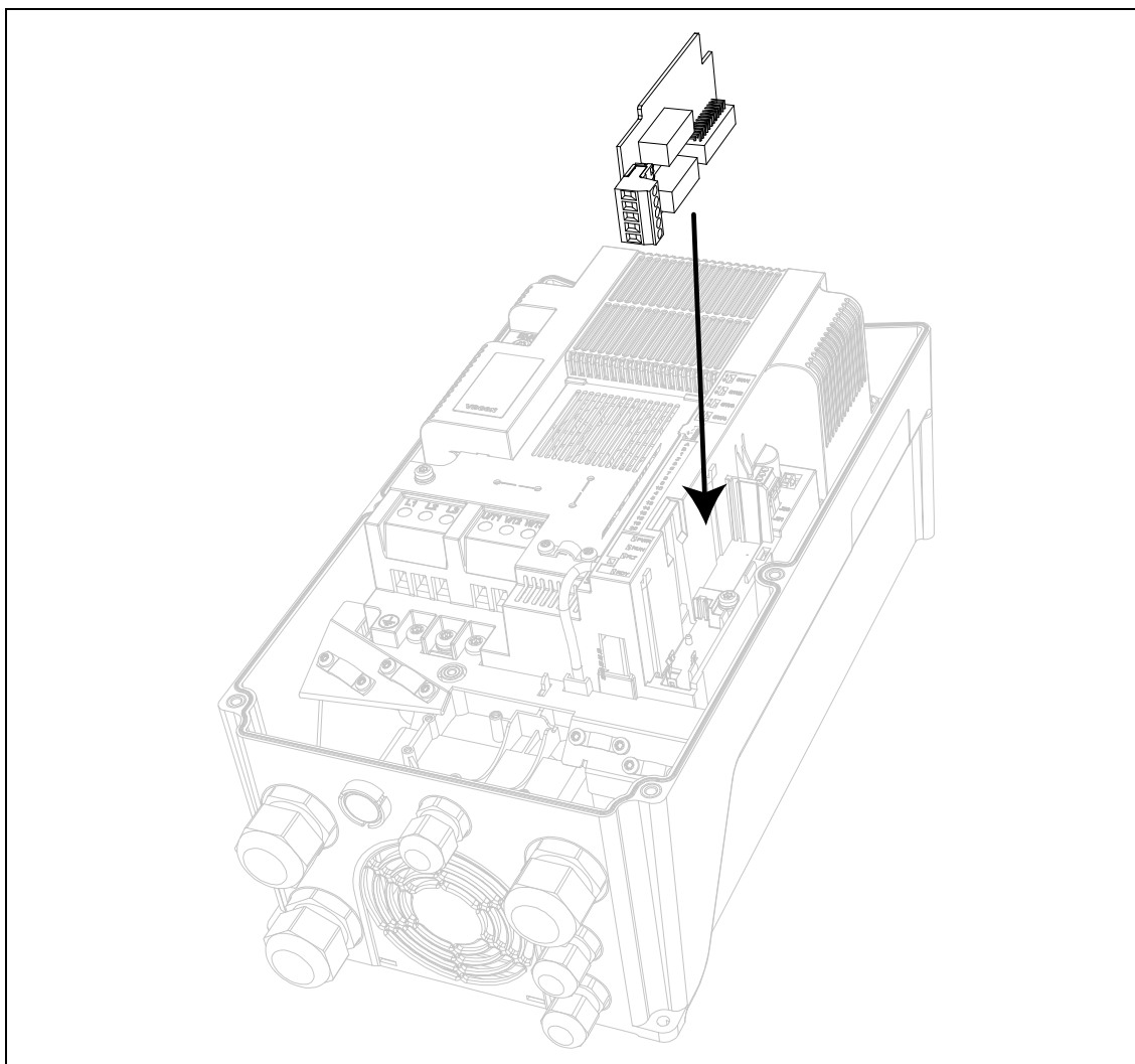
Figura 60. Installazione della scheda opzionale.
