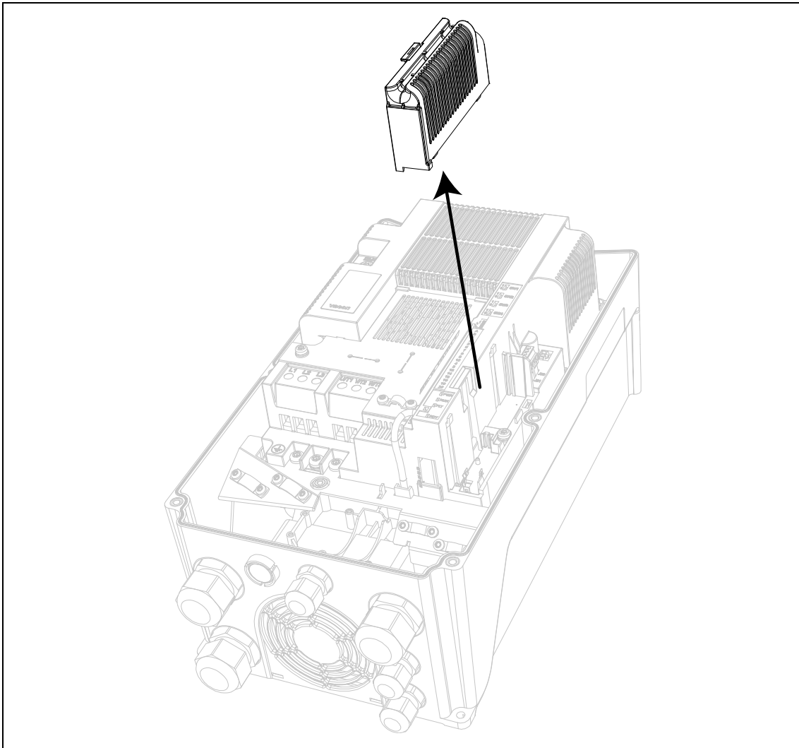
Figura 59. Rimozione del coperchio dello slot opzionale.
