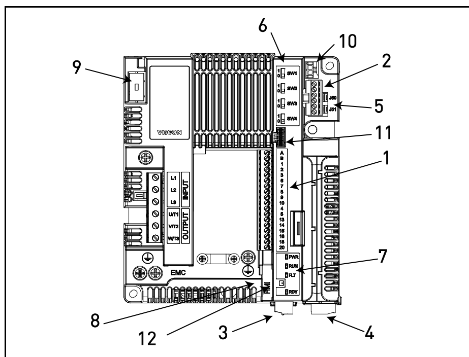
Figura 31. Posizione dei componenti nell'unità di controllo del MU2 (versione trifase).
