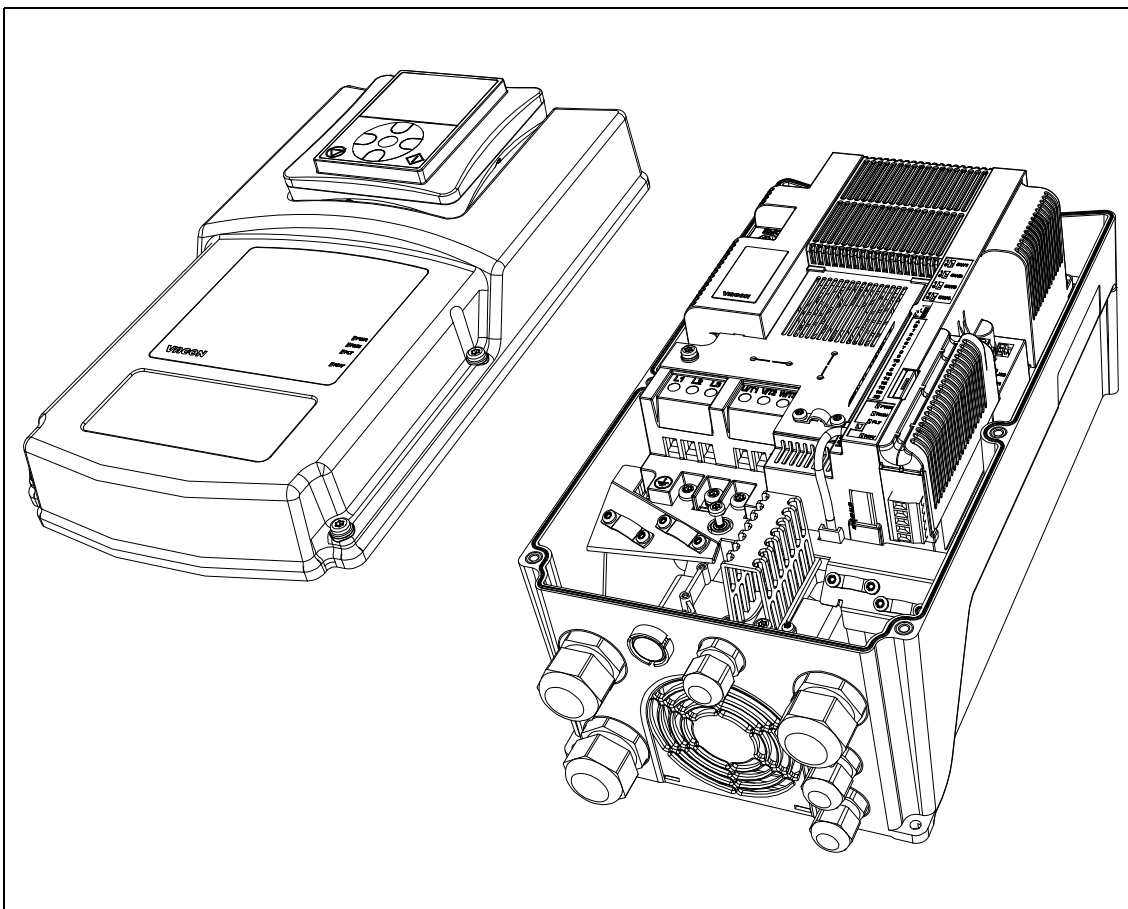
Figura 58. Apertura del coperchio principale, esempio di MU3.
