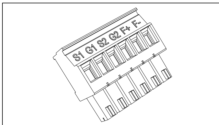
Figura 9. Connettore STO.
