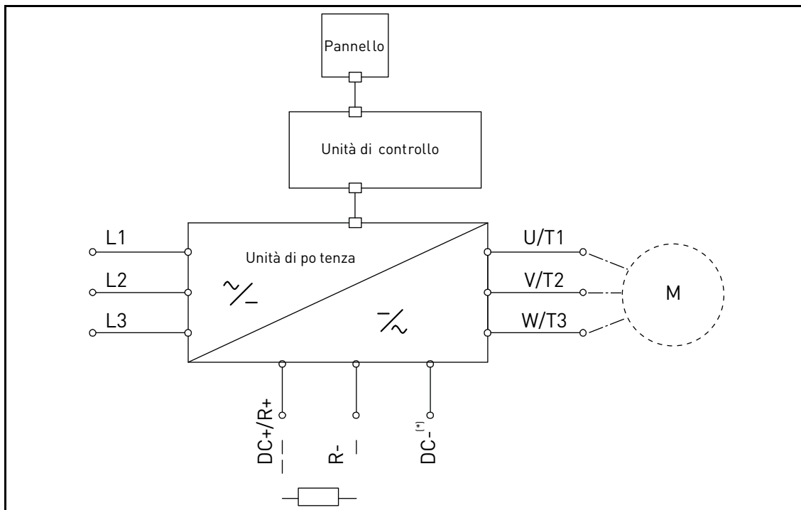
Figura 15. Schema dei collegamenti (versione trifase).
