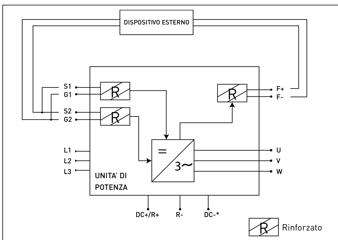
Figura 74. Esempio STO con controllo automatico del feedback e ingressi STO collegati in parallelo. (*) Solo per MU3.
