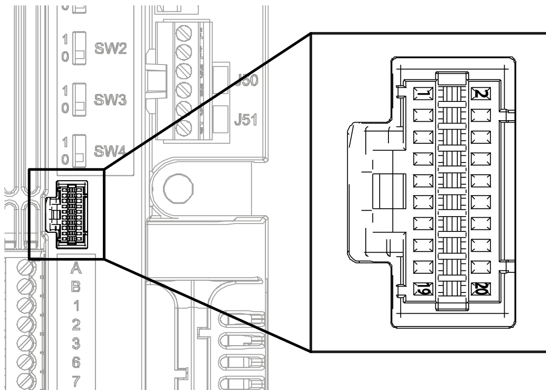
Figura 35. Connettore eco remoto I/O montato sulla scheda di controllo.
