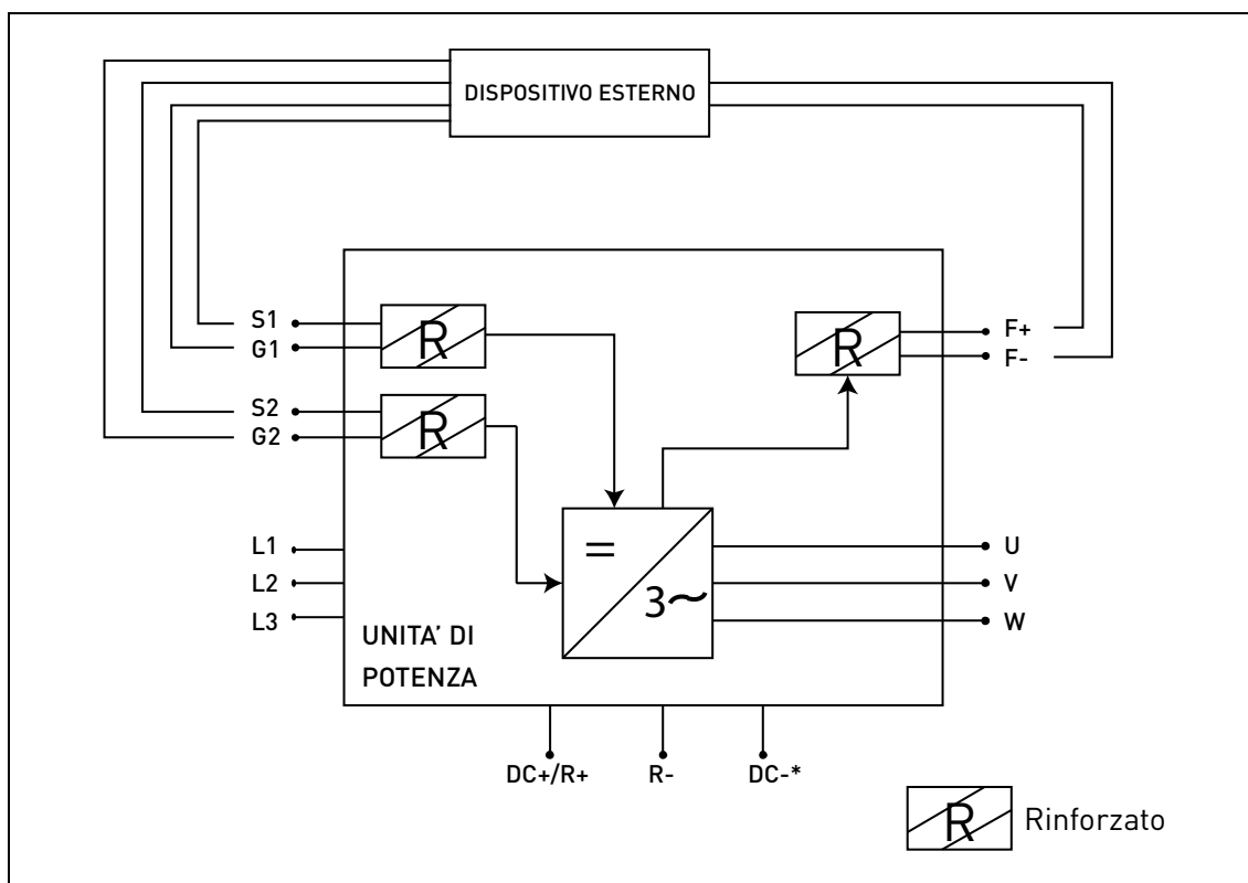
Figura 73. Esempio STO con controllo automatico del feedback ed entrambi gli ingressi STO utilizzati. (*) Solo per MU3.
