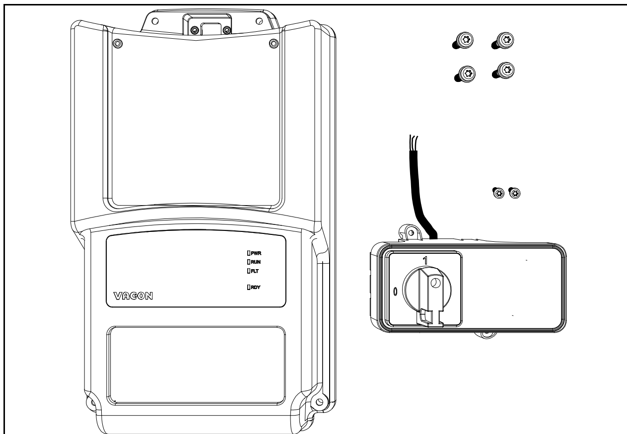
Figura 62. Il kit di ricambio opzionale dell'interruttore di rete (esempio MU2).
