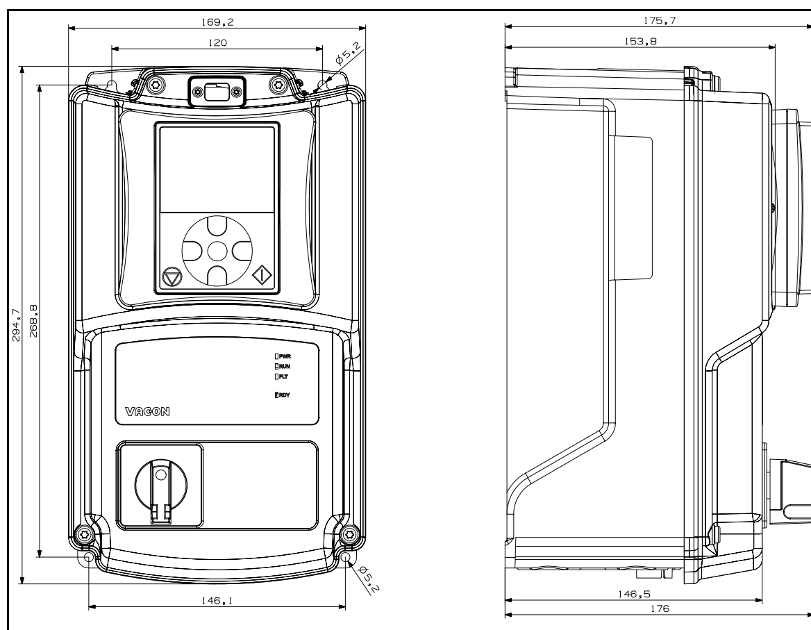
Figura 11. VACON® 20 X, MU2.
