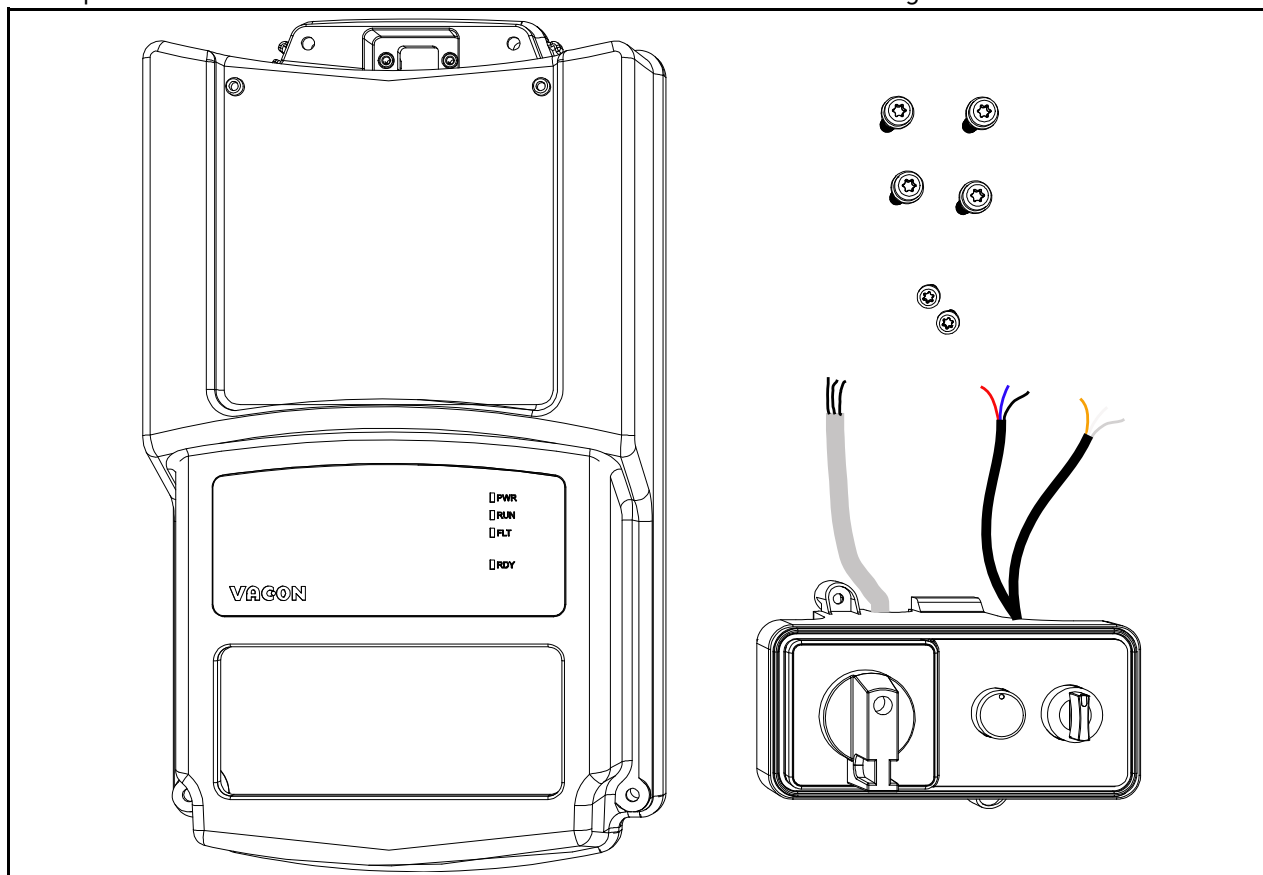
Figura 66. Il kit di ricambio opzionale del pannello operatore (esempio MU2).
