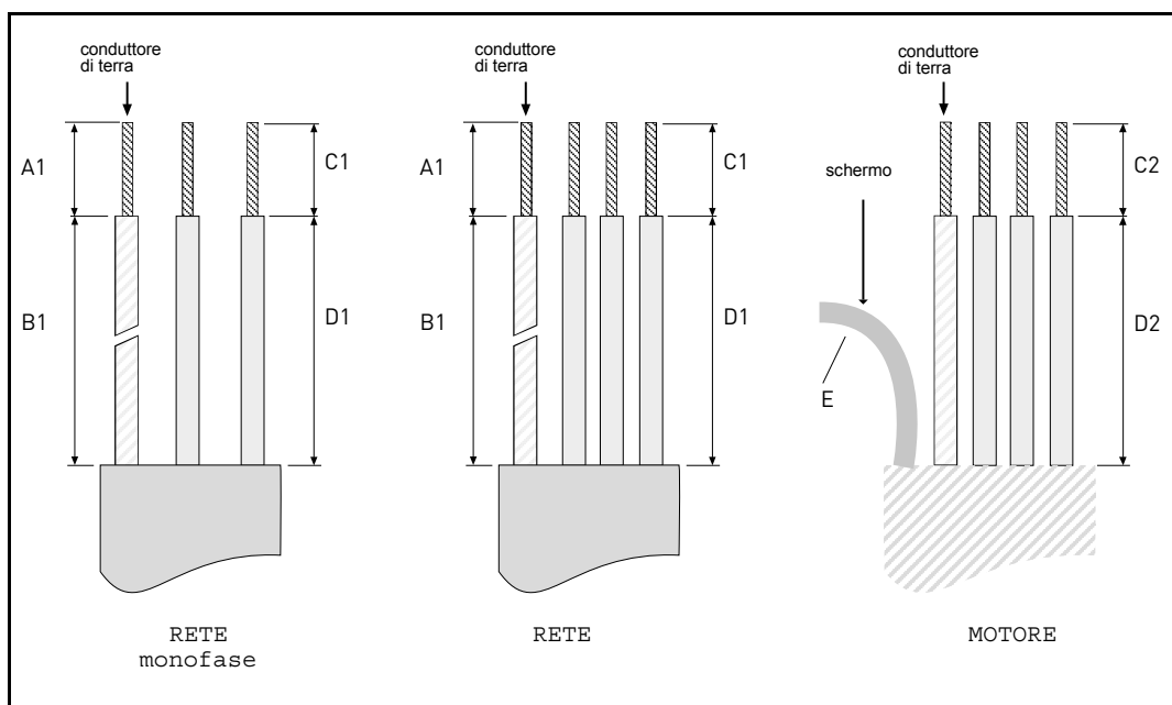
Figura 21. Spelatura dei cavi.
