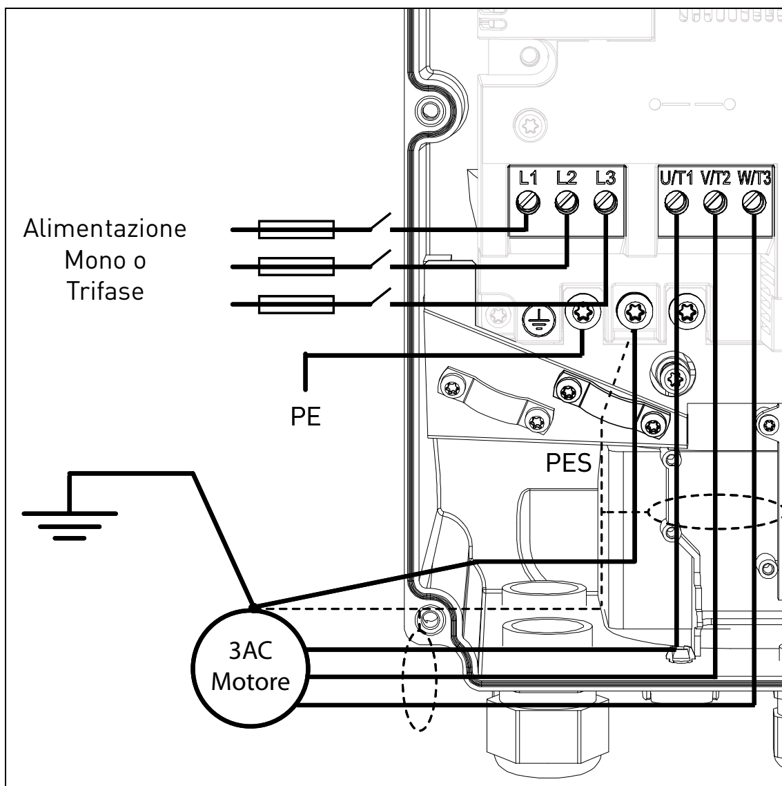
Figura 20. Collegamenti di potenza, MU3.
