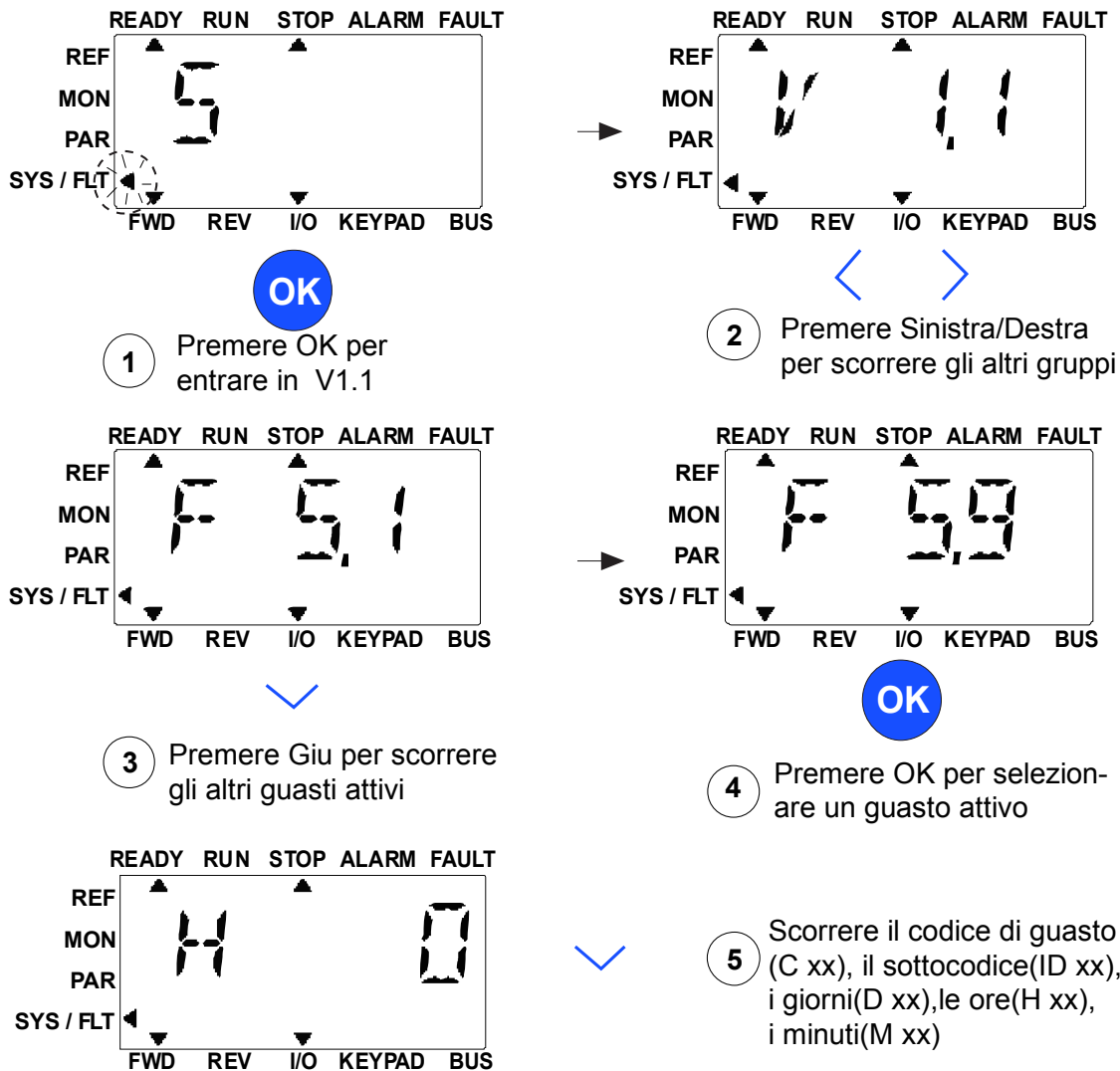
Figura 57. Menu Sistema e Guasti.
