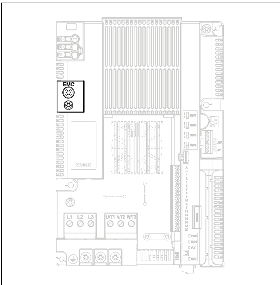
Figura 44. Cambio della classe EMC nell'unità di controllo MU3.
