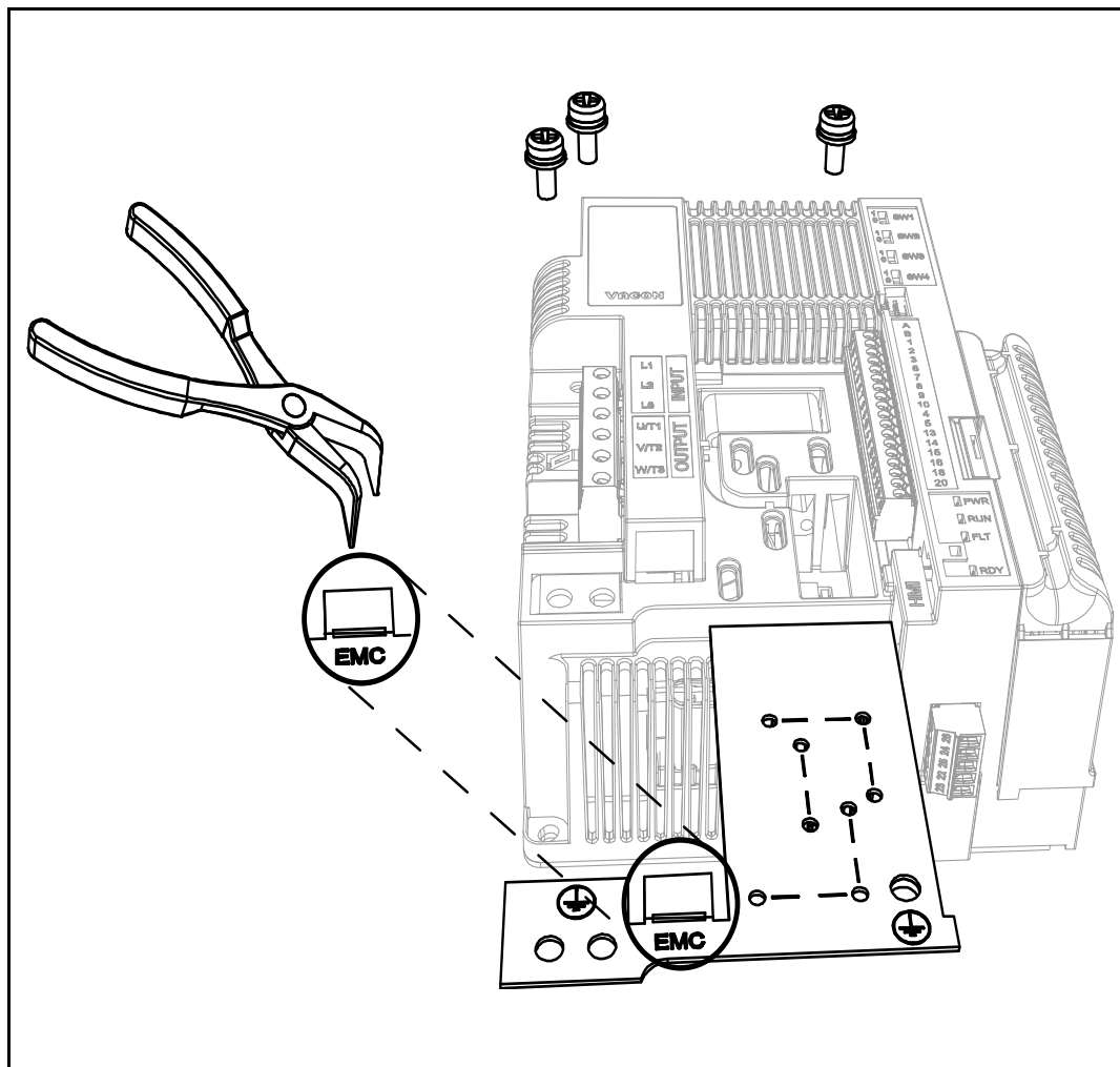
Figura 42. Cambio della classe EMC nell'unità di controllo MU2.
