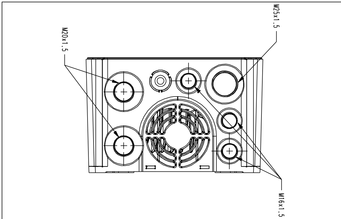
Figura 23. Ingresso cavi, MU2.
