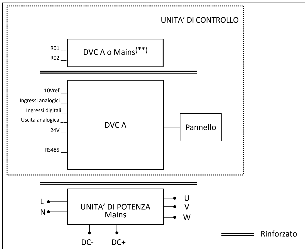
Figura 4. Sistema di isolamento (versione monofase).
