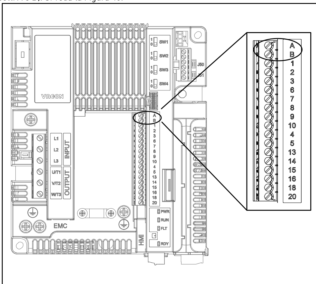
Figura 40. Posizione dei morsetti RS485 sul connettore dei morsetti della scheda I/O standard (esempio: unità di controllo MU2).
