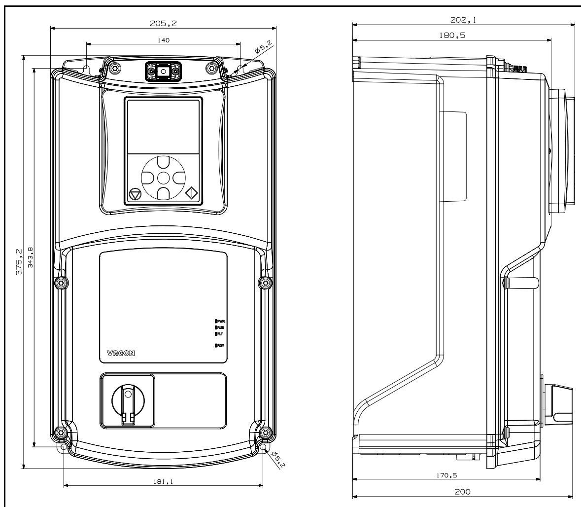
Figura 12. VACON® 20 X, MU3.
