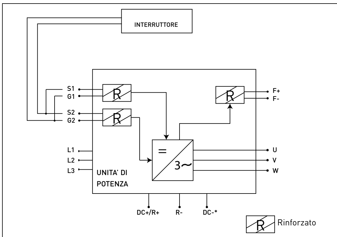
Figura 75. Esempio STO senza controllo automatico del feedback e ingressi STO collegati in parallelo. (*) Solo per MU3.
