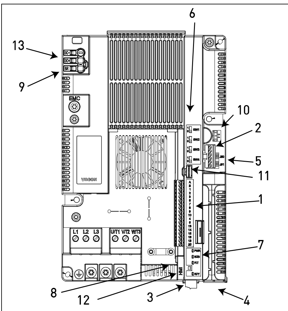
Figura 33. Posizione dei componenti nell'unità di controllo del MU3.
