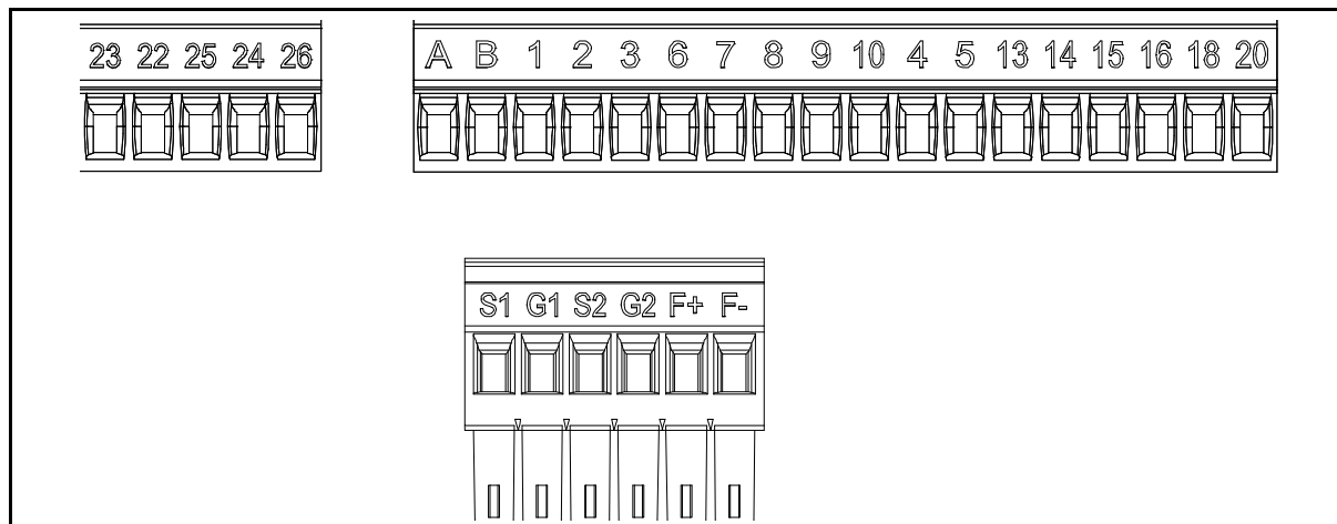
Figura 34. Morsetti di controllo.
