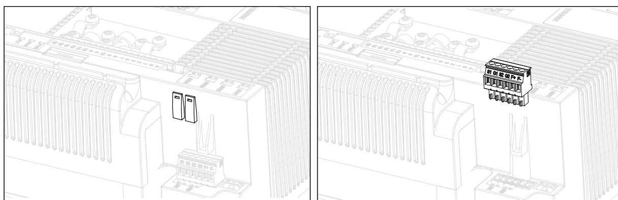
Figura 71. Rimozione dei jumper STO dall'unità di controllo.
