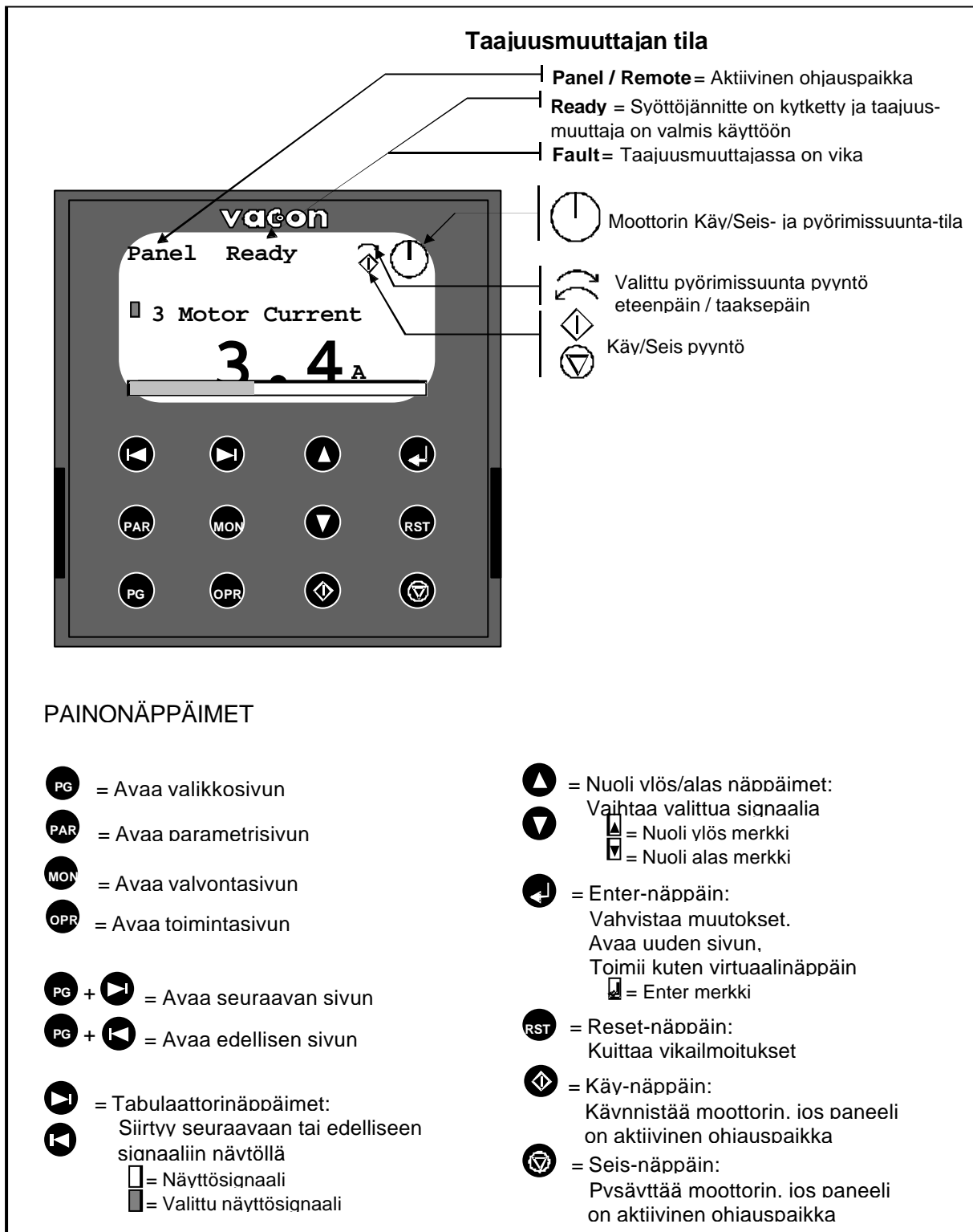
Kuva 1. Graafinen ohjauspaneeli LCD-näytöllä.
