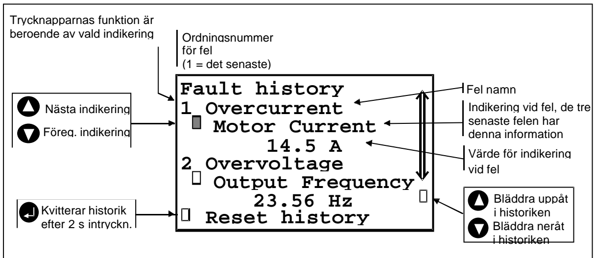
Figur 10. Felhistorik.
