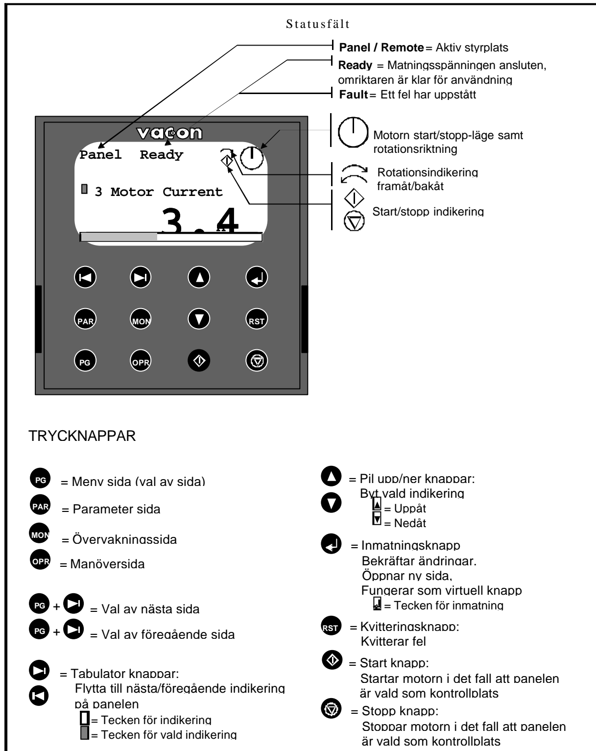
Figur 1. Grafisk kontrollpanel med LCD display.
