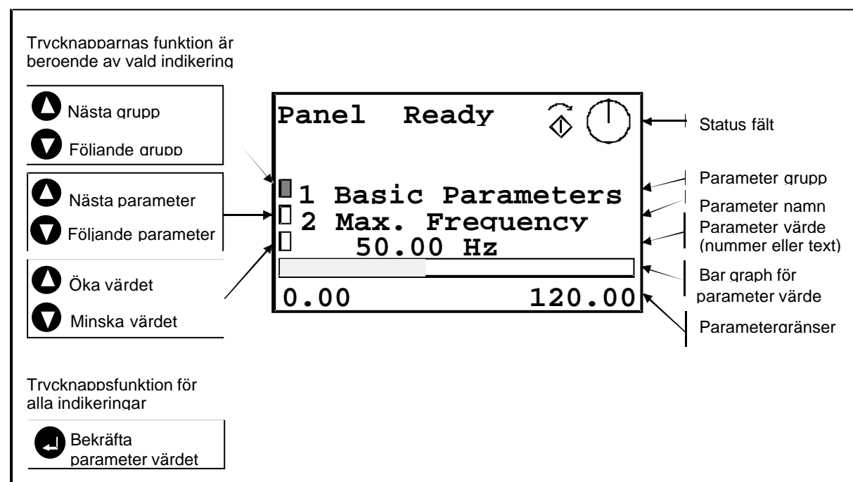
Figur 5. Inställning av parametrar.
