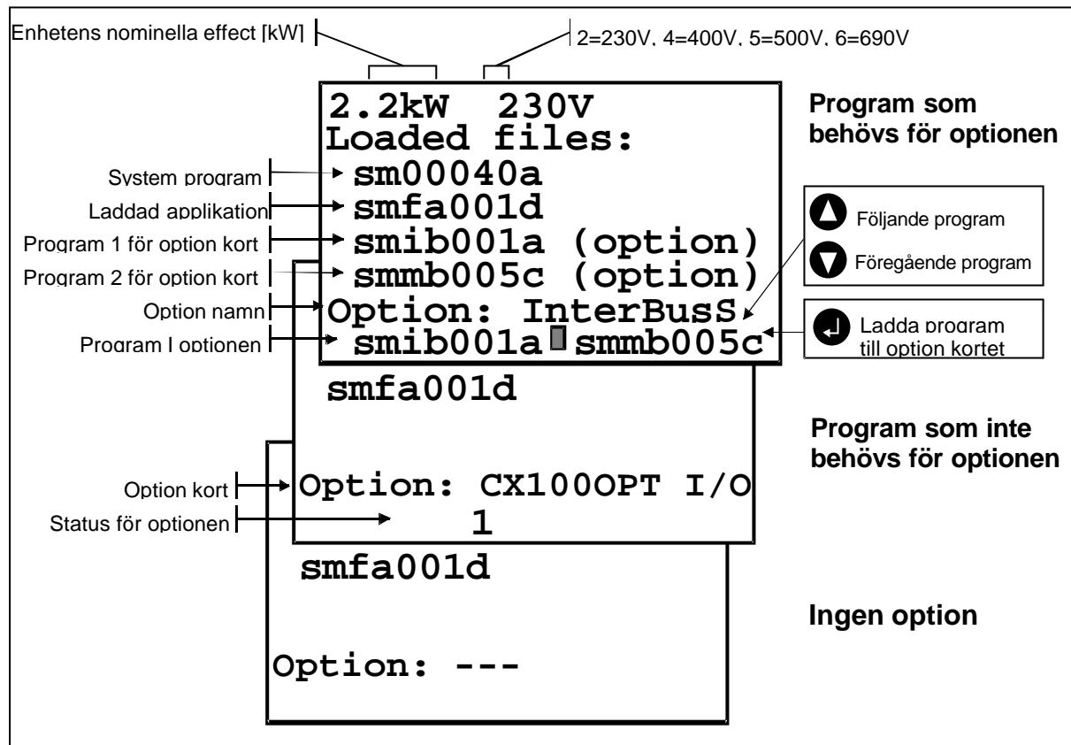
Figur 12. Program information och laddning av program till option kortet.
