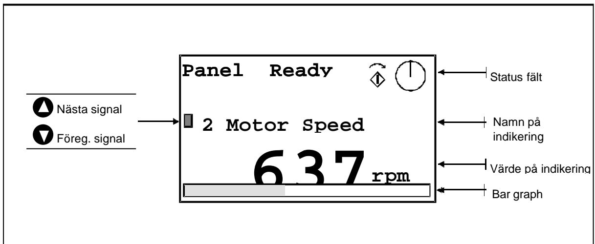
Figur 3. Övervakade signaler.
