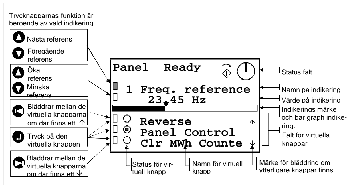
Figur 4. Inställning av referens och virtuella knappar.
