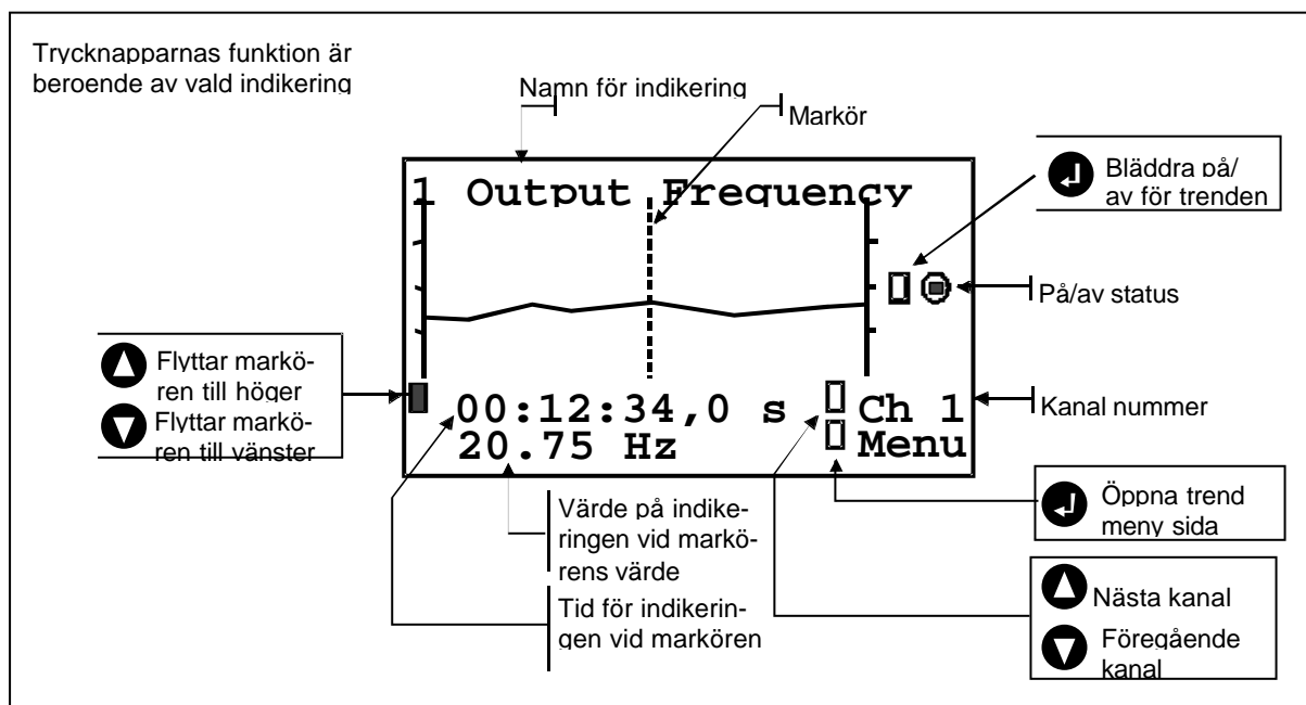
Figur 7. Trend sida.
