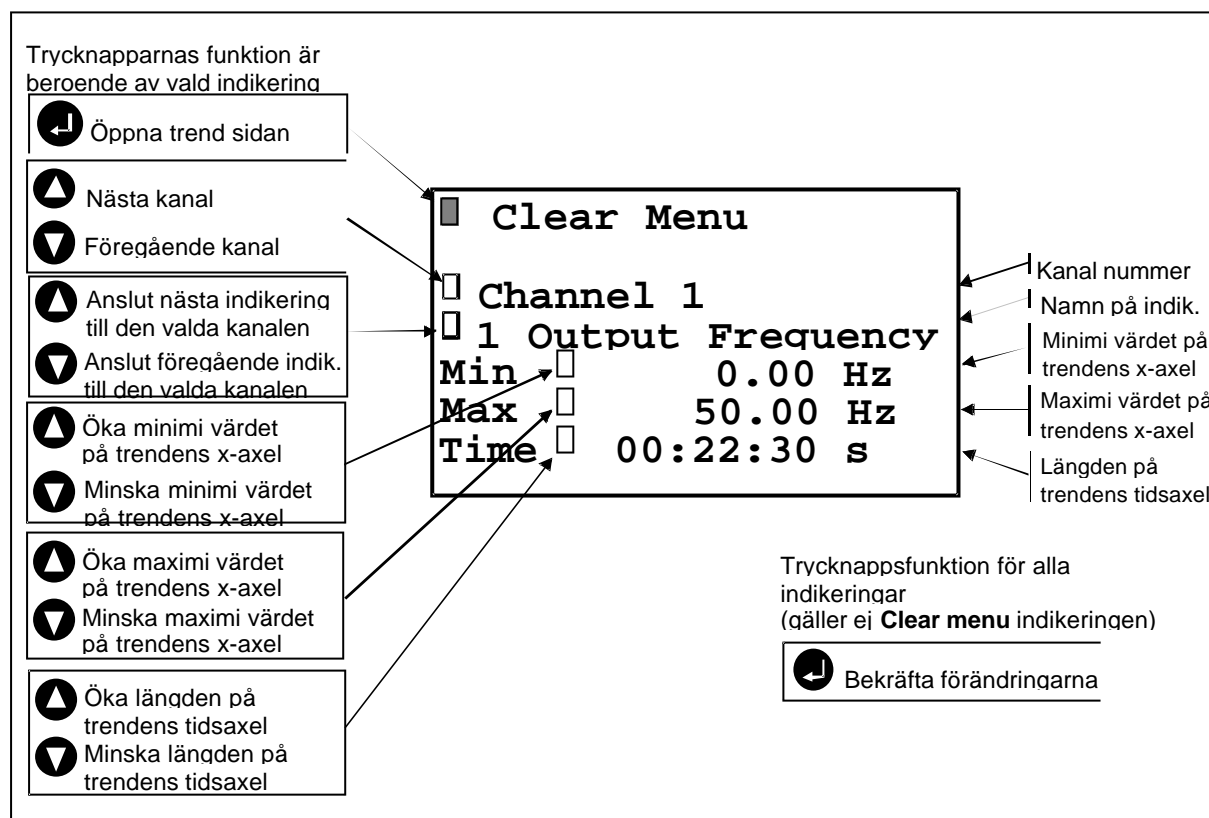
Figur 8. Anslutning av trendsignaler och ändring av trend skalor.
