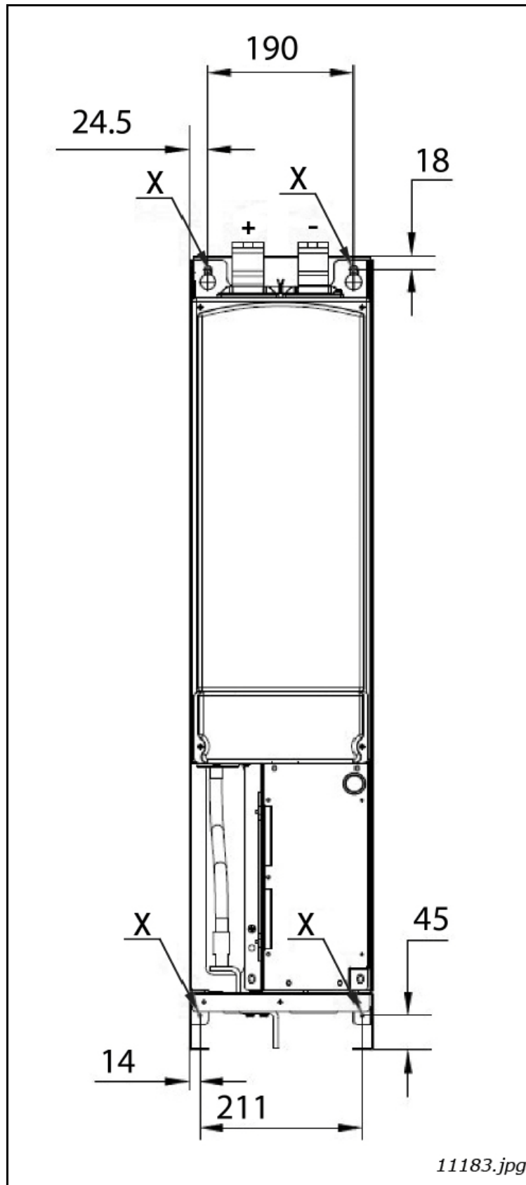
Abbildung 24. Befestigungspunkte der AFE-Einheit FI10
