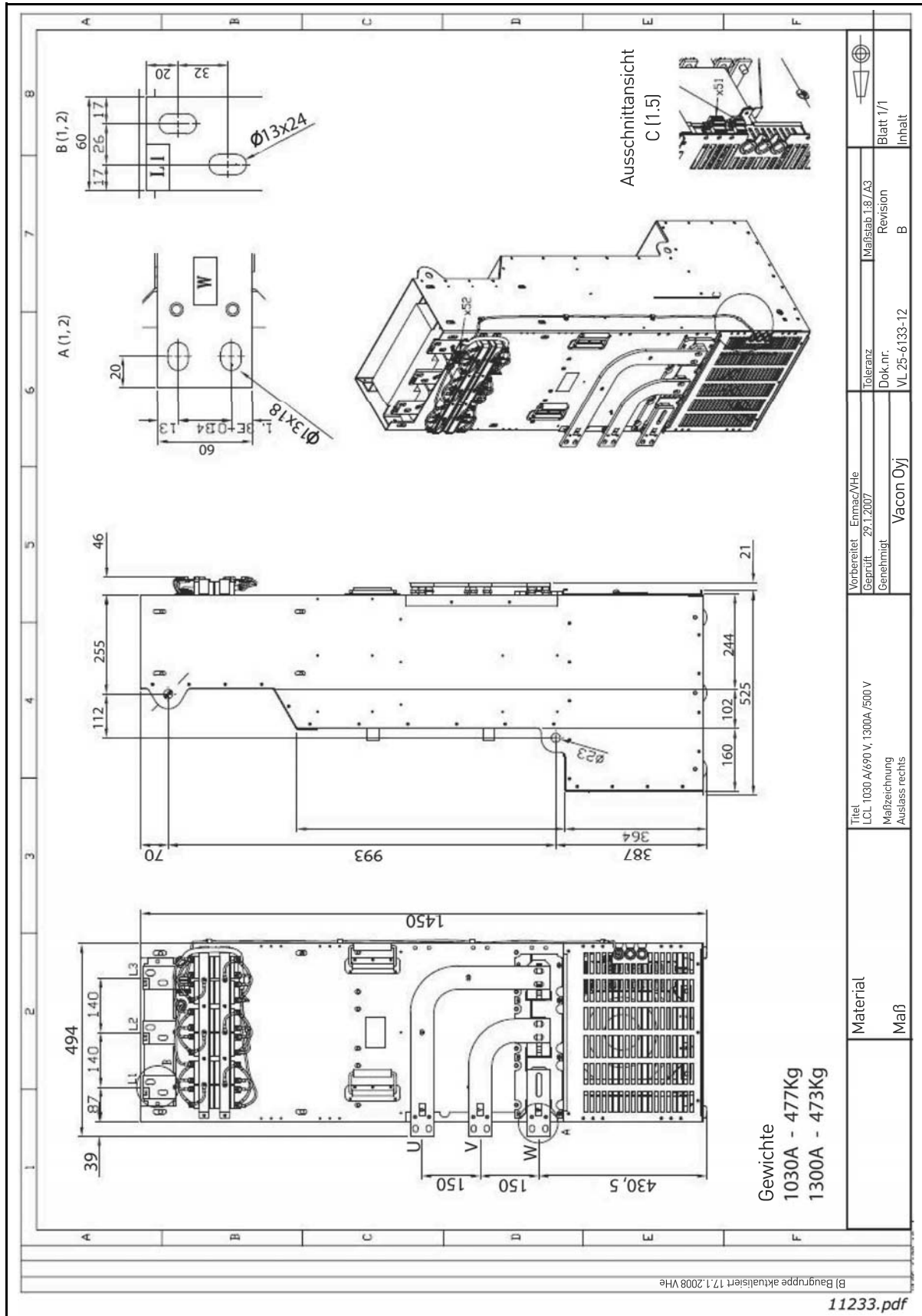
Abbildung 82. Abmessungen LCL-Filter F113, Ausgangsanschlüsse links
