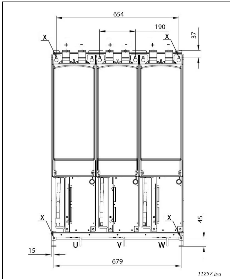
Abbildung 25. Befestigungspunkte der AFE-Einheit F113
