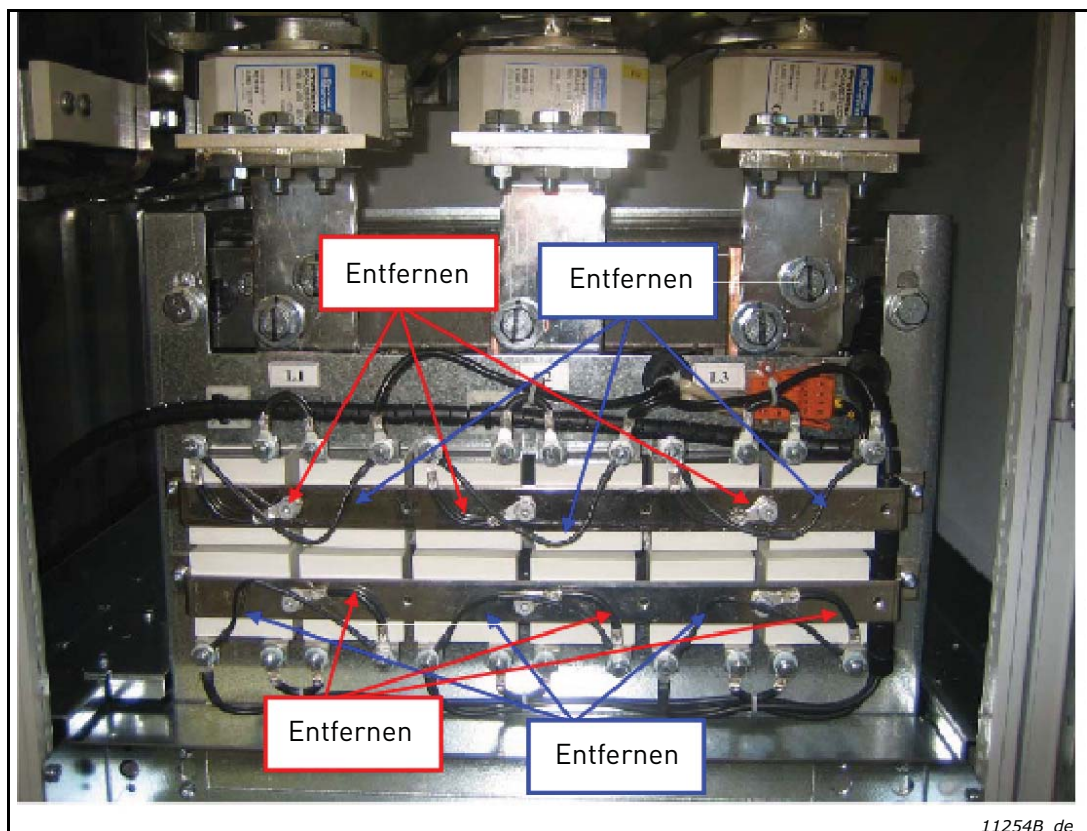
Abbildung 18. HF-Kondensatoren in FI13-LCL-Filtern
