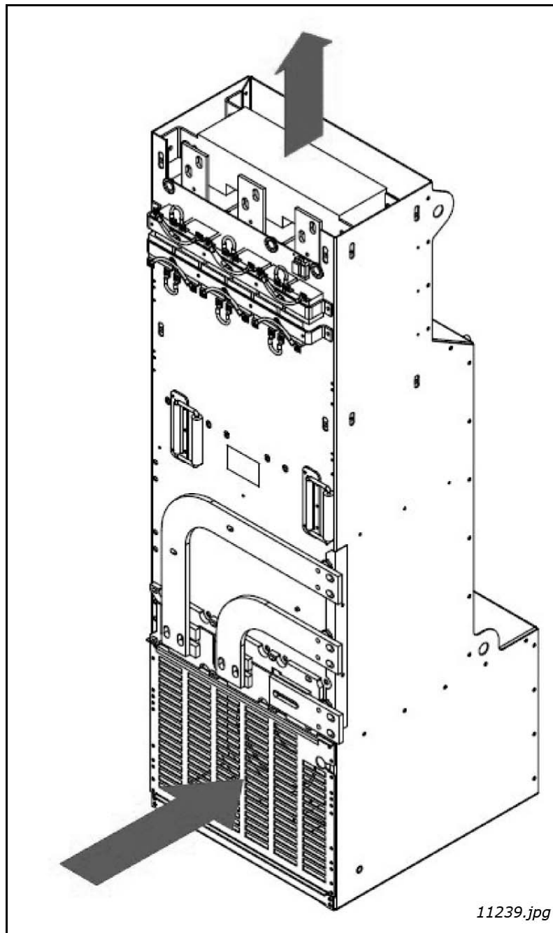
Abbildung 35. Luftleitelemente für FI13-LCL-Filter
