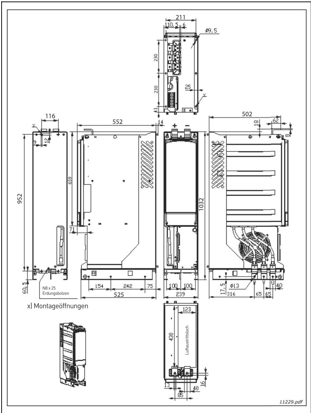
Abbildung 78. Abmessungen F110
