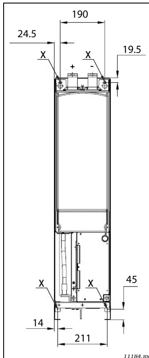
Abbildung 23. Befestigungspunkte der AFE-Einheit F19
