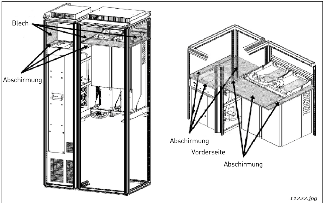
Abbildung 39. Luftleitelemente zur Schaltschrankkühlung für FI9- und FI10-AFE-Einheit und LCL-Filter
