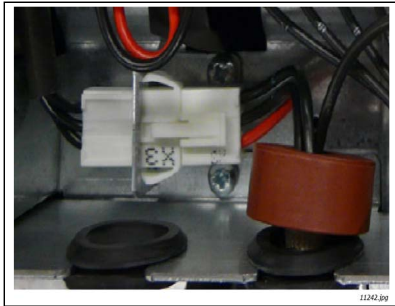
Abbildung 44. Klemme X3 (U-Phase bei FI13) in der Einheit
