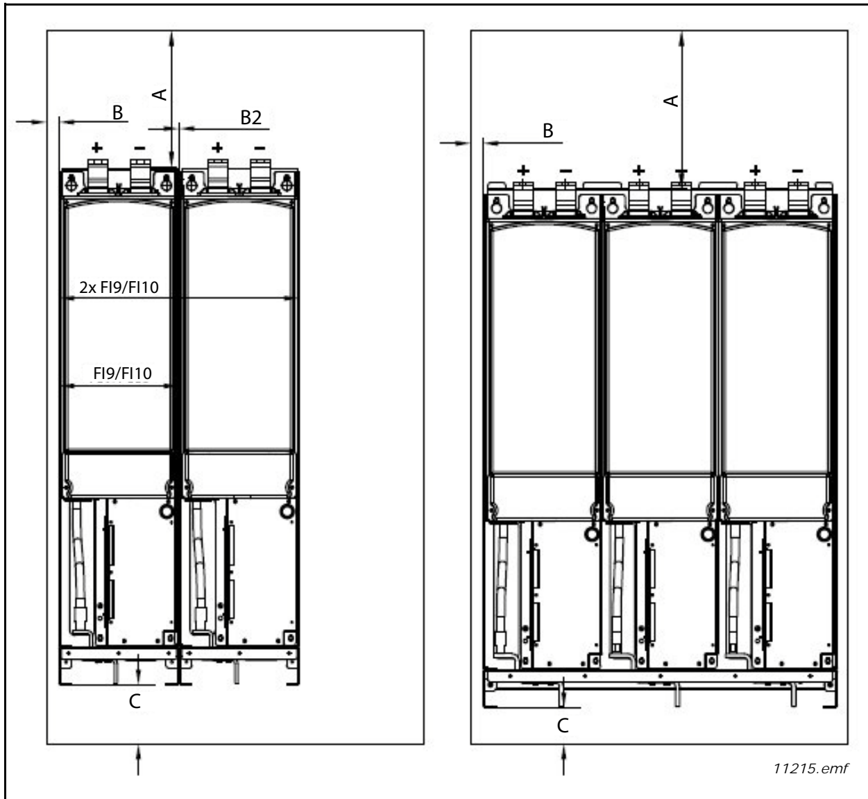
Abbildung 30. Installationsraum für FI9, FI10 und FI13
