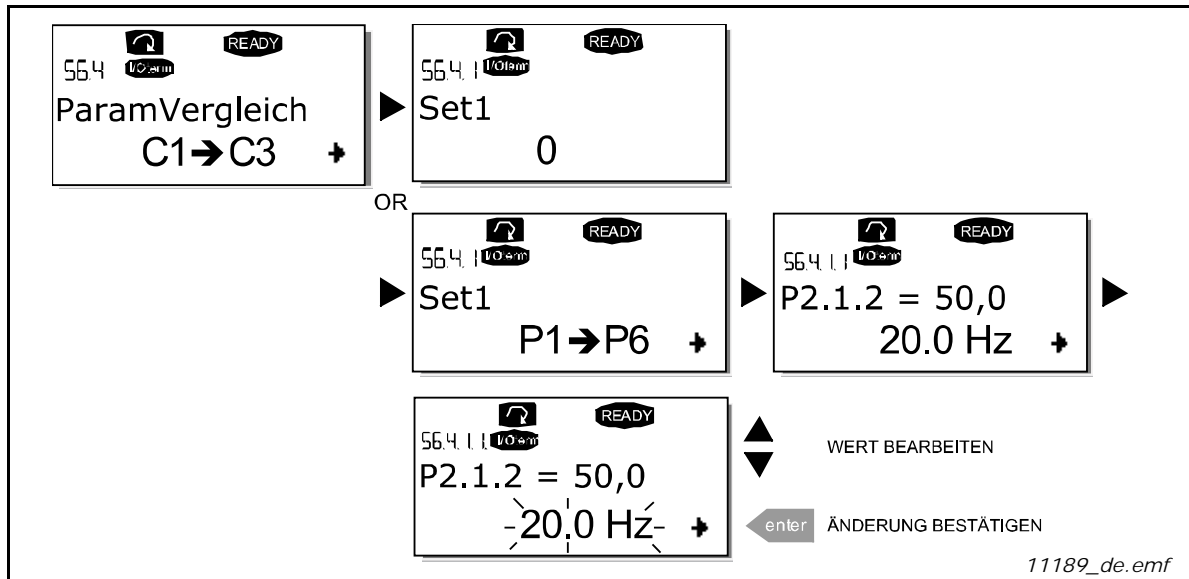
Abbildung 66. Parametervergleich
