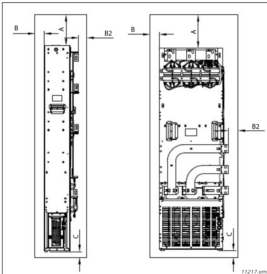
Abbildung 33. Installationsabstand
