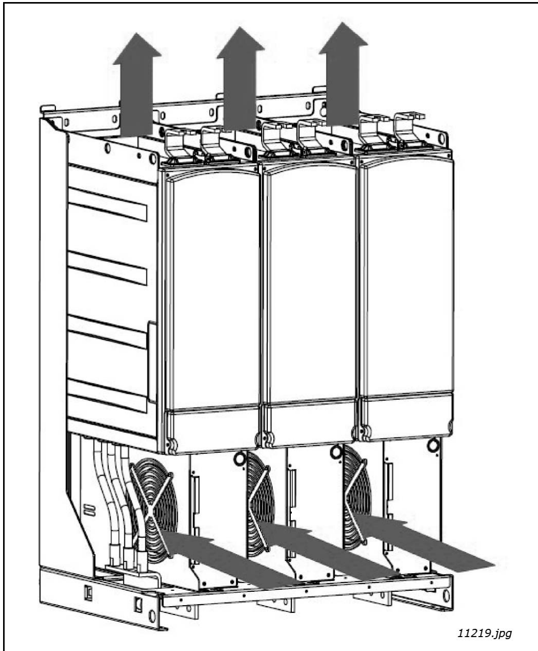
Abbildung 32. Kühlluftstrom bei der FI13-Einheit
