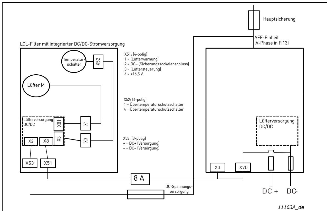
Abbildung 43. Anschlussschema der integrierten DC/DC-Versorgung
