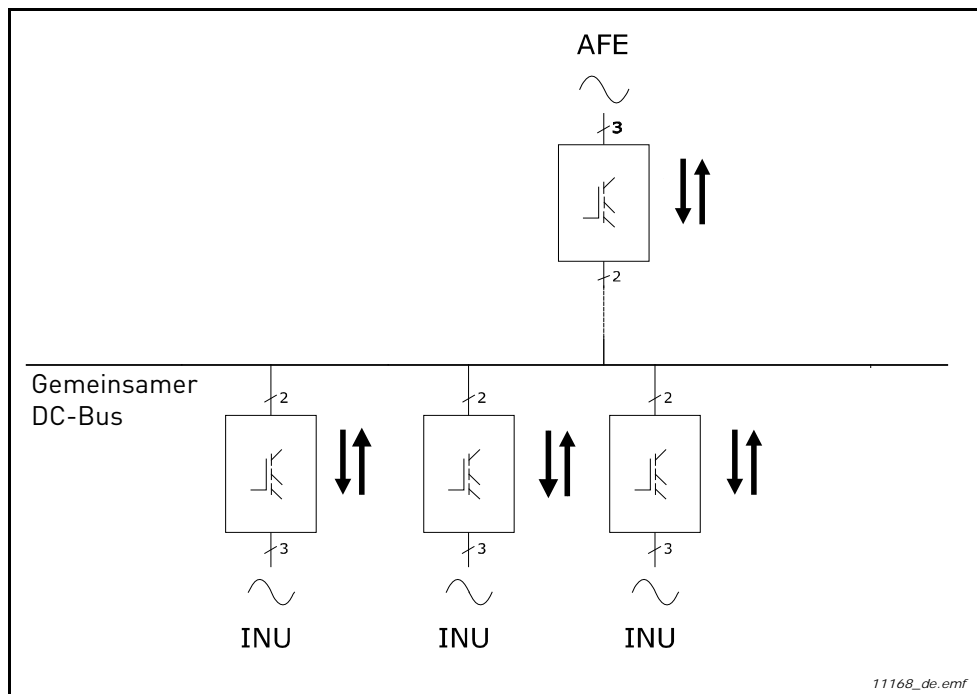
Abbildung 5. Typische Active Front End-Konfiguration
