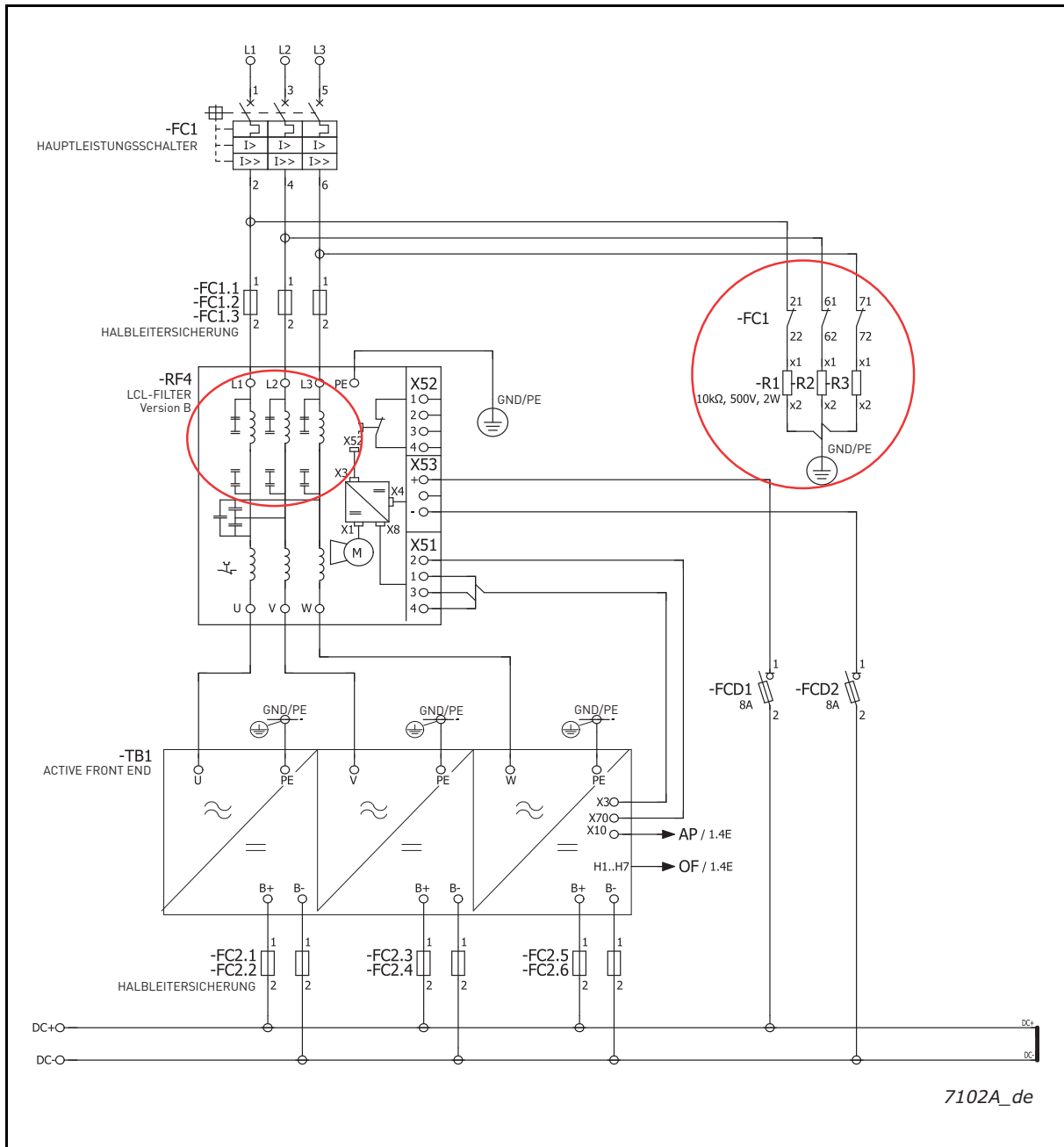
Abbildung 16. Anschlussschema für den LCL- und AFE-Kreis bei der Verwendung in Installationen mit Erdschluss-Schutzrelais oder in einem IT-Netzwerk oder wenn AFE-Einheiten anderer Hersteller Anschluss an die dieselbe Transformator-Sekundärversorgung haben
