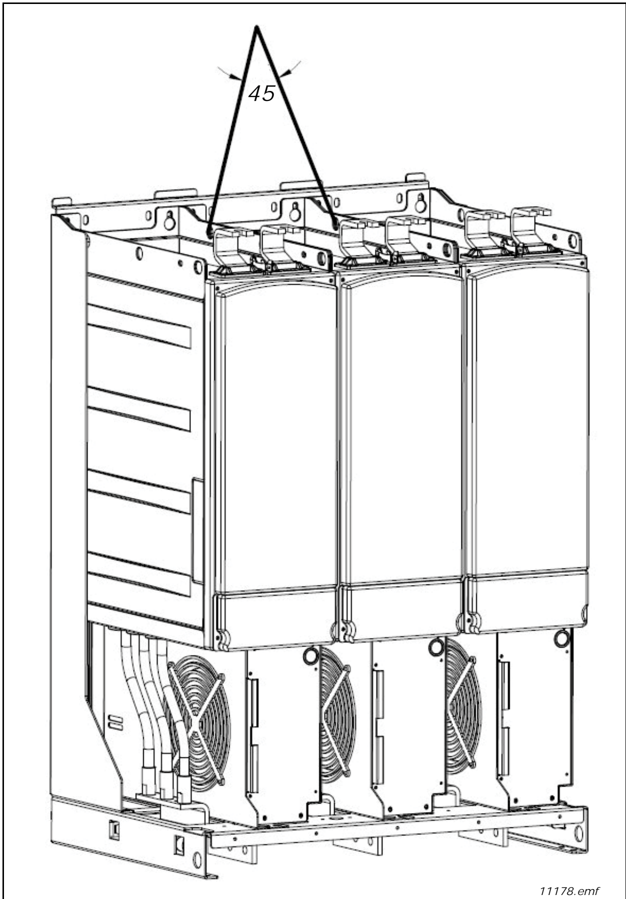
Abbildung 2. Hebepunkte für Module F113
