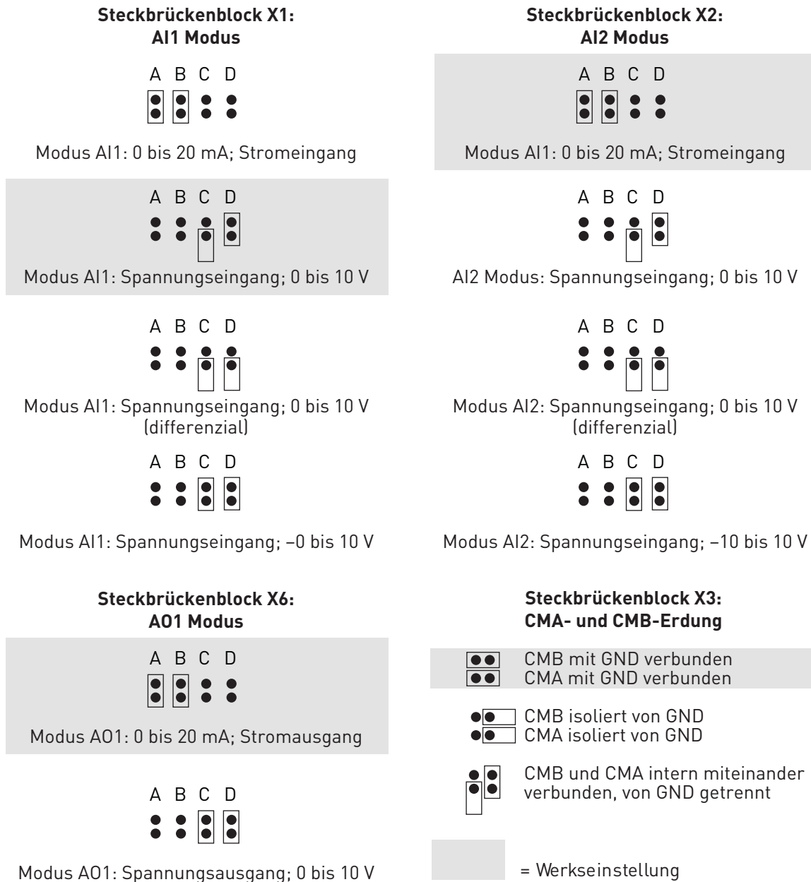
Abbildung 52. Steckbrückenauswahlmöglichkeiten für OPTA1
