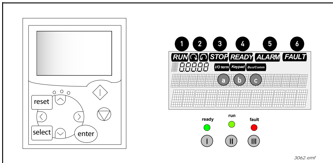
Abbildung 56. VACON®-Steuertafel und Gerätestatusanzeigen
