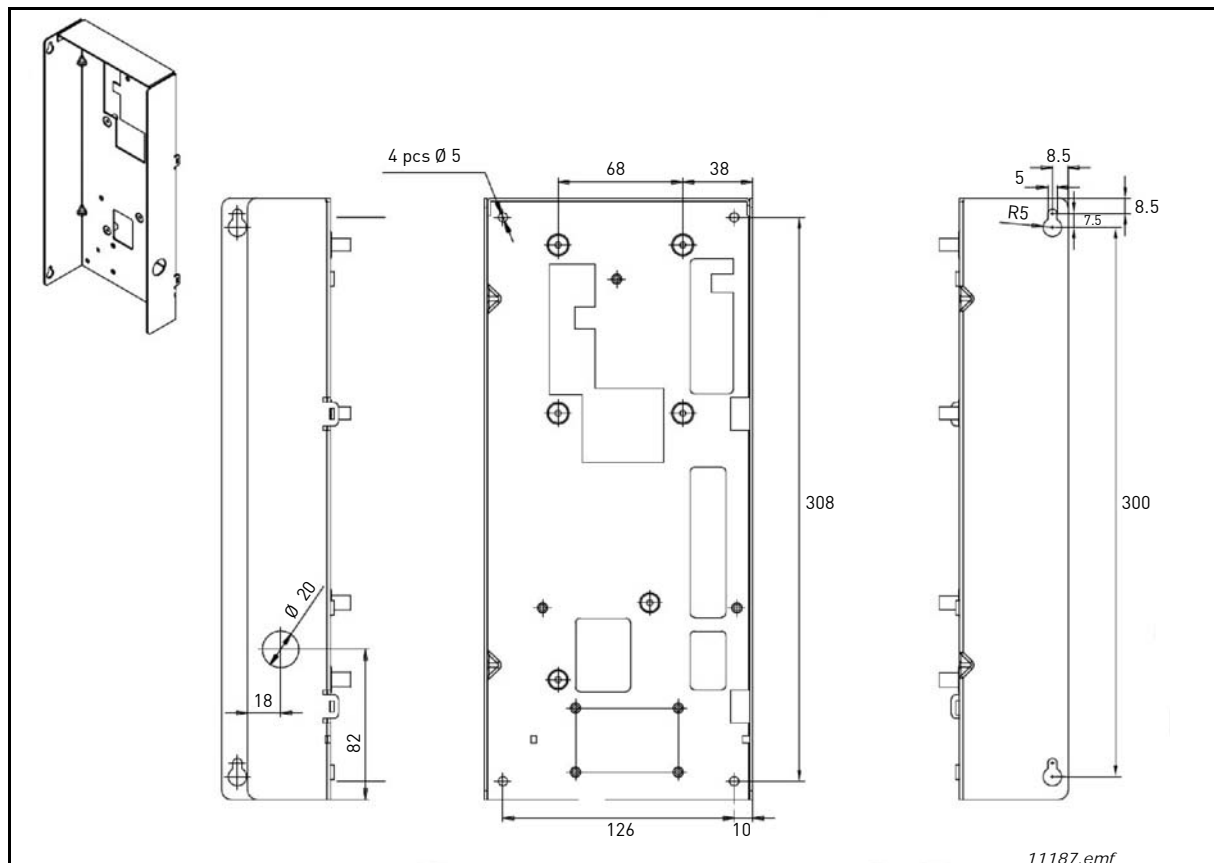
Abbildung 29. Befestigungspunkte der Steuereinheit
