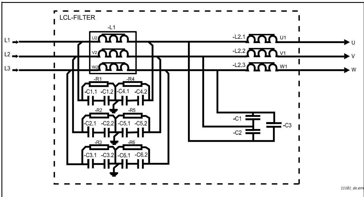
Abbildung 14. Anschlussschema für VACON® LCL-Filter
