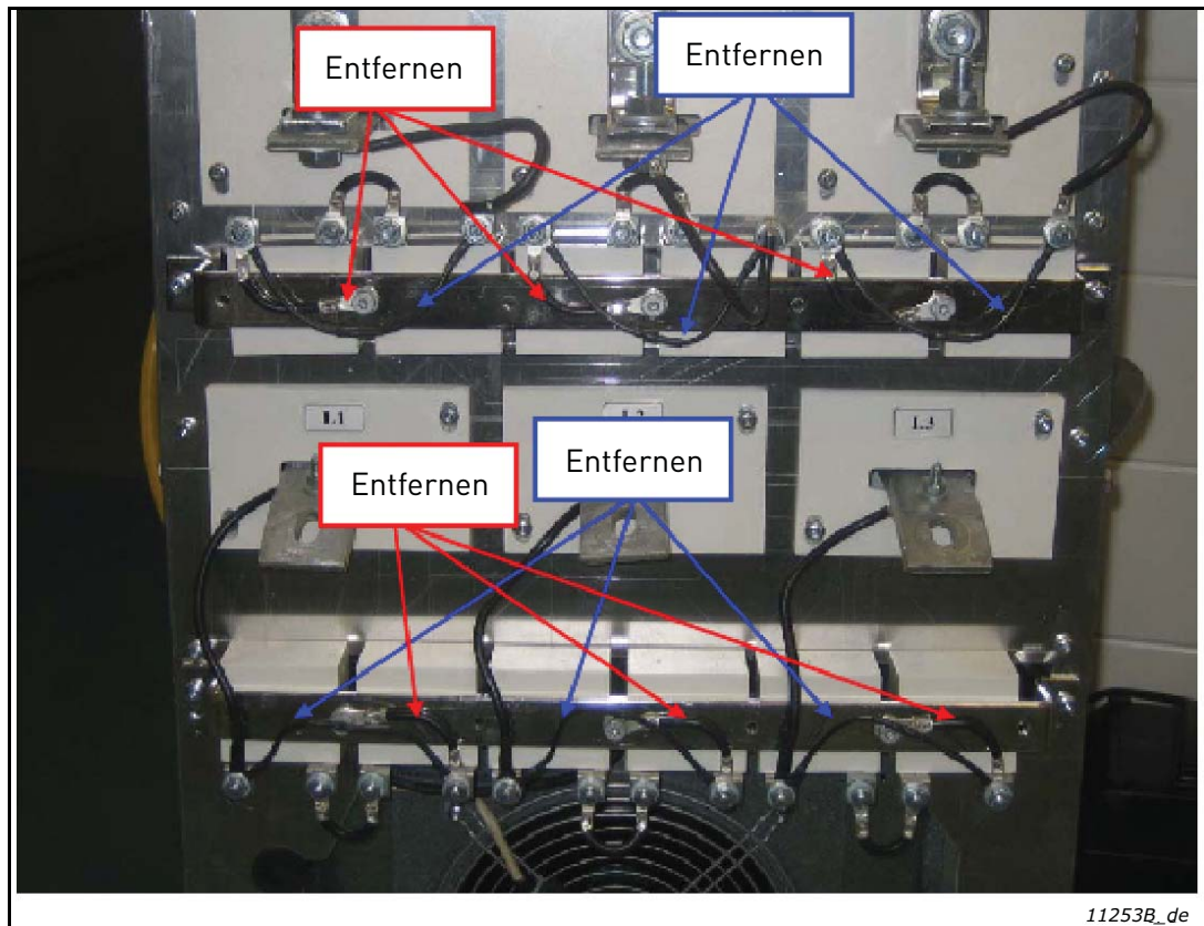
Abbildung 17. HF-Kondensatoren in FI9- und FI10-LCL-Filtern
