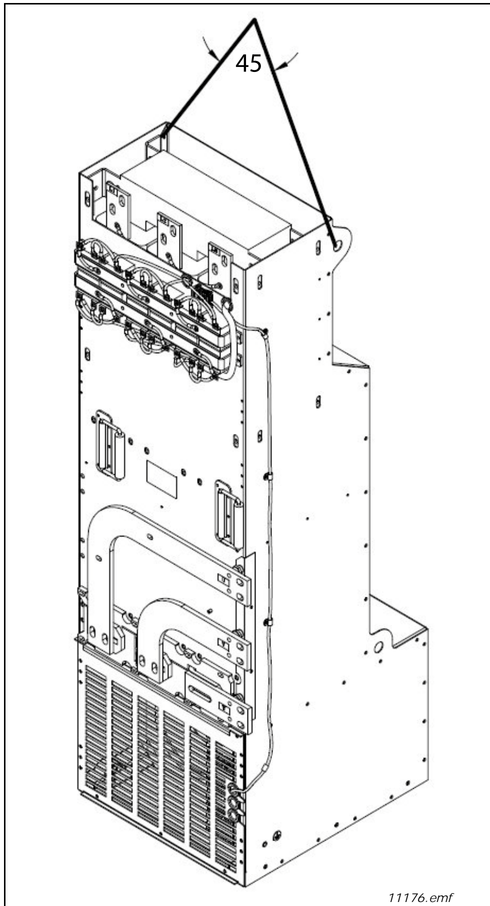
Abbildung 4. Hebepunkte für LCL-Filter FI13
