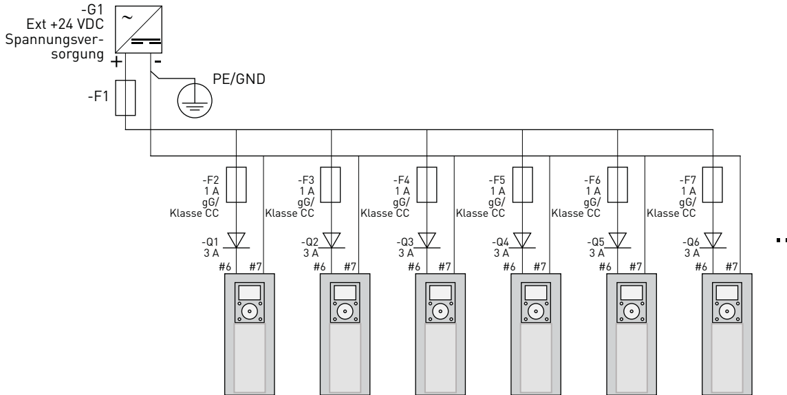
Abbildung 47. Parallele Verbindung der 24-V-Eingänge mit vielen Frequenzumrichter
