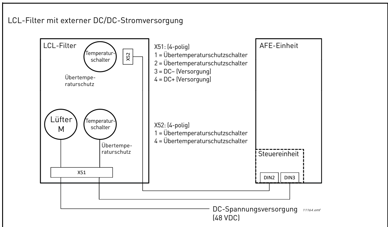
Abbildung 45. Anschlussschema der externen DC/DC-Versorgung
