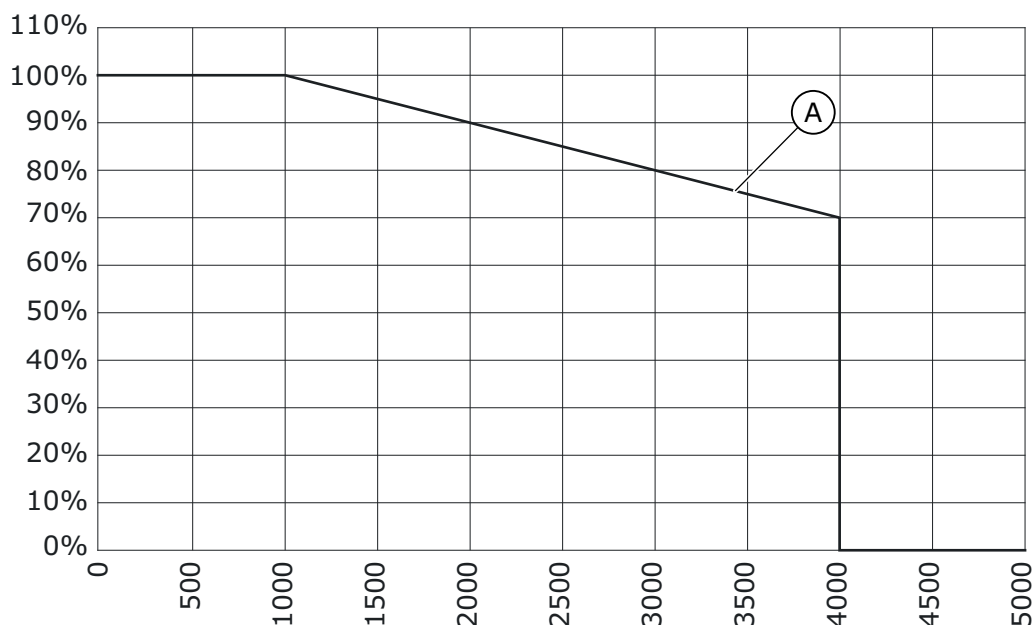
Abbildung 22. Überlastungen in großen Höhen
