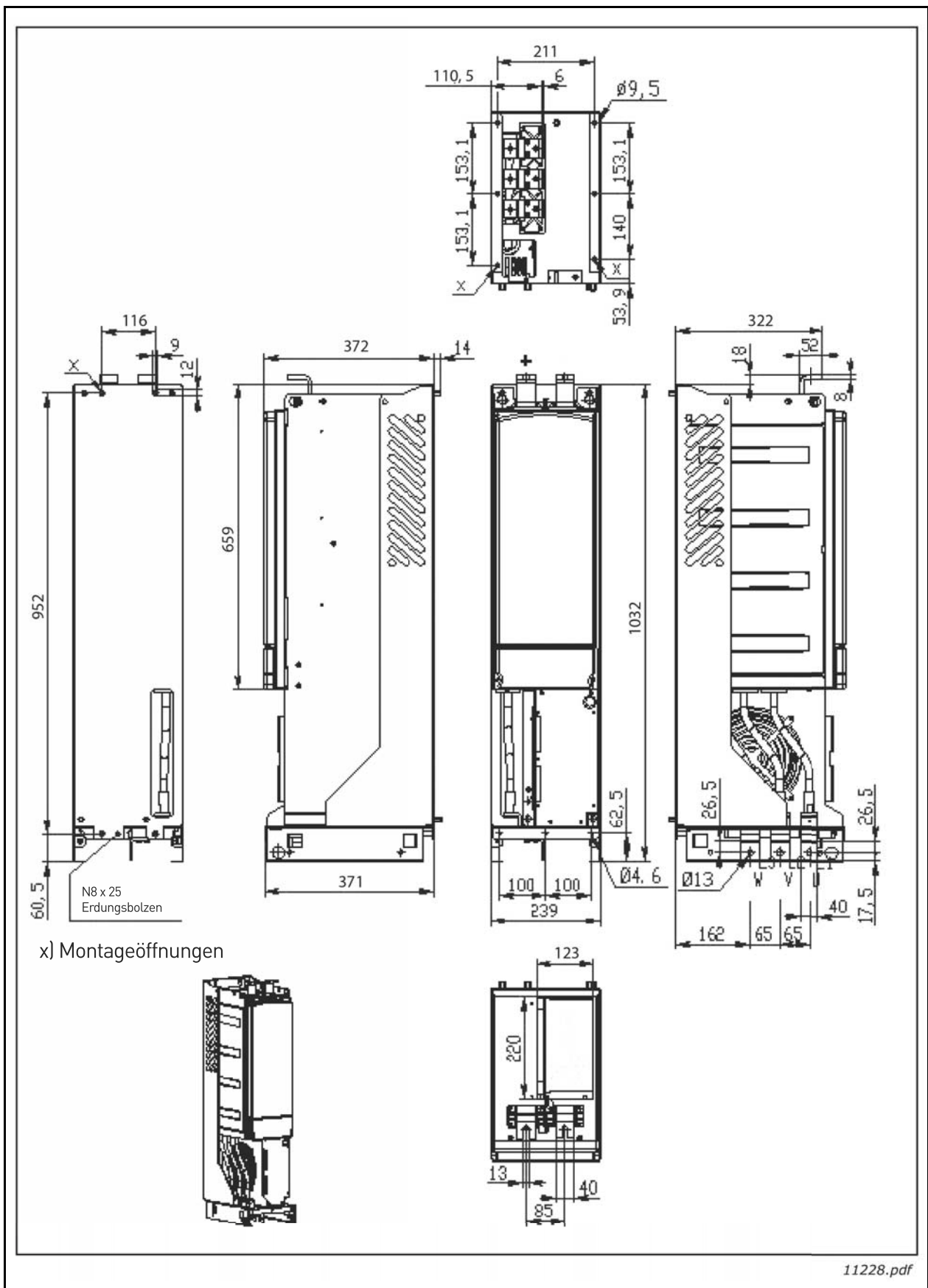
Abbildung 77. Abmessungen F19
