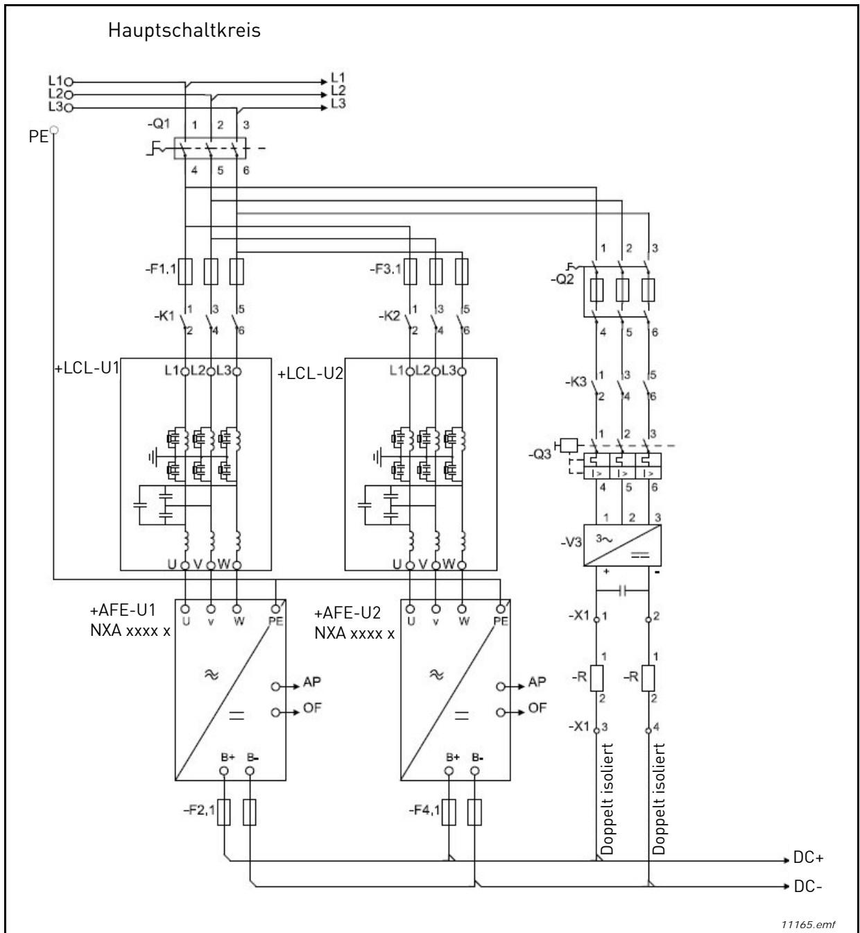
Abbildung 19. Parallelschaltung von Active-Front-End-Geräten mit einer gemeinsamen Vorladeschaltung
