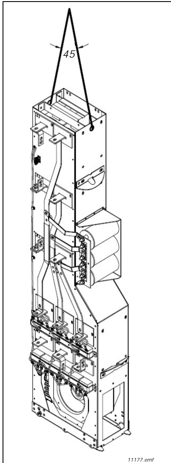
Abbildung 3. Hebepunkte für LCL-Filter FI9 und FI10
