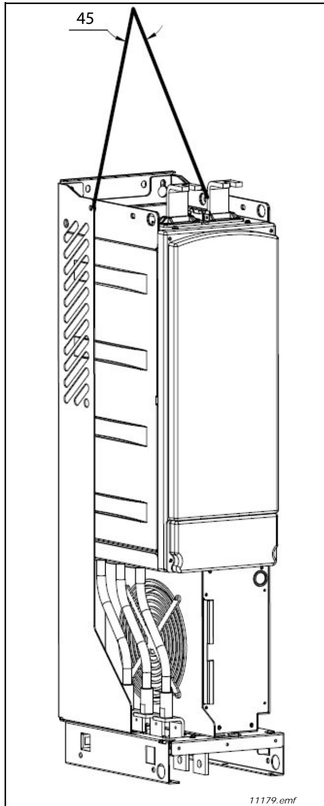
Abbildung 1. Hebepunkte für Module FI9 und FI10
