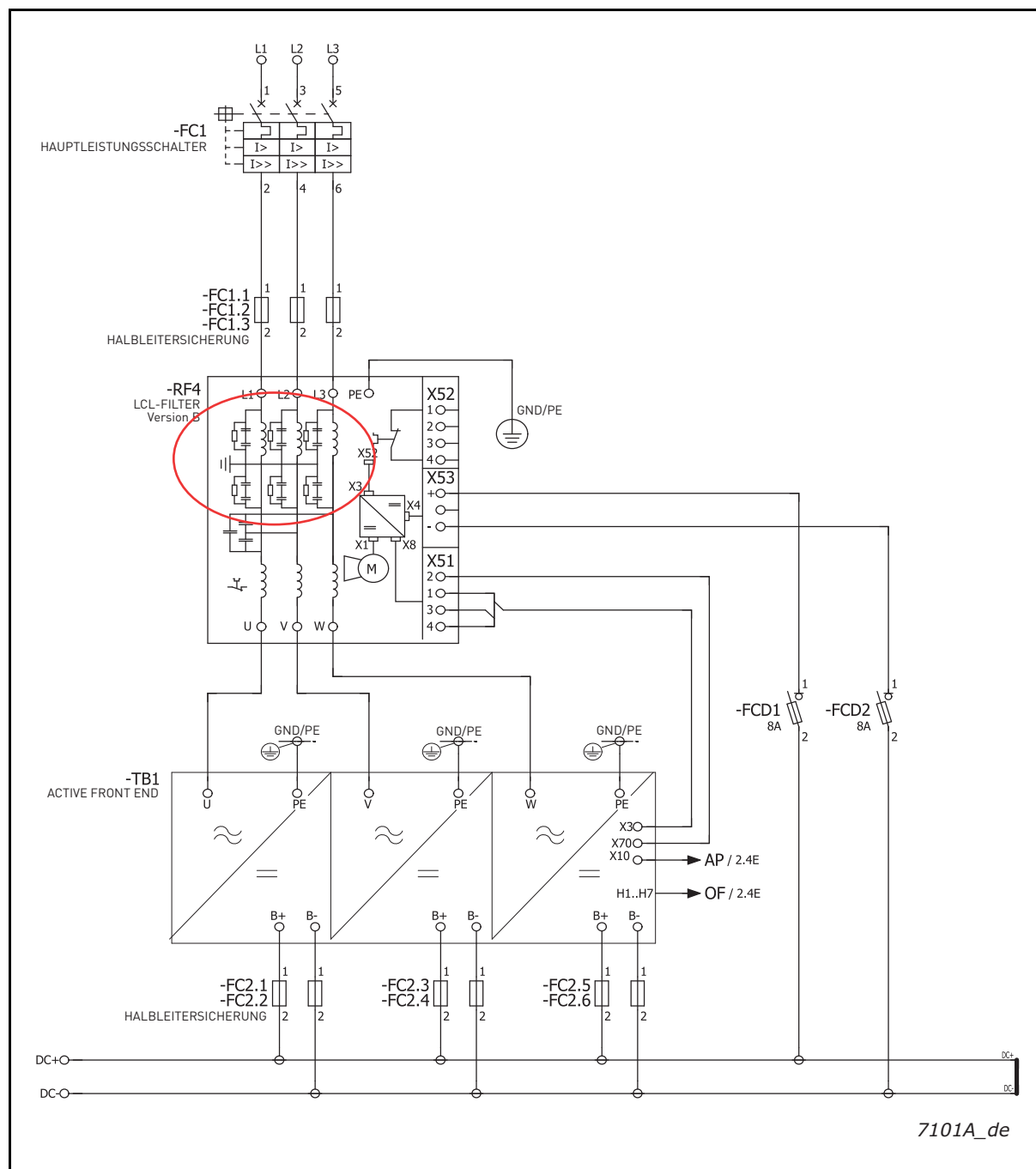
Abbildung 15. Anschlussschema des Standard-LCL-Filters
