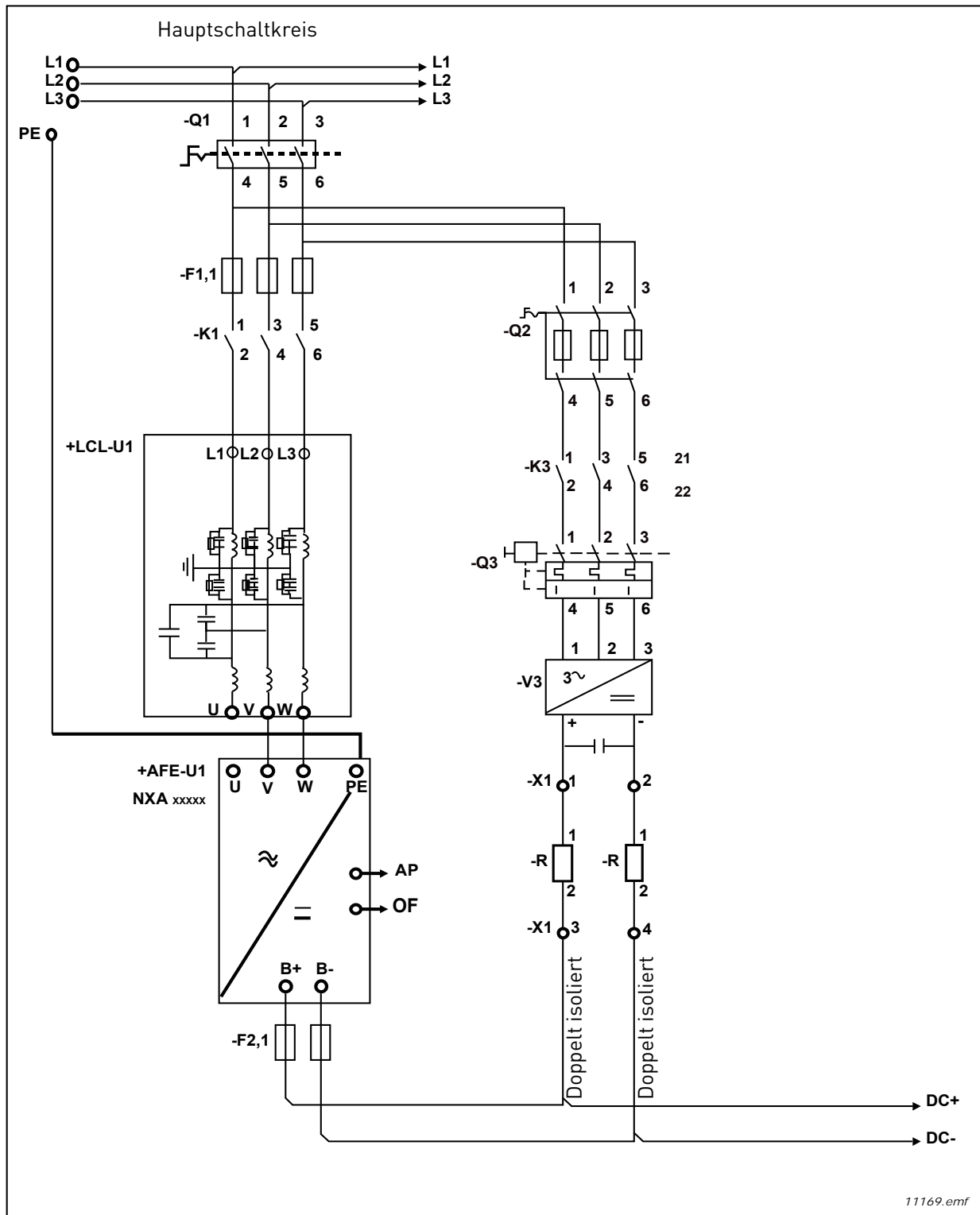
Abbildung 6. Anschlüsse eines VACON® Active-Front-End-Einzelgeräts
