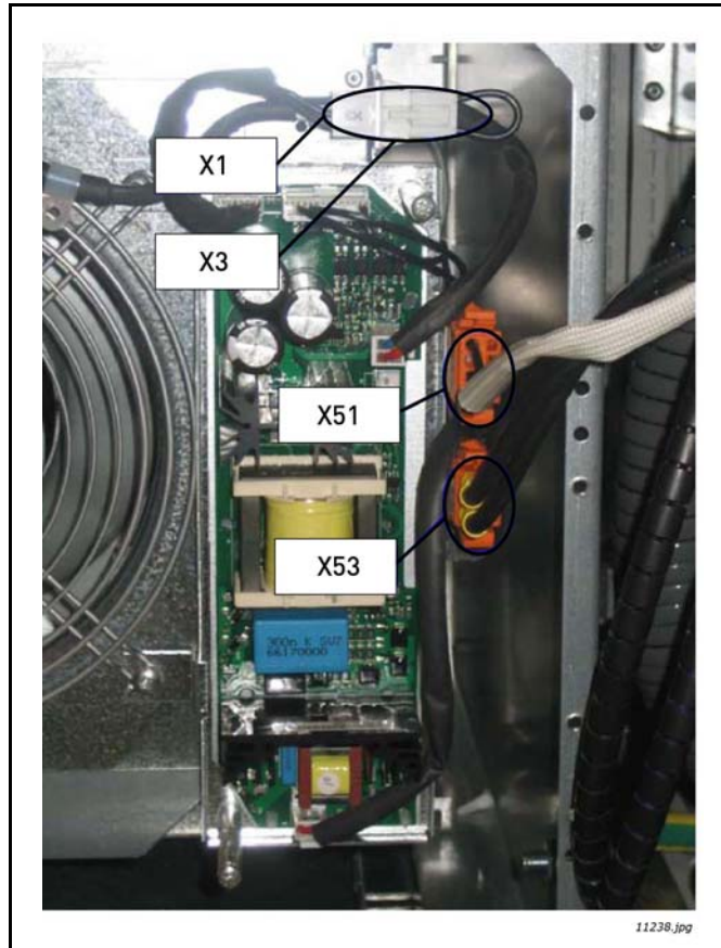
Abbildung 42. Integrierte DC/DC-Stromversorgung für F113-LCL-Filter
