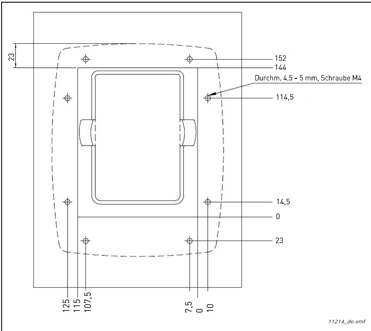
Abbildung 86. Abmessungen des Tür-Einbausatzes
