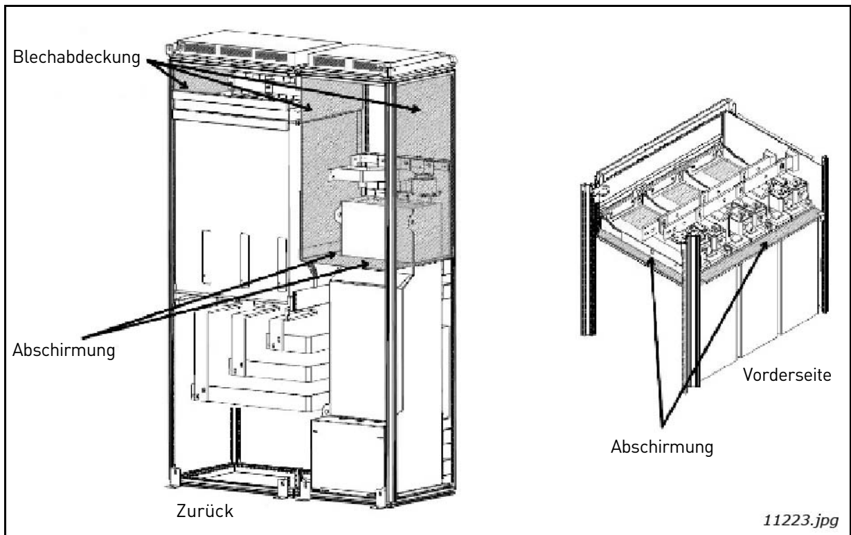
Abbildung 40. Luftleitelemente zur Schaltschrankkühlung für FI13-AFE-Einheit und LCL-Filter
