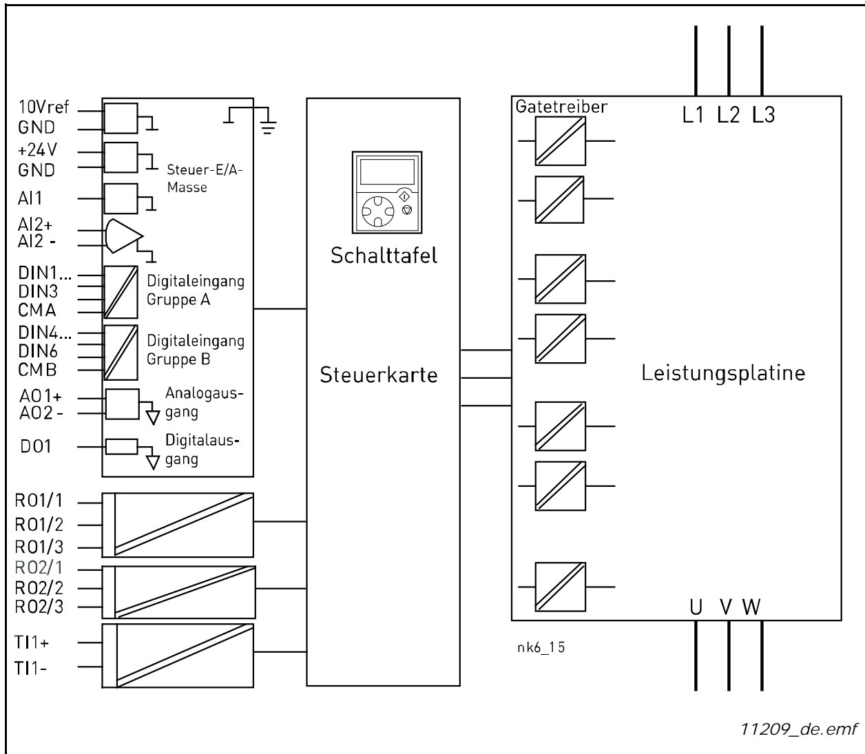
Abbildung 55. Galvanische Trennung
