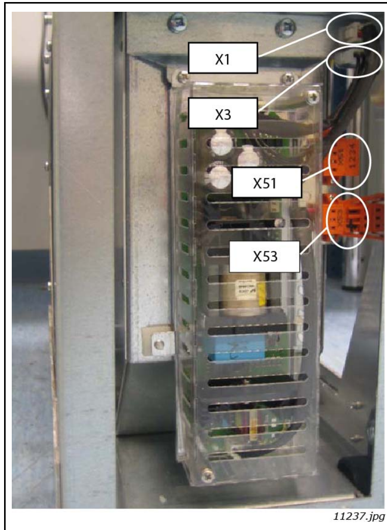
Abbildung 41. Integrierte DC/DC-Stromversorgung für FI9- und FI10-LCL-Filter
