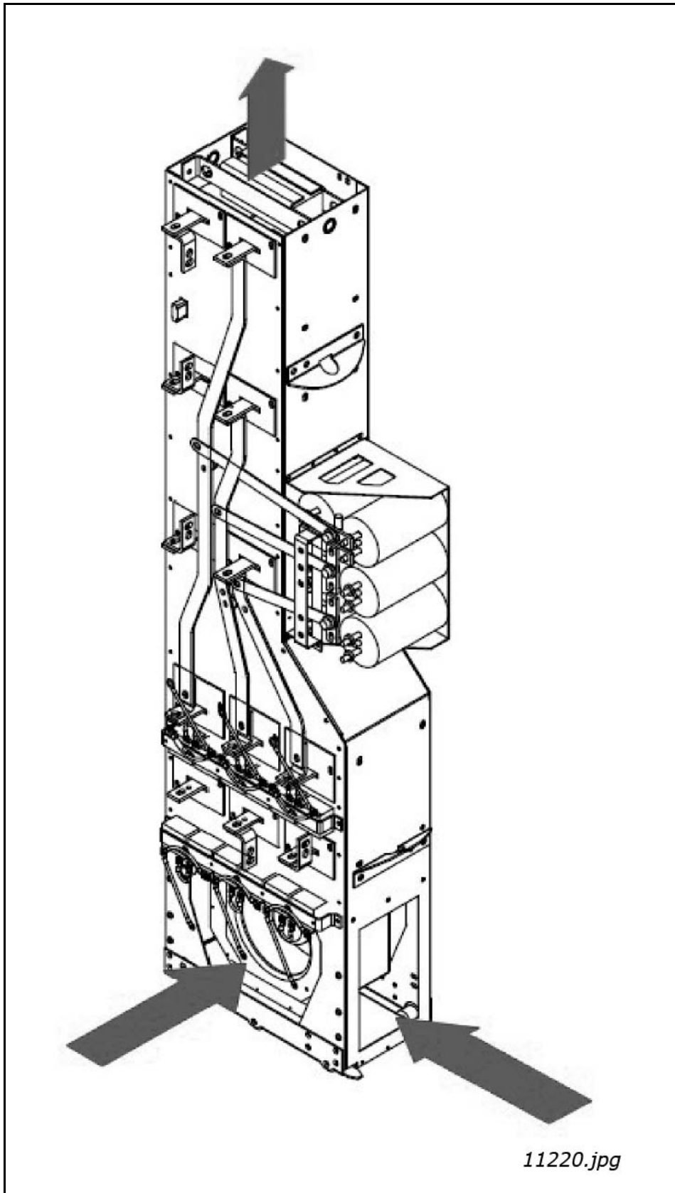
Abbildung 34. Kühlluftstrom bei FI9- und FI10-LCL-Filtern
