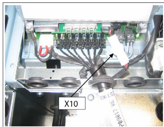
Abbildung 13. Glasfaserkabelklemmen in der Einheit (Beispiel F113)
