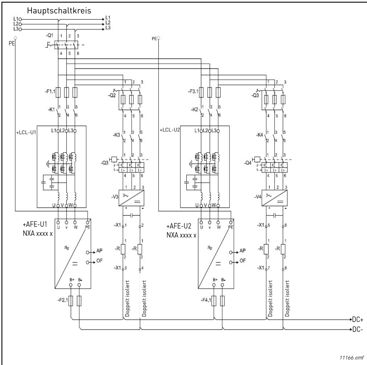
Abbildung 20. Parallelschaltung von Active-Front-End-Geräten mit eigenen Vorladeschaltungen
