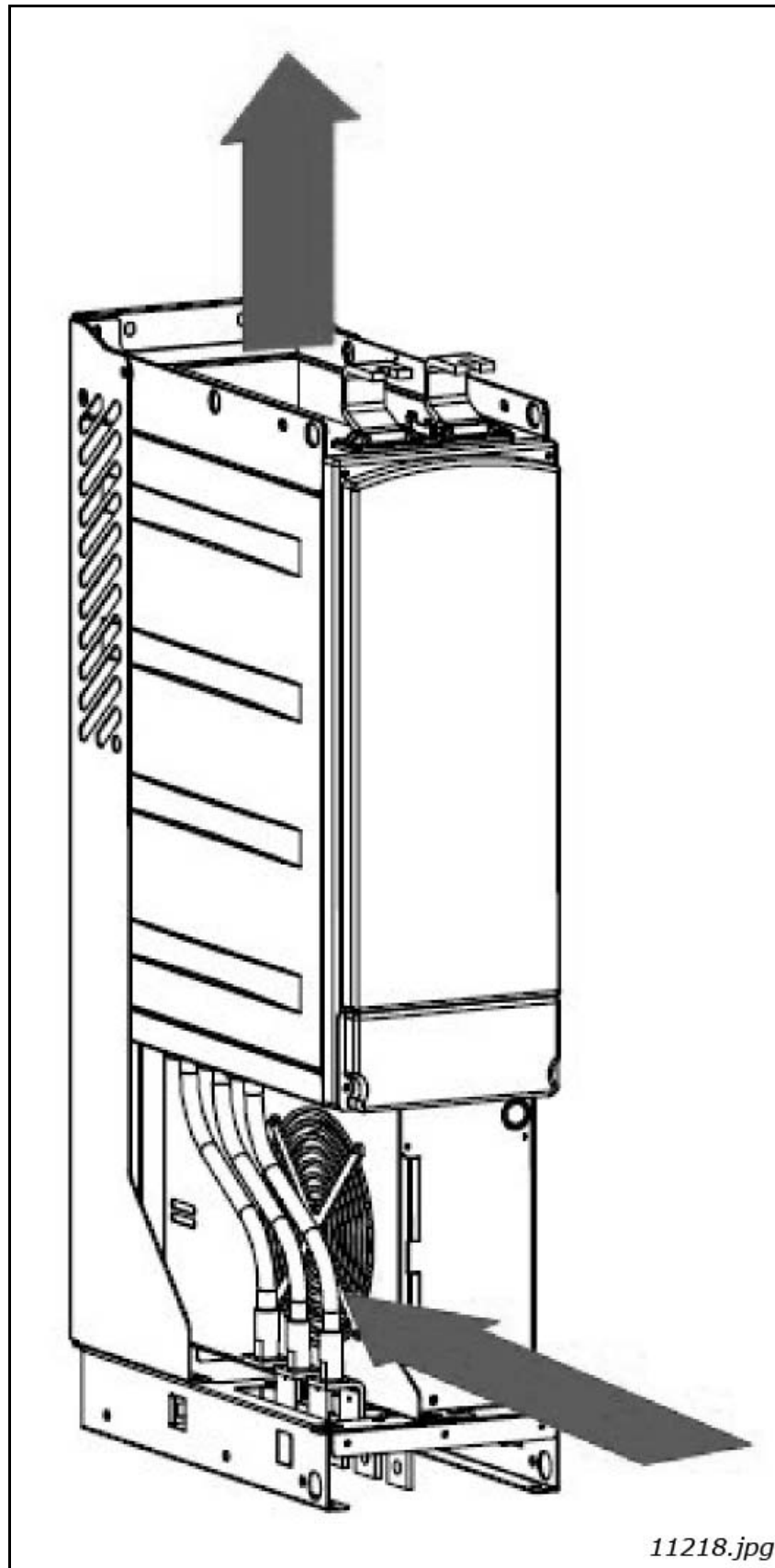
Abbildung 31. Kühlluftstrom bei F19- und F110-Einheiten
