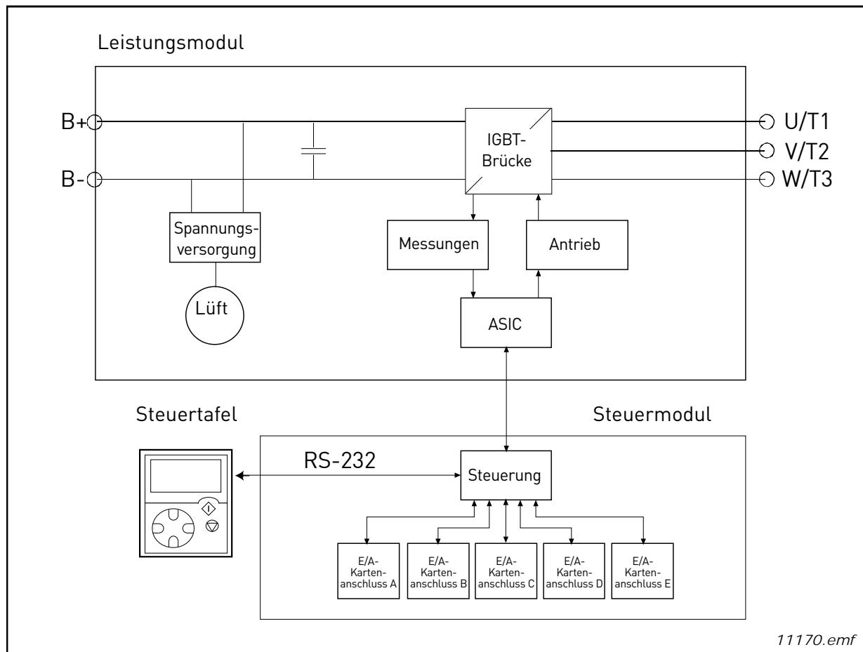
Abbildung 7. NXA-Blockschaltbild
