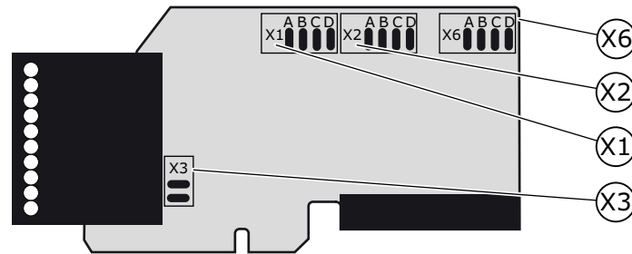
Abbildung 51. Steckbrückenblöcke auf OPTA1
