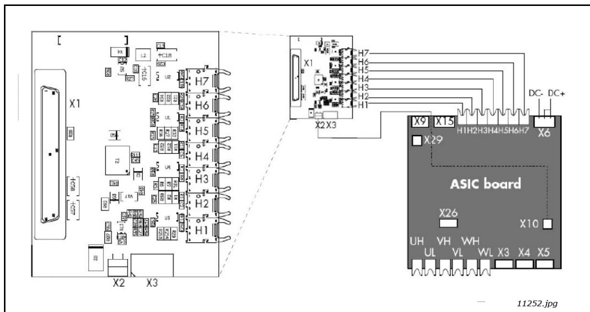
Abbildung 11. Adapterkarte für optische Kabel
