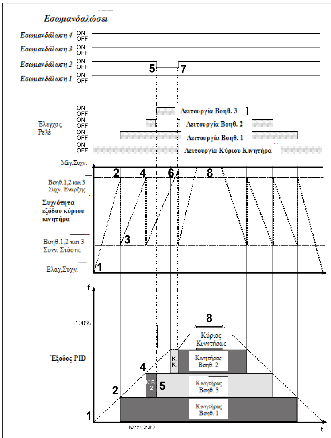
Σχήμα 7-4. Παράδειγμα της λειτουργίας της εφαρμογής Ελέγχου Αντλίας και Ανεμιστήρα (PFC) με 3 βοηθ. κινητήρες.
