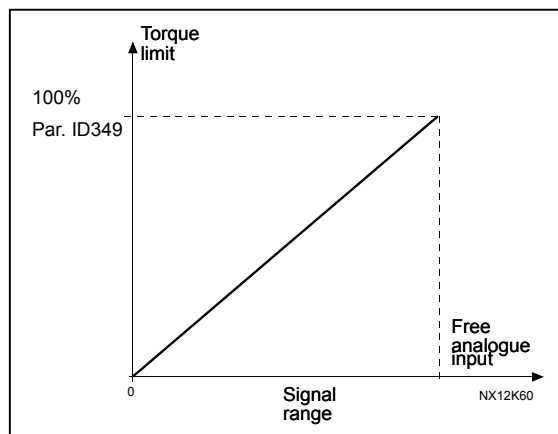
Σχήμα 8-29. Μείωση του ορίου επίβλεψης ροπής
