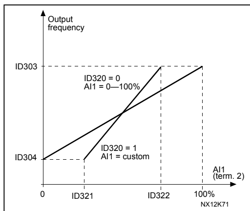
Σχήμα 8-18. AI1 καμία αναστροφή σήματος
