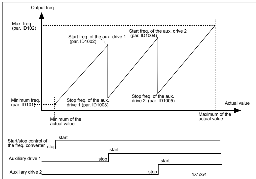
Σχήμα 8-59. Παράδειγμα του μετατροπέα συχνότητας και δύο βοηθητικών κινητήρων με παράκαμψη του ελεγκτή PID
