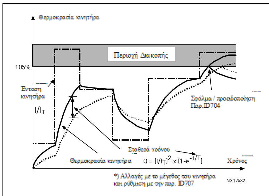
Σχήμα 8-48. Υπολογισμός της θερμοκρασίας του κινητήρα
