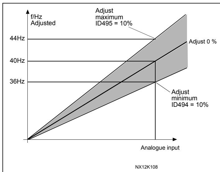
Σχήμα 8-41. Ένα παράδειγμα ρύθμισης της εισόδου
