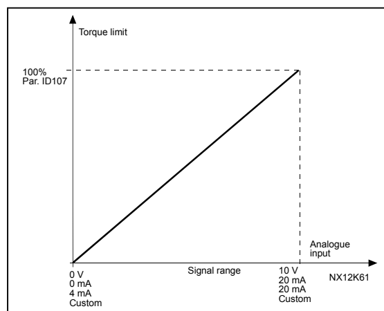
Σχήμα 8-26. Κλιμάκωση της μέγ. έντασης κινητήρα
