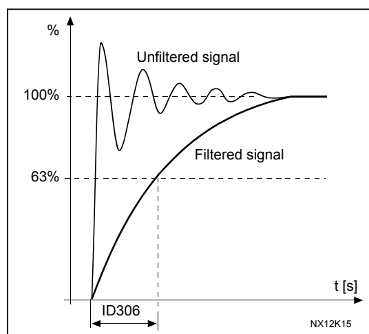
Σχήμα 8-12. Φιλτράρισμα αναφοράς
