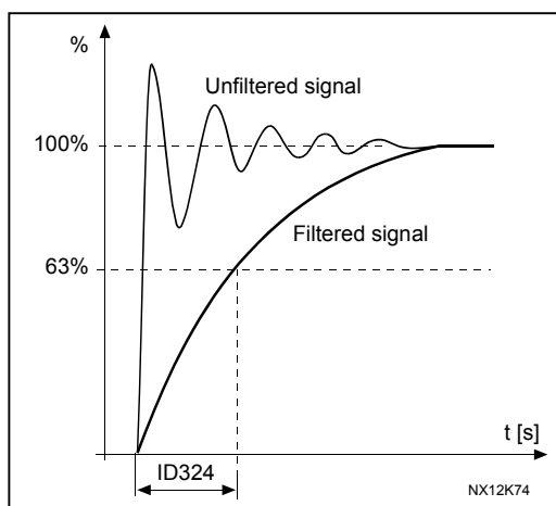
Σχήμα 8-20. AI1 φιλτράρισμα σήματος
