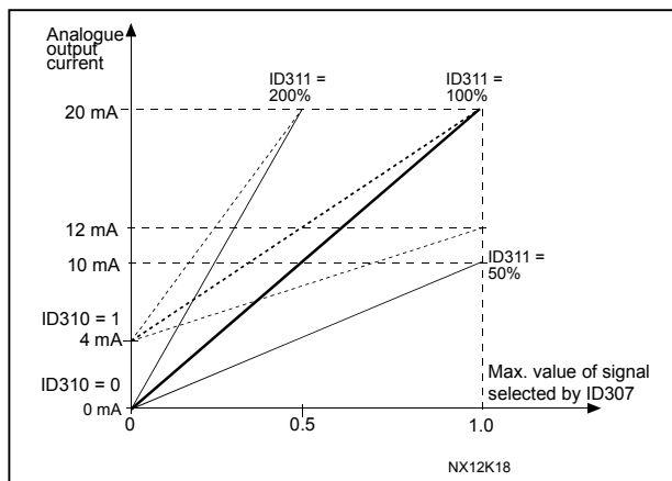
Σχήμα 8-15. Κλιμάκωση αναλογικής εξόδου
