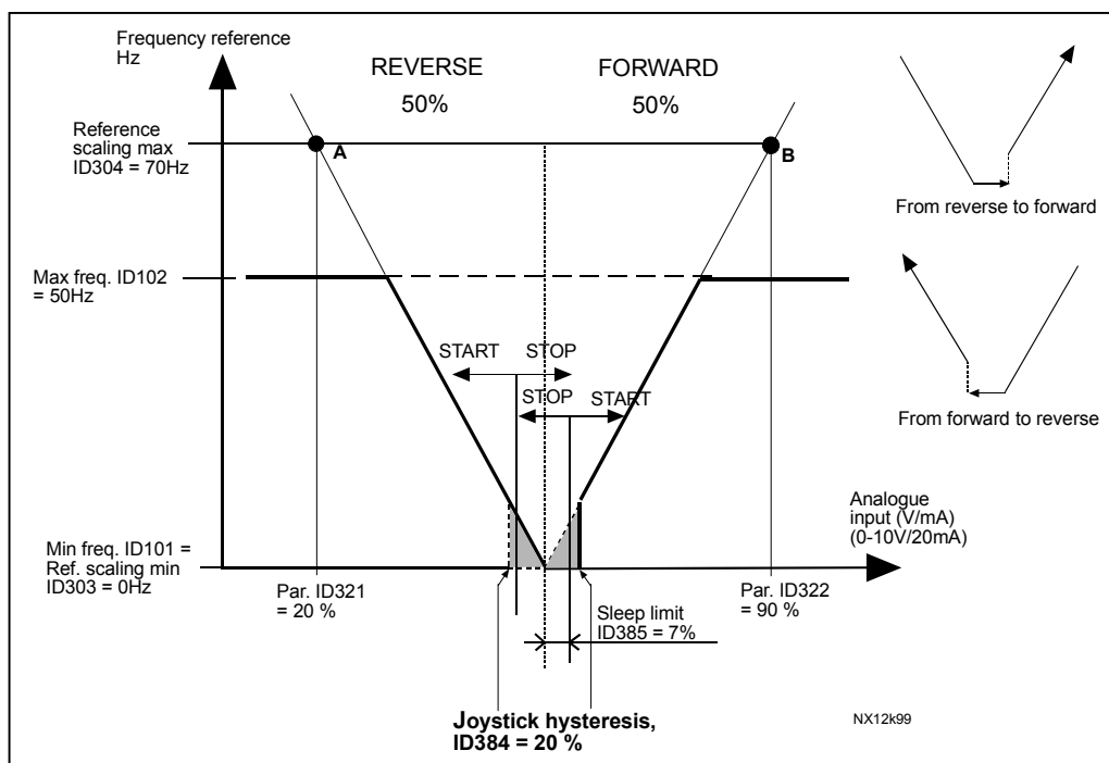
Σχήμα 8-35. Παράδειγμα της λειτουργίας του ορίου υπολειτουργίας της μονάδας
