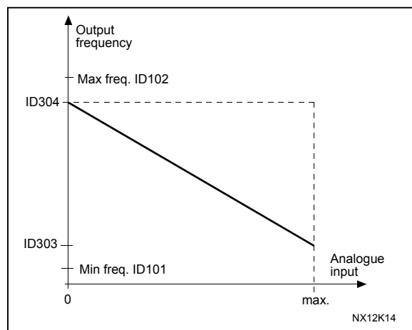
Σχήμα 8-11. Αναστροφή αναφοράς.
