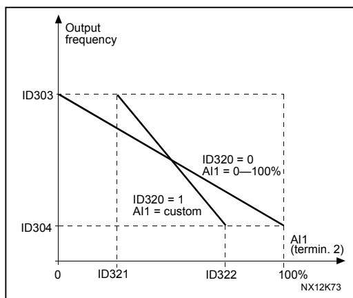
Σχήμα 8-19. AI1 αναστροφή σήματος
