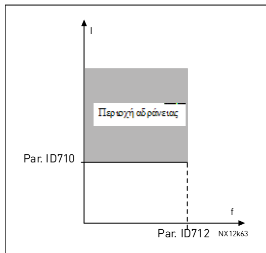
Σχήμα 8-50. Ρυθμίσεις χαρακτηριστικών αδράνειας
