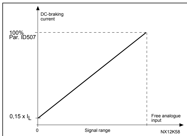
Σχήμα 8-37. Κλιμάκωση της έντασης του DC-φρένου
