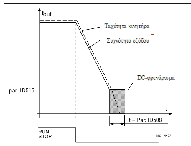
Σχήμα 8-44. Χρόνος DC-φρεναρίσματος όταν ο τρόπος Στάσης = Ράμπα
