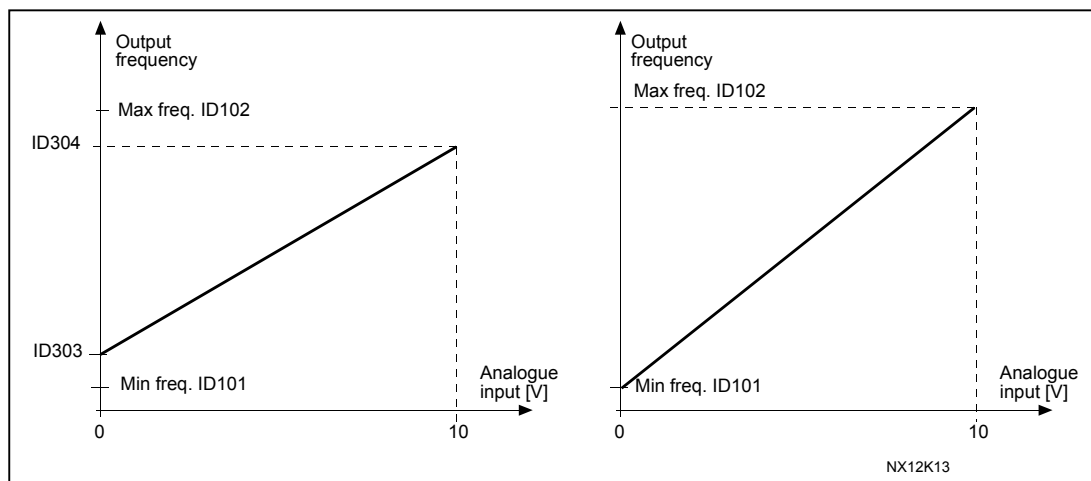
Σχήμα 8-10. Αριστερά: Κλιμάκωση αναφοράς. Δεξιά: Δεν χρησιμοποιείται κλιμάκωση (παρ. ID303 = 0).
