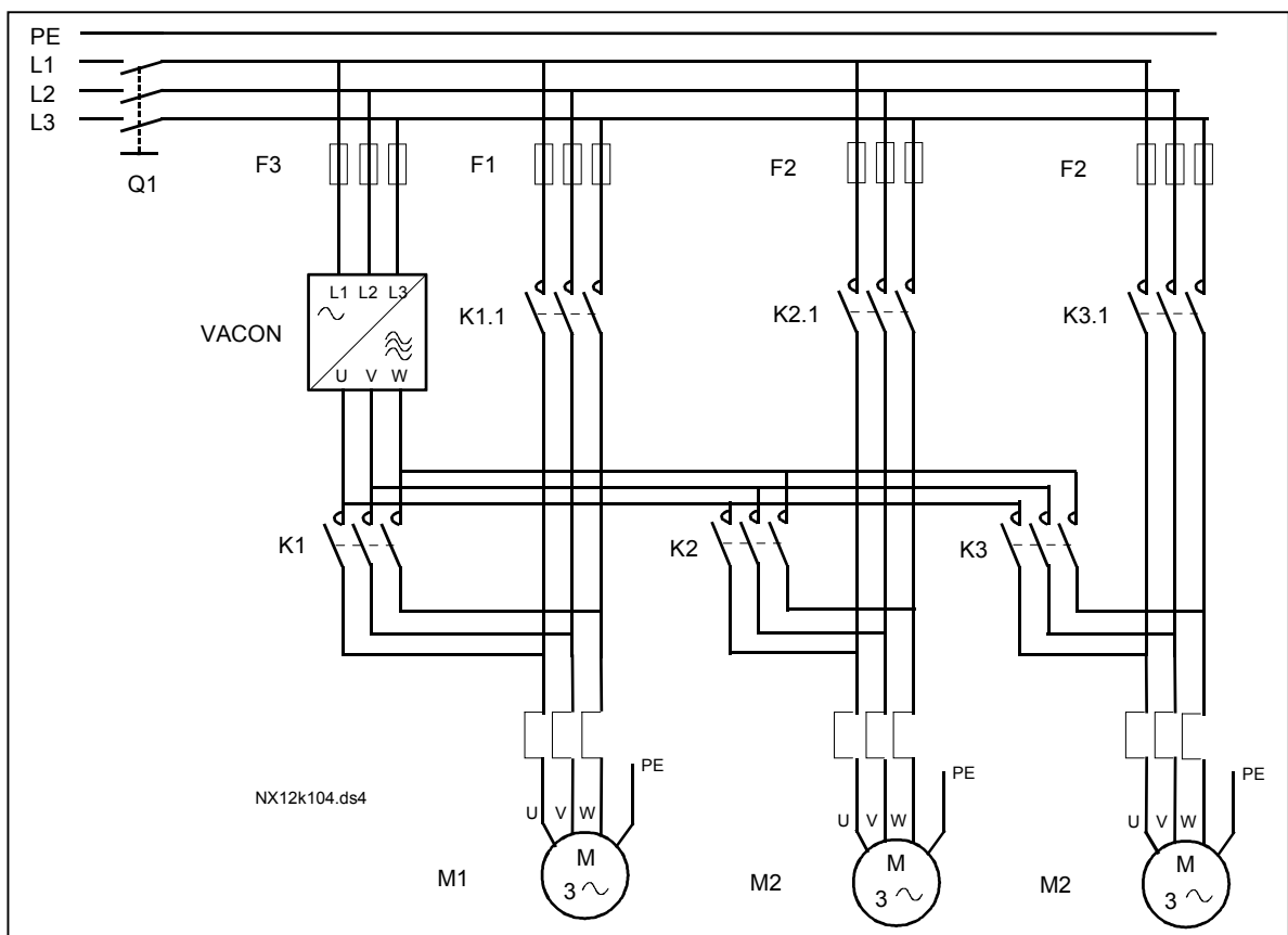
Σχήμα 7-6. Παράδειγμα αυτοαλλαγής 3-αντλιών, κύριο διάγραμμα
