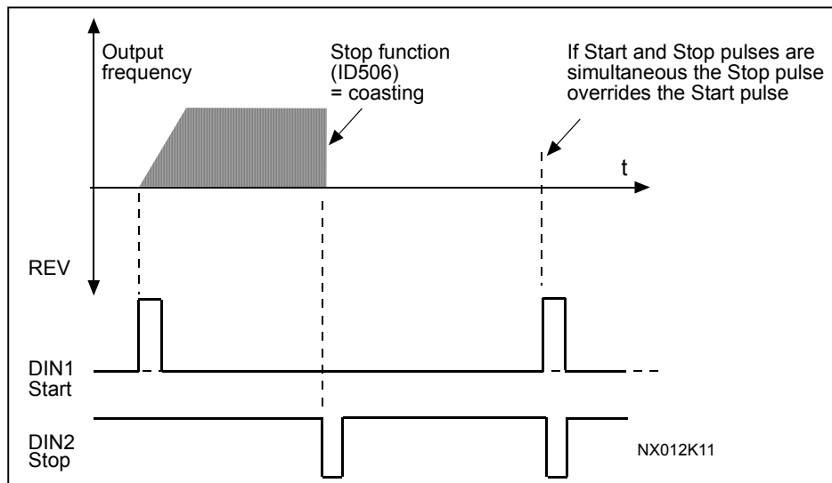
Σχήμα 8-8. Παλμός εκκίνησης / Παλμός στάσης.
