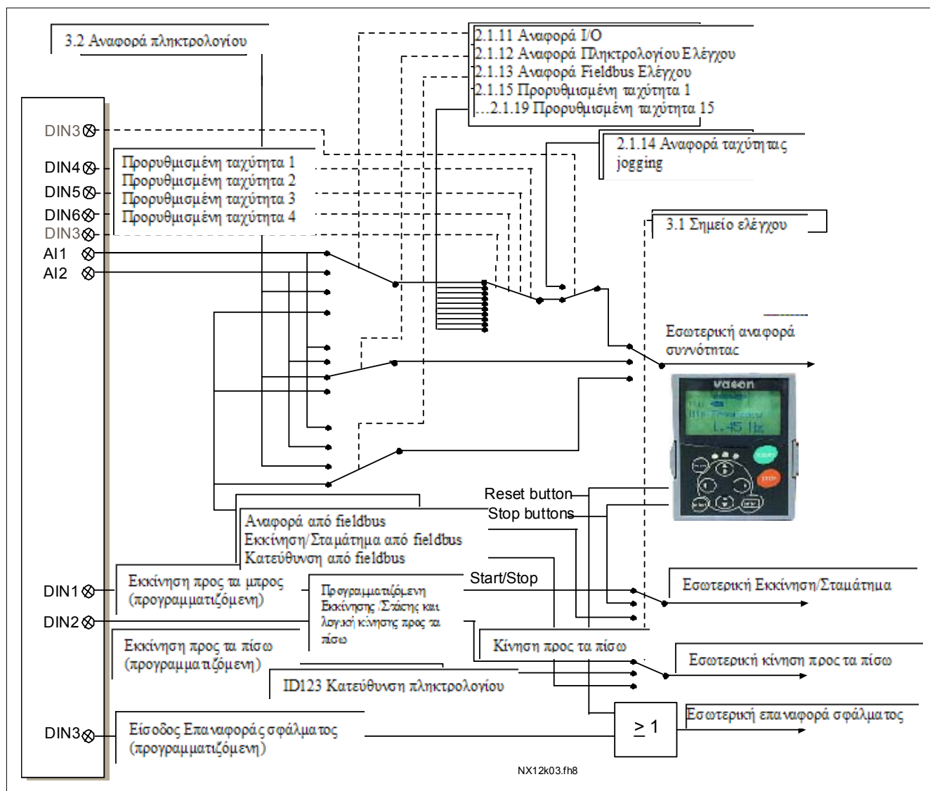
Σχήμα 4-1. Λογική σήματος ελέγχου της Εφαρμογής Πολύ-Βηματικού Ελέγχου Ταχύτητας
