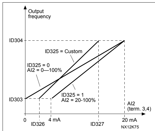
Σχήμα 8-21. Κλιμάκωση της αναλογικής εισόδου AI2.
