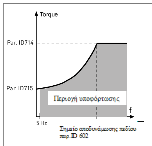
Σχήμα 8-52. Ρύθμιση ελάχιστου φορτίου
