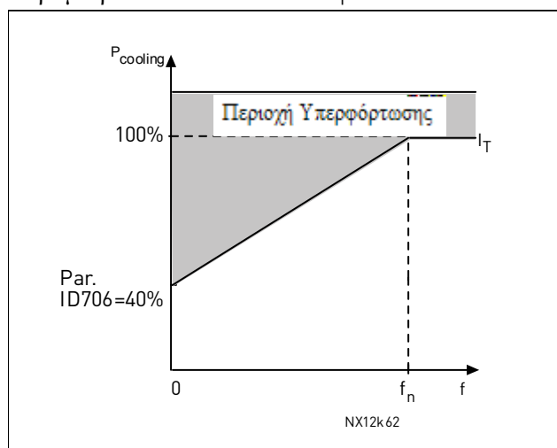
Σχήμα 8-47. Καμπύλη θερμικής έντασης I_T κινητήρα
