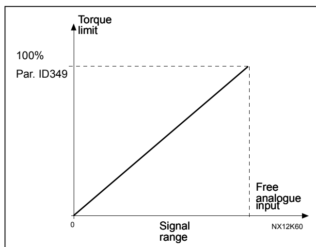
Σχήμα 8-39. Μείωση ορίου επίβλεψης ροπής
