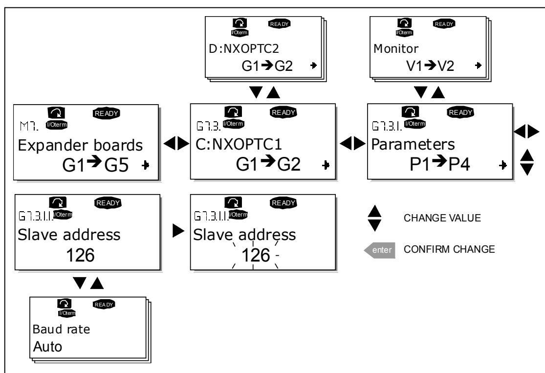
Rysunek 68. Menu kart WE/WY (M7).
