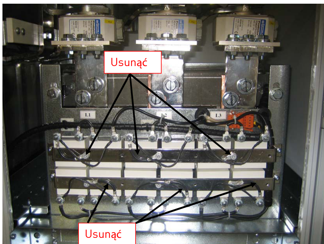
Rysunek 13. Kondensatory HF filtra LCL w przetwornicy NXC regeneratywnej o niskiej zawartości harmonicznych, wielkości FI13 FI14.
