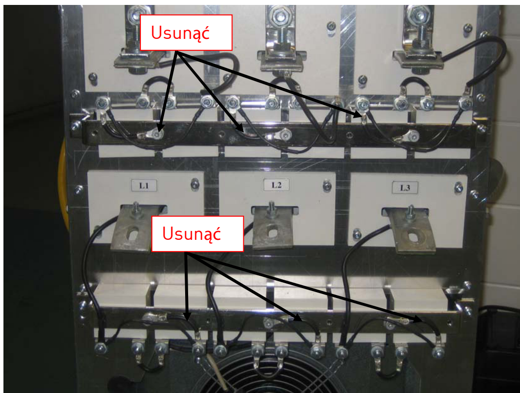
Rysunek 12. Kondensatory HF filtra LCL w przetwornicy NXC regeneratywnej o niskiej zawartości harmonicznych, wielkości FI9, FI10 i FI12.
