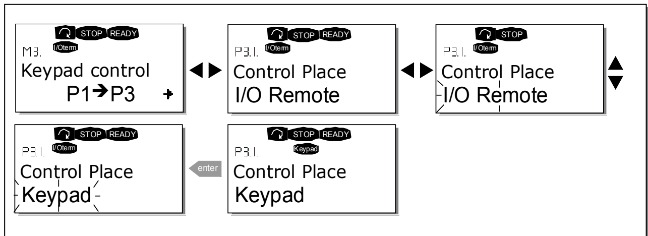
Rysunek 47. Wybór miejsca sterowania napędu.
