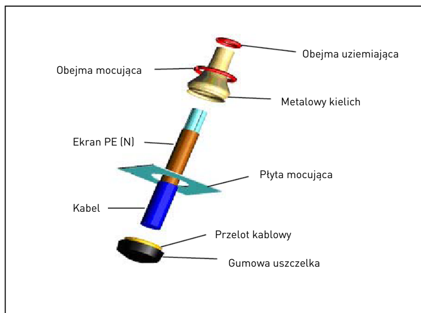
Rysunek 23. Elementy dławika kablowego.
