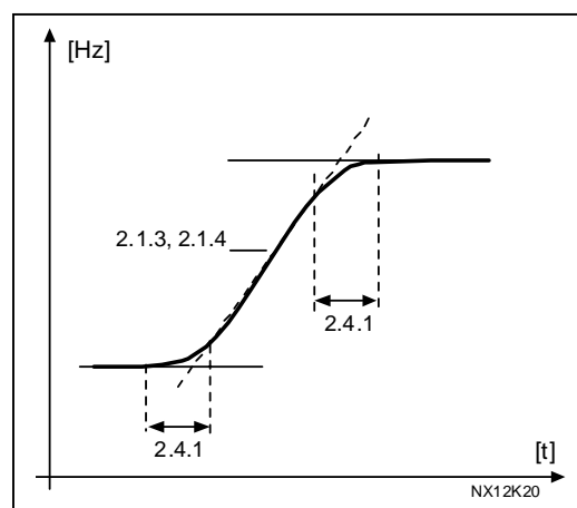
Figura 1- 9. Supervisione frequenza di uscita
