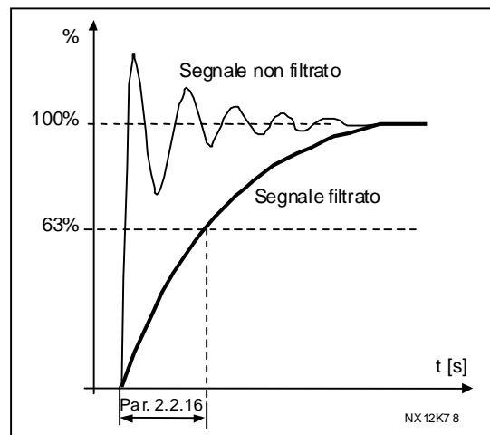
Figura 1- 4. Filtraggio segnale AI2 ( I_{in} )
