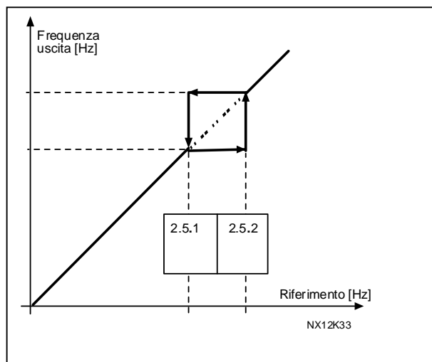
Figura 1- 15. Impostazione area di frequenza proibita.
