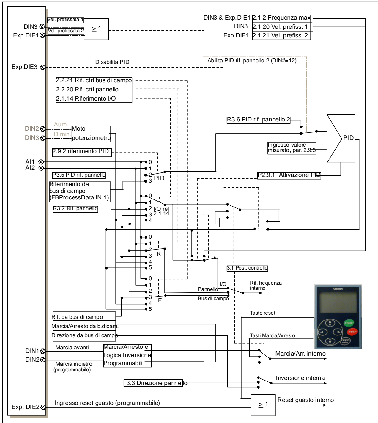
Figura 1- 39. Logica dei segnali di controllo nell'applicazione MultiControllo
