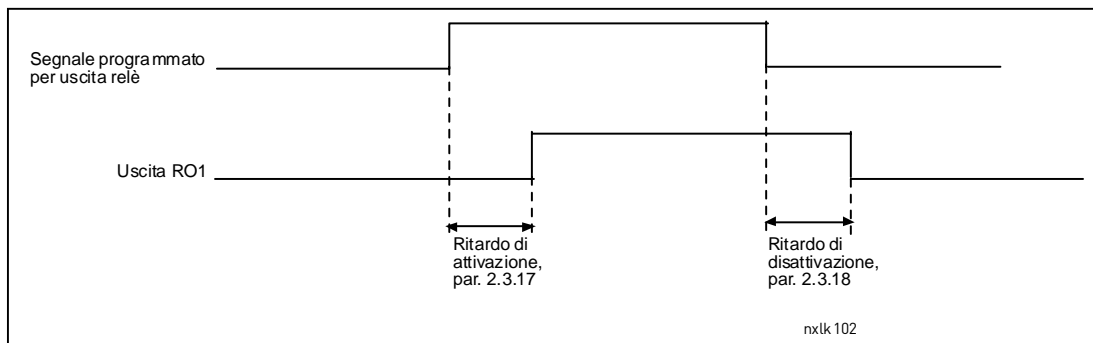
Figura 1- 10. Ritardi di attivazione e disattivazione uscita relè 1
