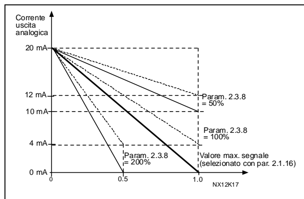
Figura 1- 7. Inversione uscita analogica
