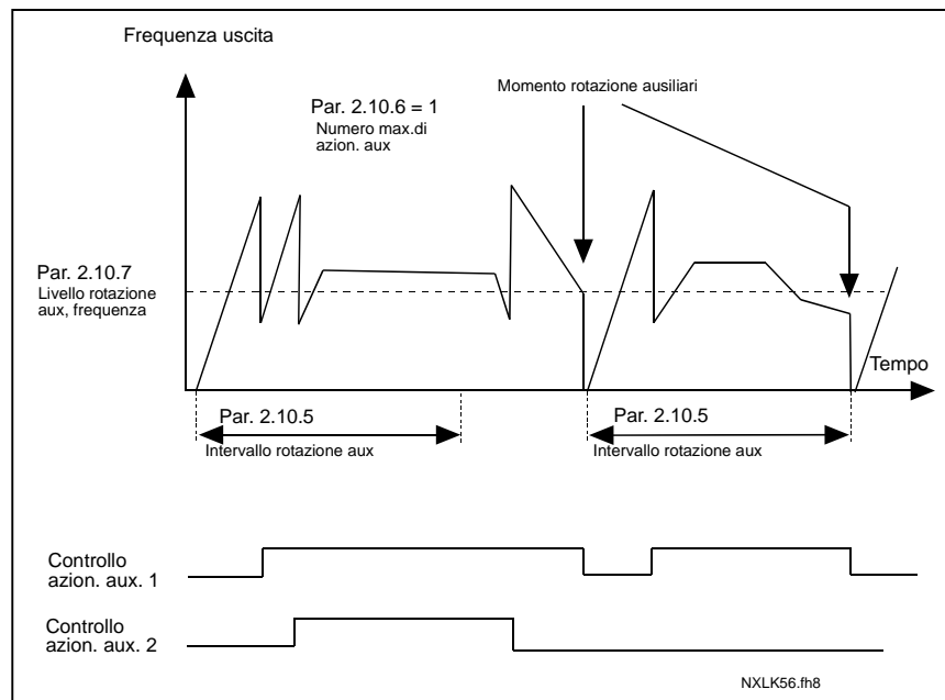
Figura 1- 38. Intervallo e limiti della rotazione degli ausiliari
