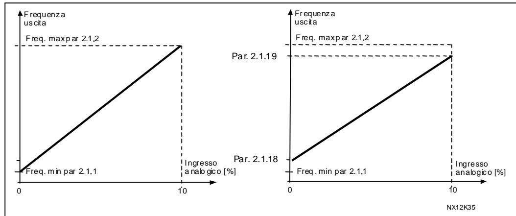
Figura 1- 5. Sinistra: Par. 2.1.18=0 (Nessuna scalatura di riferimento) Destra: Scalatura di riferimento.
