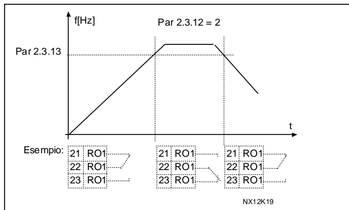
Figura 1- 11. Accelerazione/Decelerazione (a S)
