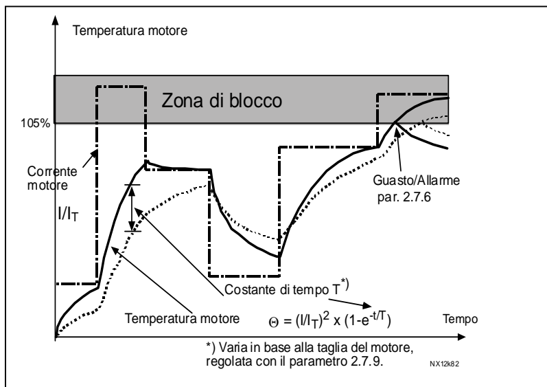
Figura 1- 20. Calcolo temperatura motore
