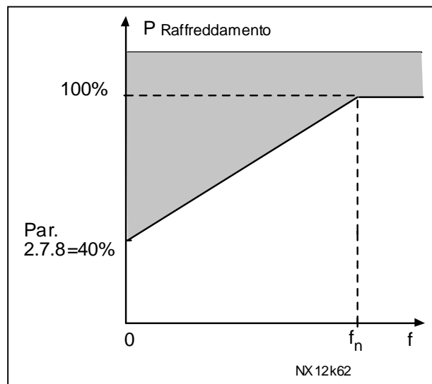
Figura 1- 19. Capacità di raffreddamento del motore
