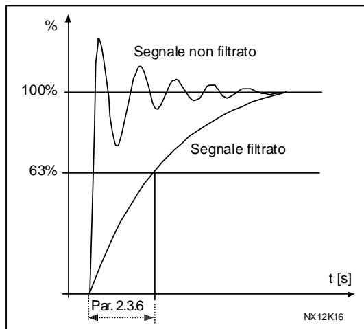
Figura 1- 6. Filtraggio uscita analogica
