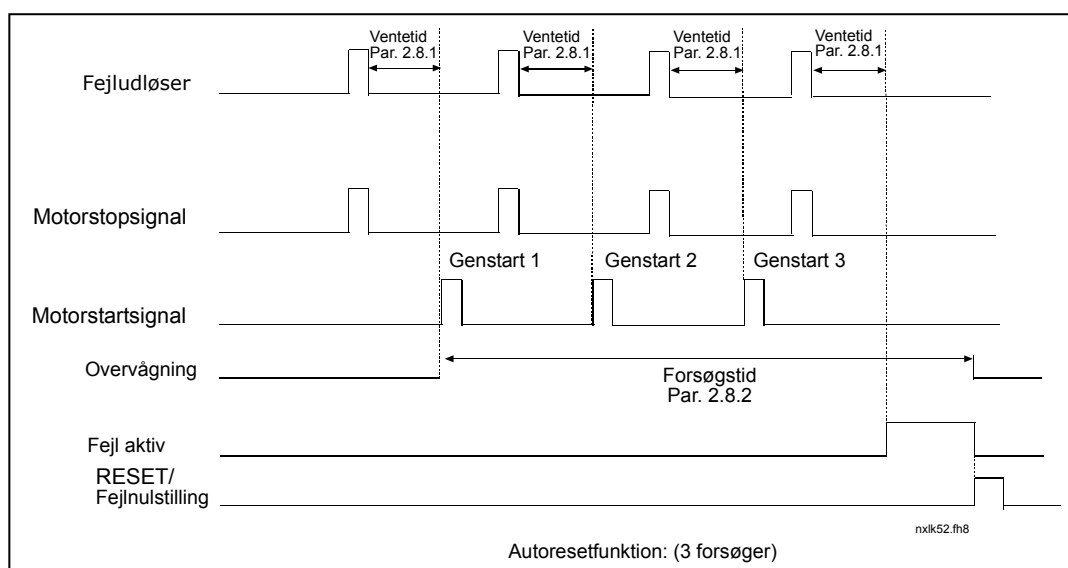
Figur 1- 24. Automatisk genstart
