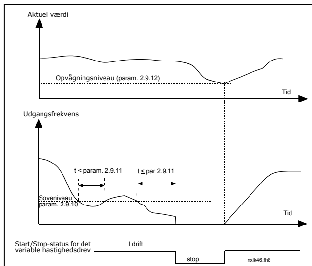
Figur 1-29. Frekvensomformerens sovefunktion
