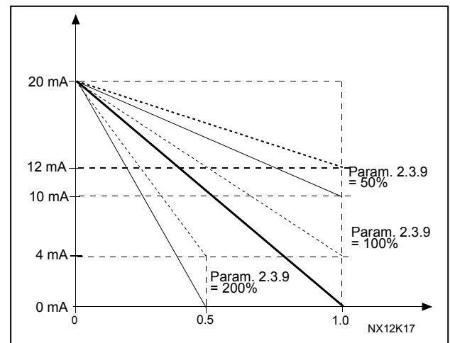
Figur 1-6. Invertering af analog udgang
