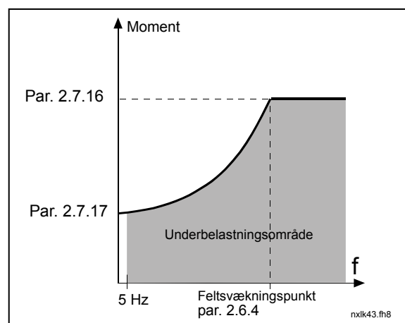
Figur 1-22. Indstilling af minimumsbelastningen
