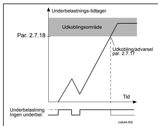
Figur 1-23. Tidtagning af underbelastning
