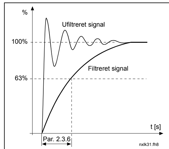
Figur 1-5. Filtrering af analog udgang
