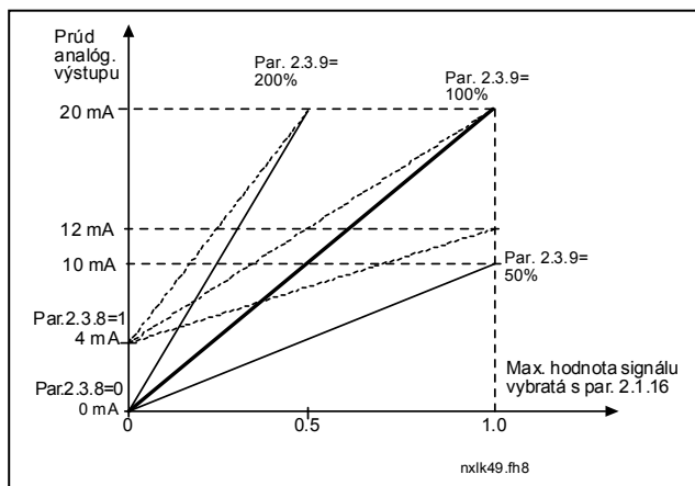
Obr. 1-7. Zmena mierky analóg. výstupu
