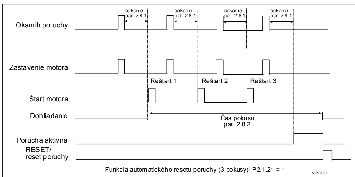
Obr. 1-24. Automatický reštart.
