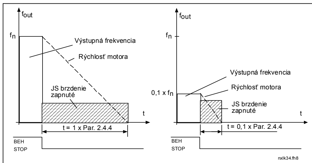
Obr. 1-11. Čas JS brzdienia, keď spôsob zastavenia = voľný dobeh.
