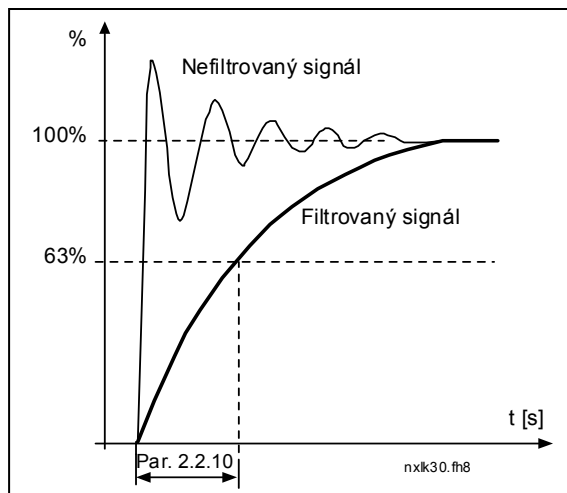
Obr. 1-3. Filtrovanie signálu AI1
