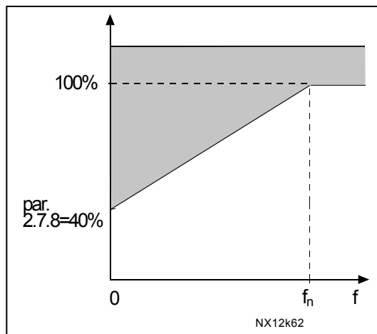
Obr. 1-18. Výkon chladenia motora
