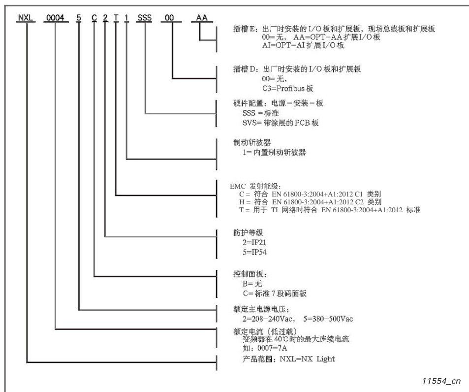
图 3-2. Vacon NXL 型号标识码 (MF4 - MF6)
