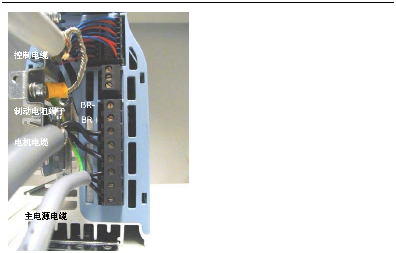
图 6-9. MF3 变频器的电缆安装
