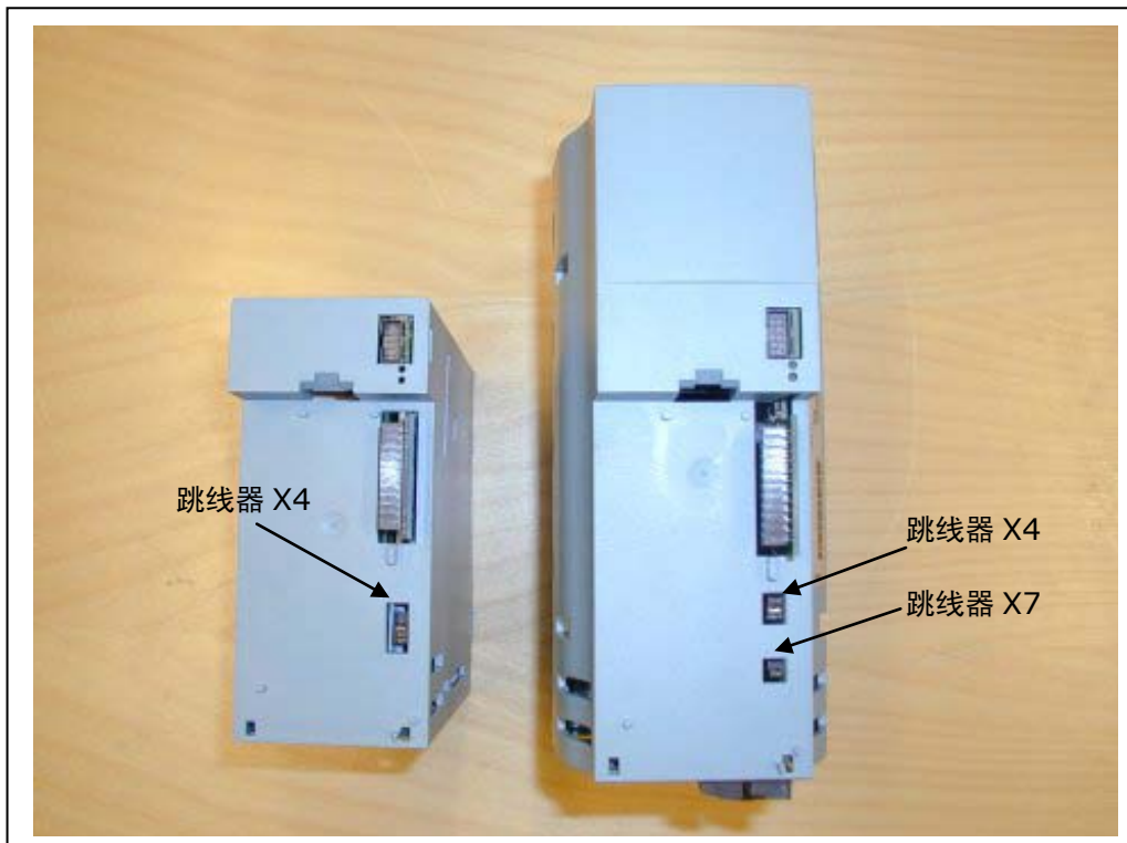
图 6-25. MF2(左)和 MF3(右)变频器的跳线器位置
