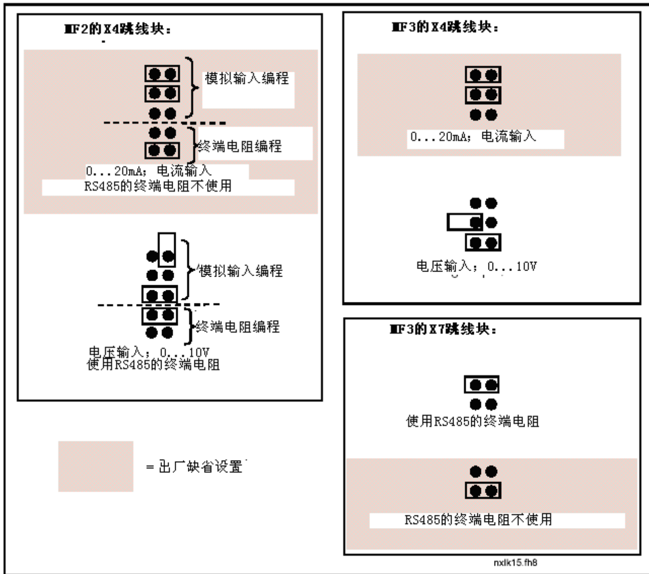
图 6-23. Vacon NXL 变频器的跳线选择, MF2 和 MF3
