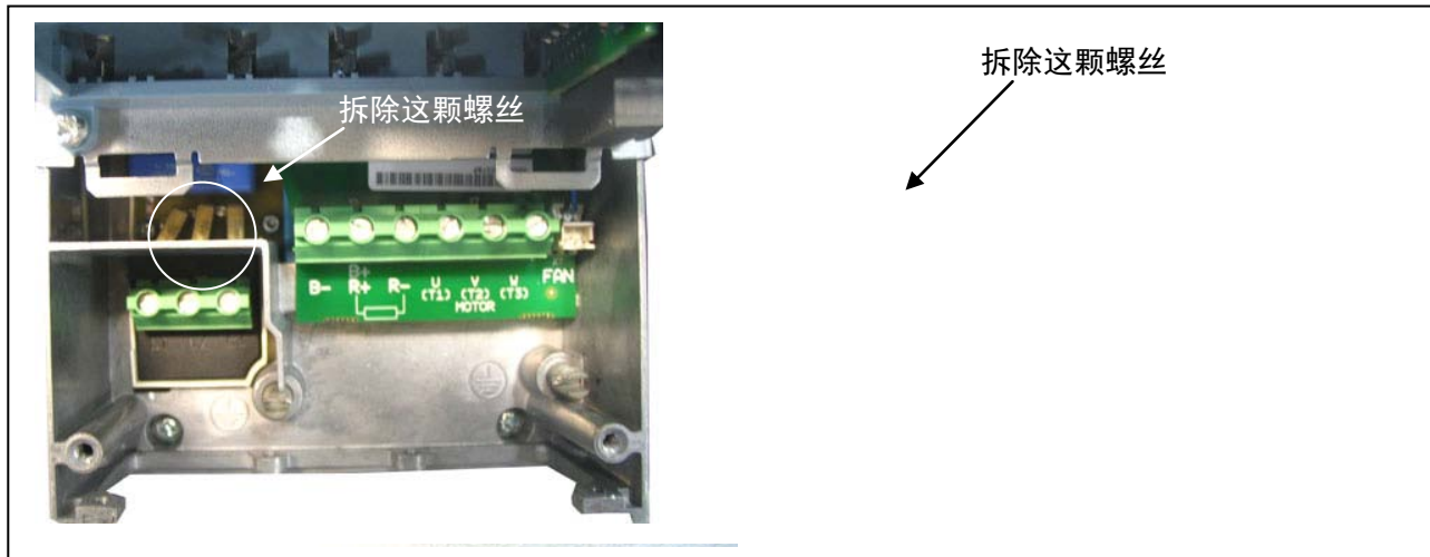
图 5-7. 改变 EMC 防护等级，MF4(左)和 MF5(右)
