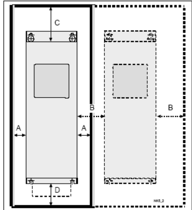
图 5-6. 安装空间
