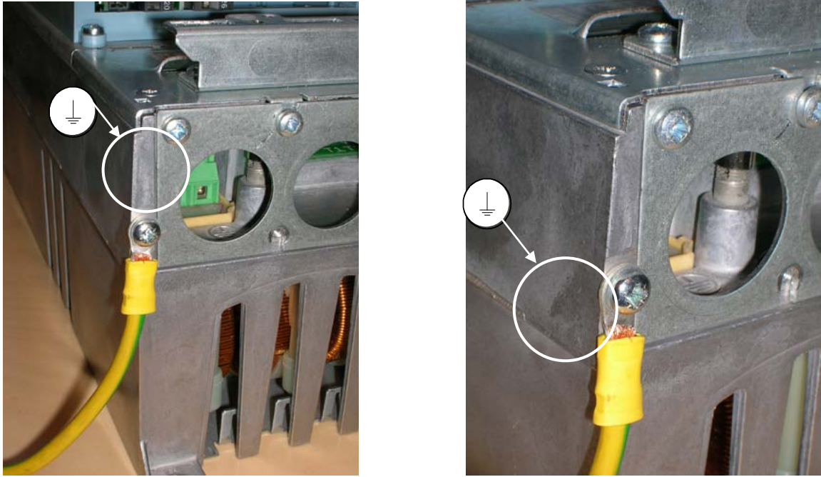
图 6-15. 附加接地电缆的连接, MF4。请参见第 1.3 章
