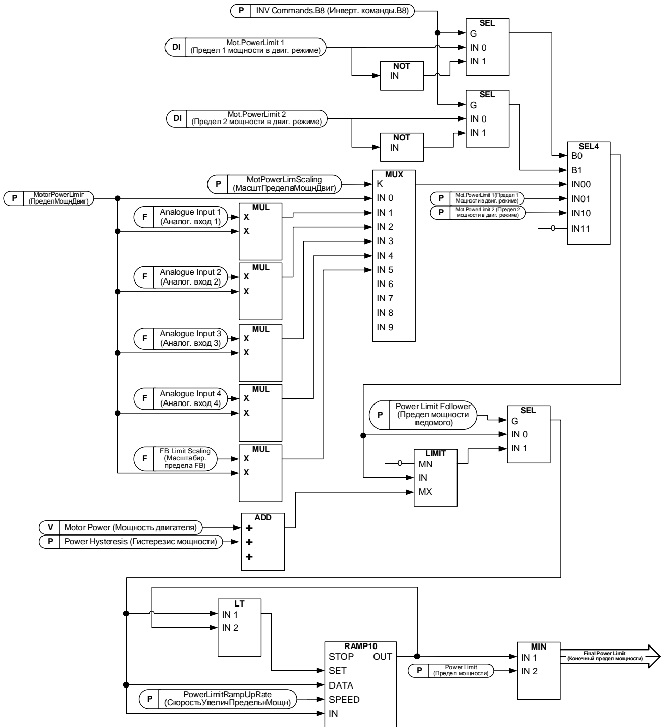
Управление изменением скорости посредством ограничения мощности
