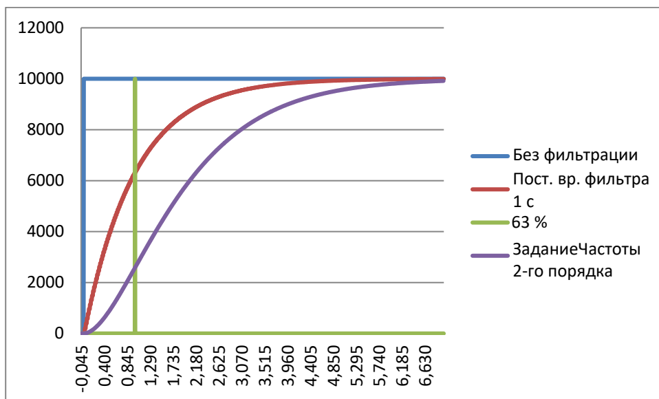
Рис. 7-10. Фильтрация сигнала A11
