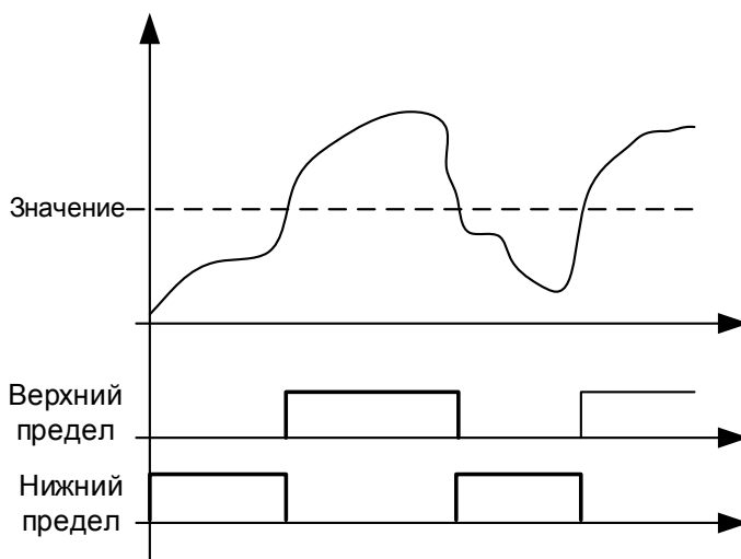
Рис. 7-12. Функция контроля
