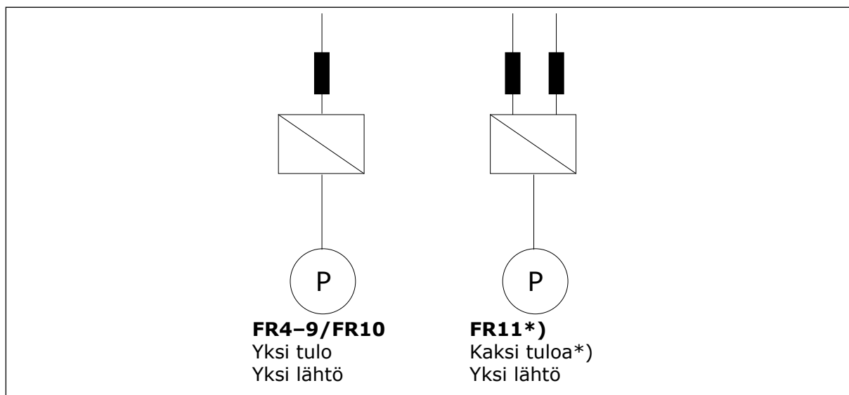
Kuva 19: Kokoluokkien FR4–FR11 topologia
