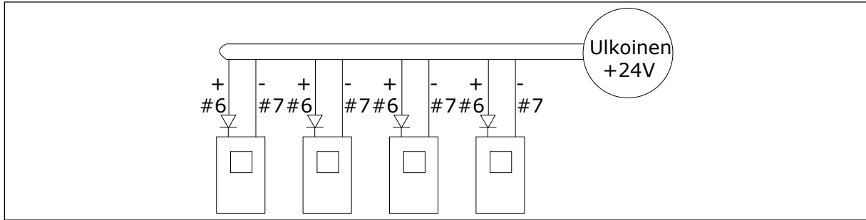
Kuva 21: Useiden taajuusmuuttajien 24 V:n rinnankytkentä
