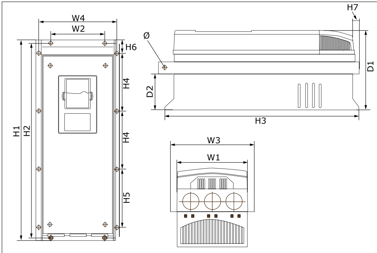
Kuva 10: Kauluksella varustettujen NXS- ja NXP-taajuusmuuttajien mitat, FR7 ja FR8
