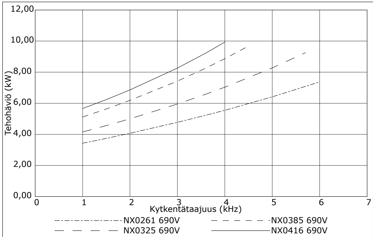
Kuva 46: Tehohäviö kytentätaajuuden funktiona; NXS tai NXP 0261-0416
