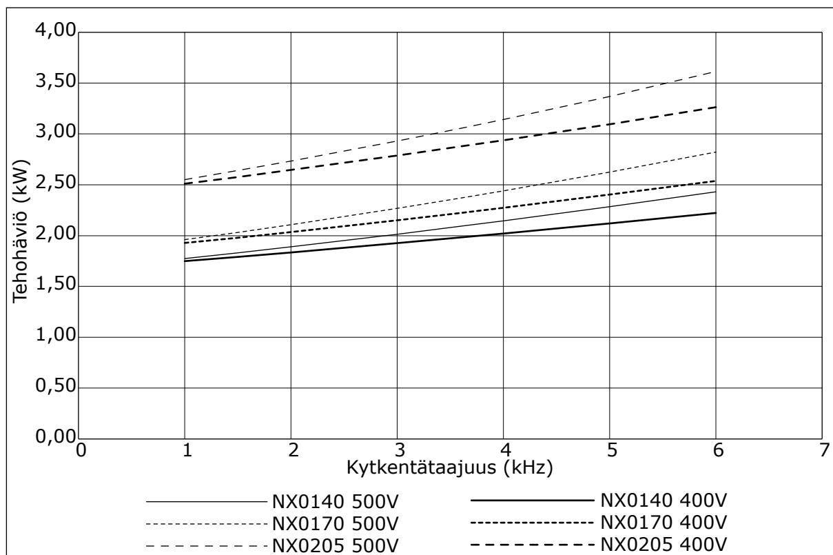
Kuva 38: Tehohäviö kytentätaajuuden funktiona; NXS tai NXP 0140–0205
