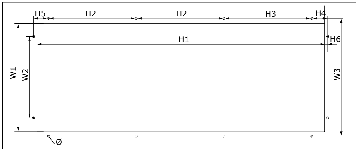
Kuva 11: Aukon ja kauluksella varustetun taajuusmuuttajan ulkokuoren mitat, FR7
