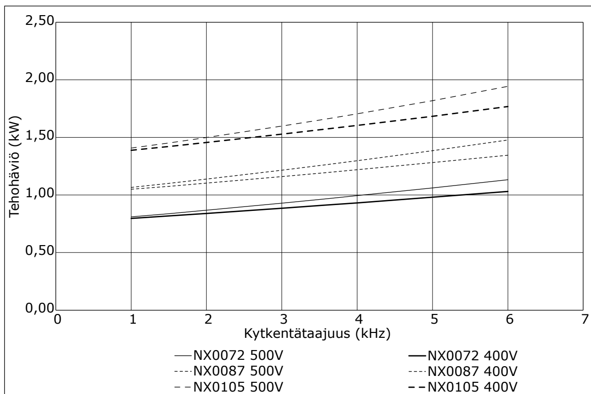
Kuva 37: Tehohäviö kytentätaajuuden funktiona; NXS tai NXP 0072–0105
