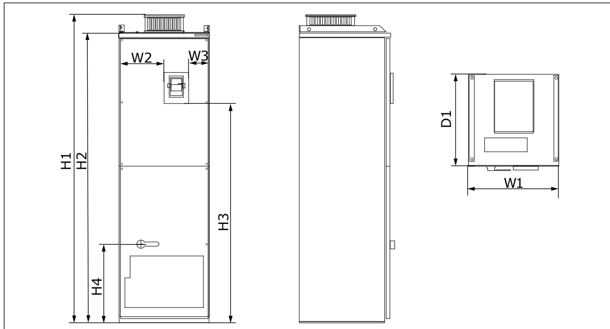
Kuva 14: NXS- ja NXP-taajuusmuuttajien mitat, FR10 ja FR11
