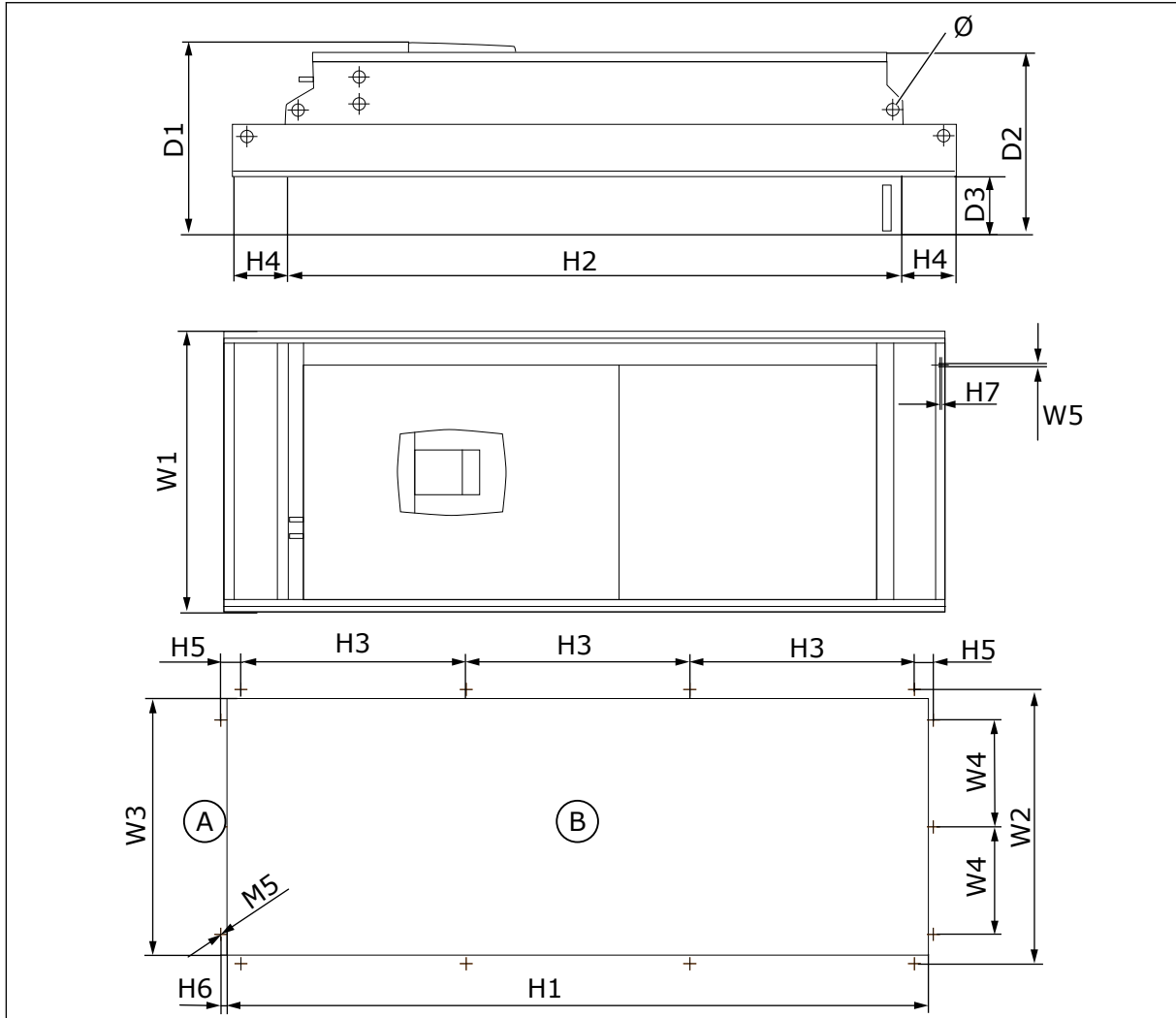
Kuva 13: NXS- ja NXP-taajuusmuuttajien mitat, F9
