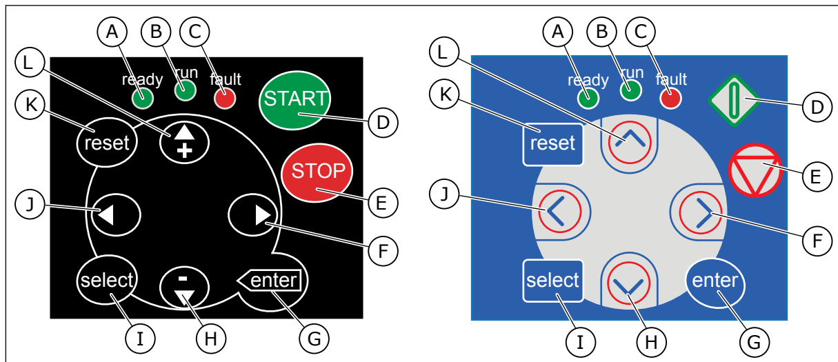
Kuva 28: Paneelin painikkeet, vasemmalla: NXS, oikea: NXP
