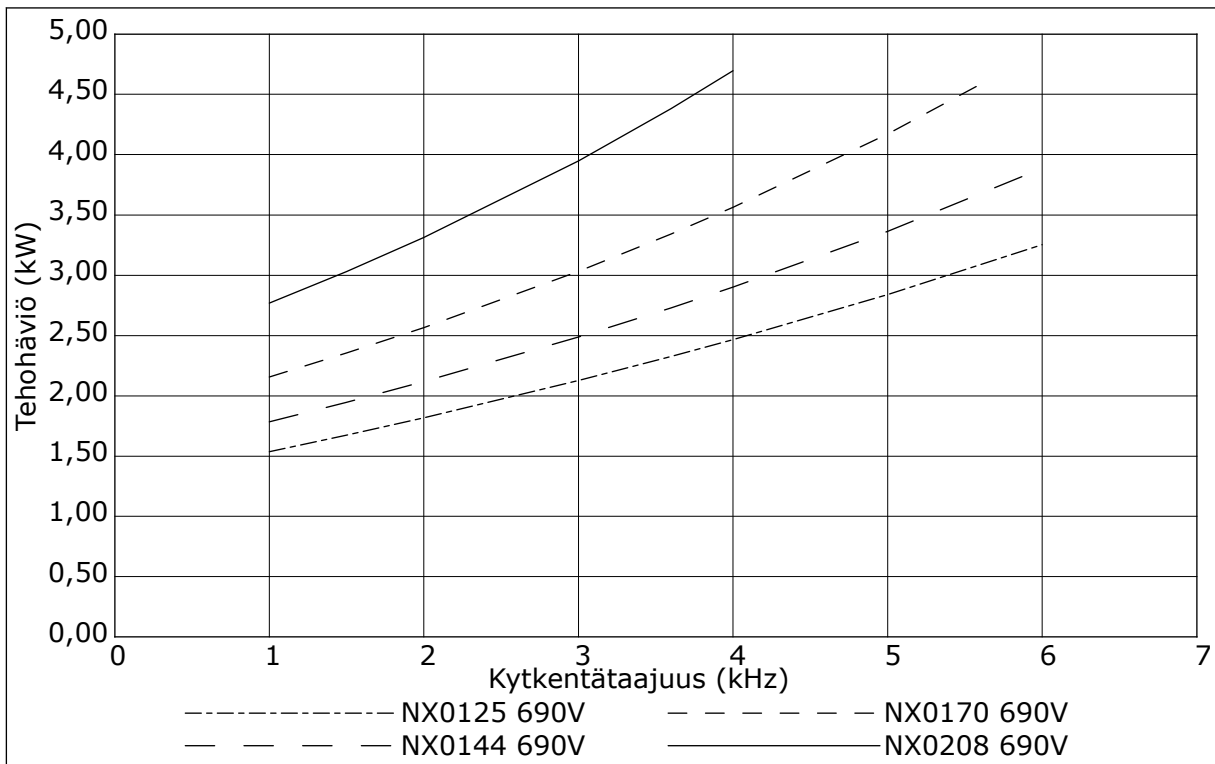
Kuva 45: Tehohäviö kytKentätaajuuden funktiona; NXS tai NXP 0125-0208
