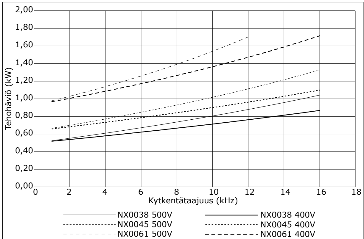
Kuva 36: Tehohäviö kytentätaajuuden funktiona; NXS tai NXP 0038-0061
