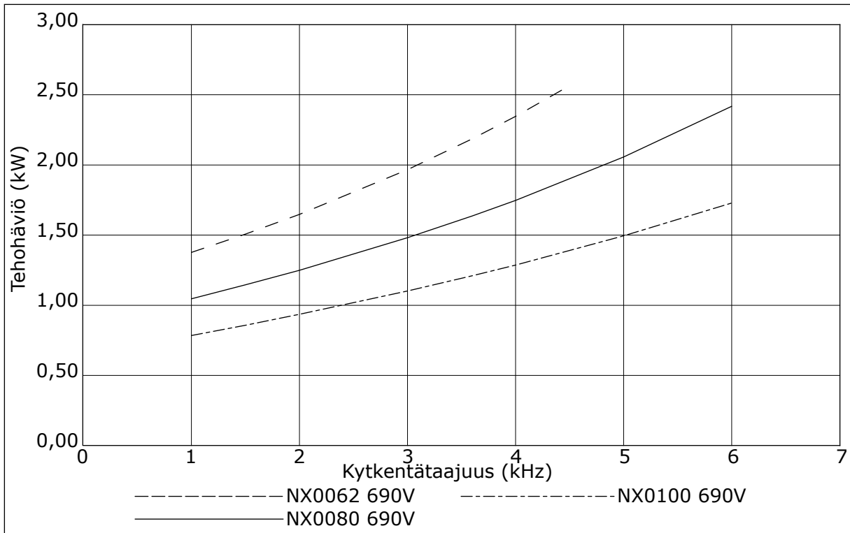
Kuva 44: Tehohäviö kytKentätaajuuden funktiona; NXS tai NXP 0062-0100
