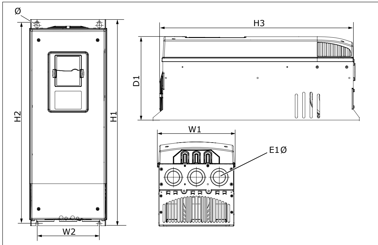
Kuva 5: NXS- ja NXP-taajuusmuuttajien mitat, FR7
