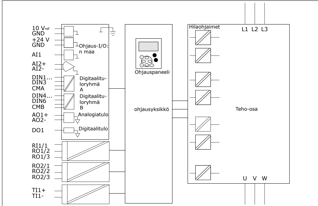
Kuva 27: Galvaaniset erottimet
