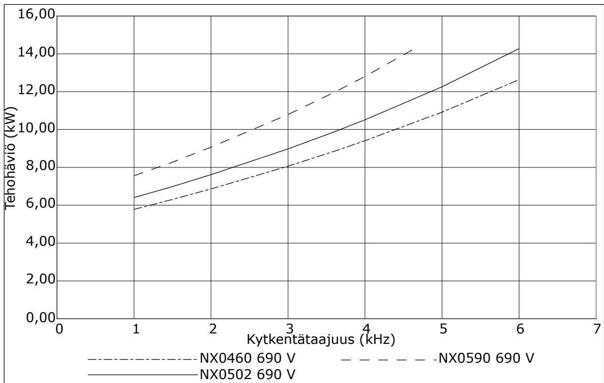
Kuva 47: Tehohäviö kytentätaajuuden funktiona; NXS tai NXP 0460-0590
