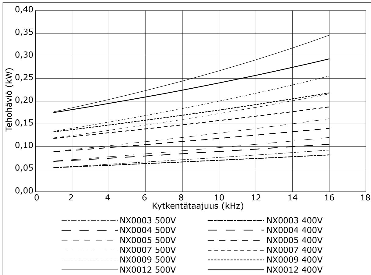
Kuva 34: Tehohäviö kytkentätaajuuden funktiona; NXS tai NXP 0003–0012
