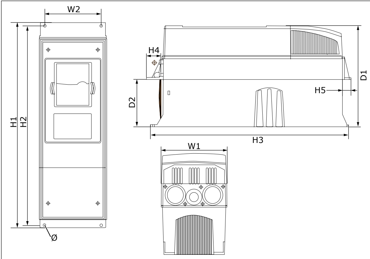
Kuva 8: Kauluksella varustettujen NXS- ja NXP-taajuusmuuttajien mitat, FR4-FR6
