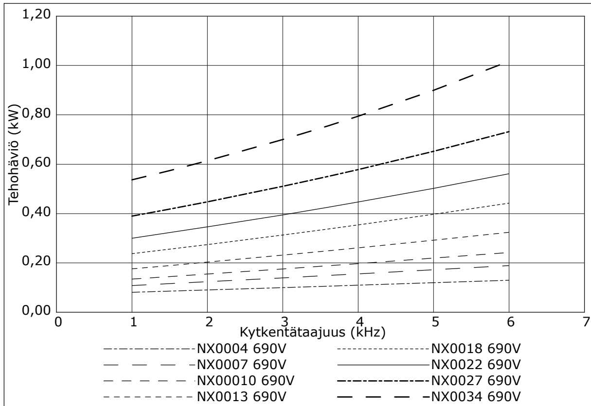
Kuva 42: Tehohäviö kytentätaajuuden funktiona; NXS tai NXP 0004–0034
