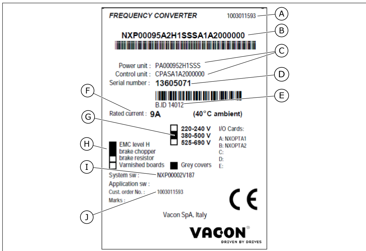
Kuva 1: Vacon-taajuusmuuttajien tavaraseloste
