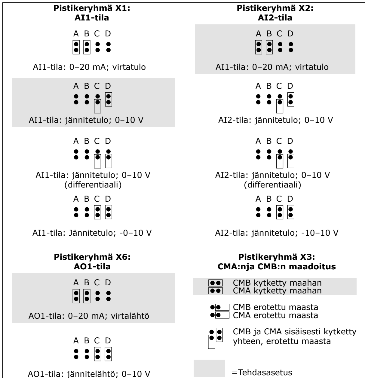
Kuva 26: OPTA1-kortin pistikevalinnat
