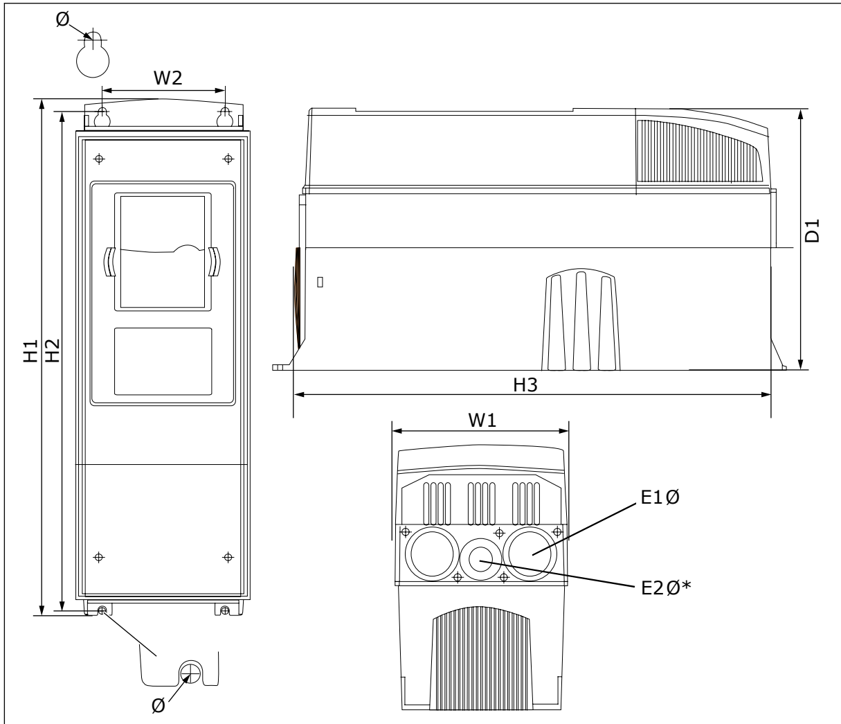
Kuva 4: NXS- ja NXP-taajuusmuuttajien mitat, FR4-FR6
