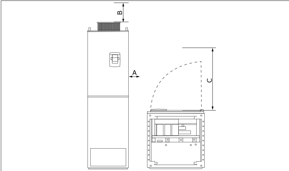
Kuva 16: Vähimmäisilmavälit taajuusmuuttajan ympärillä
