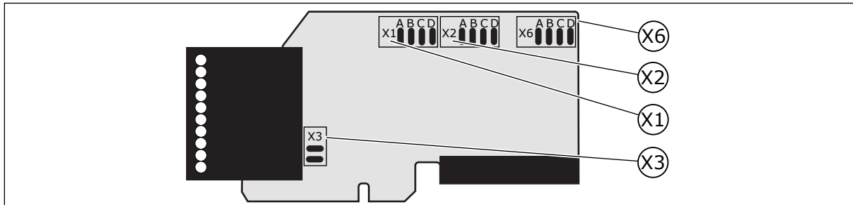
Kuva 25: OPTA1-kortin pistikeryhmät
