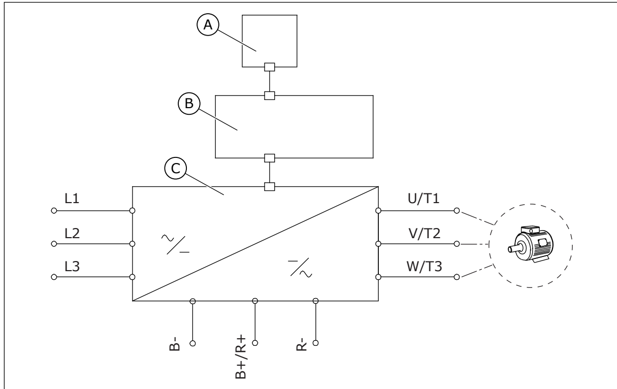
Kuva 17: Ensisijainen kytkentäkaavio
