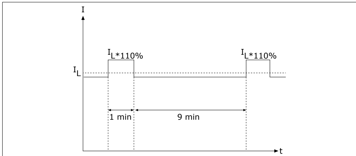
Kuva 32: Pieni ylikuormitus
