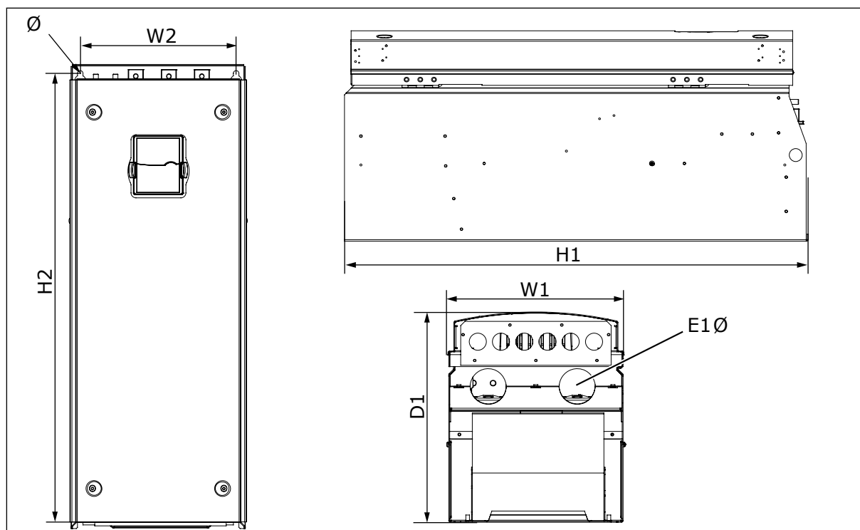
Kuva 6: NXS- ja NXP-taajuusmuuttajien mitat, FR8
