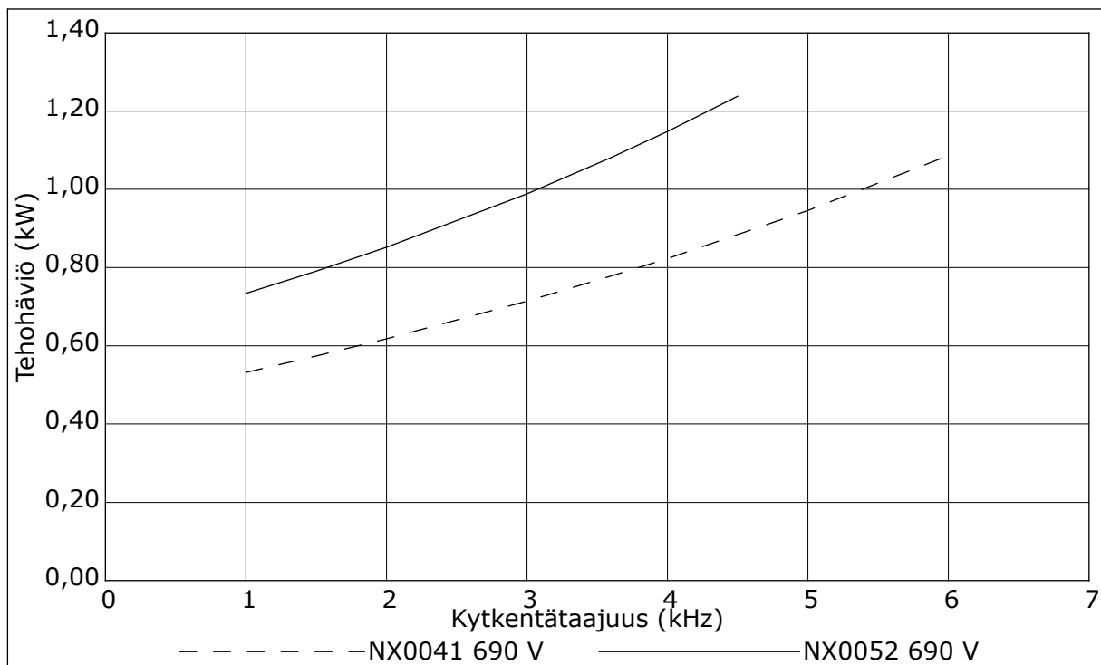
Kuva 43: Tehohäviö kytentätaajuuden funktiona; NXS tai NXP 0041–0052
