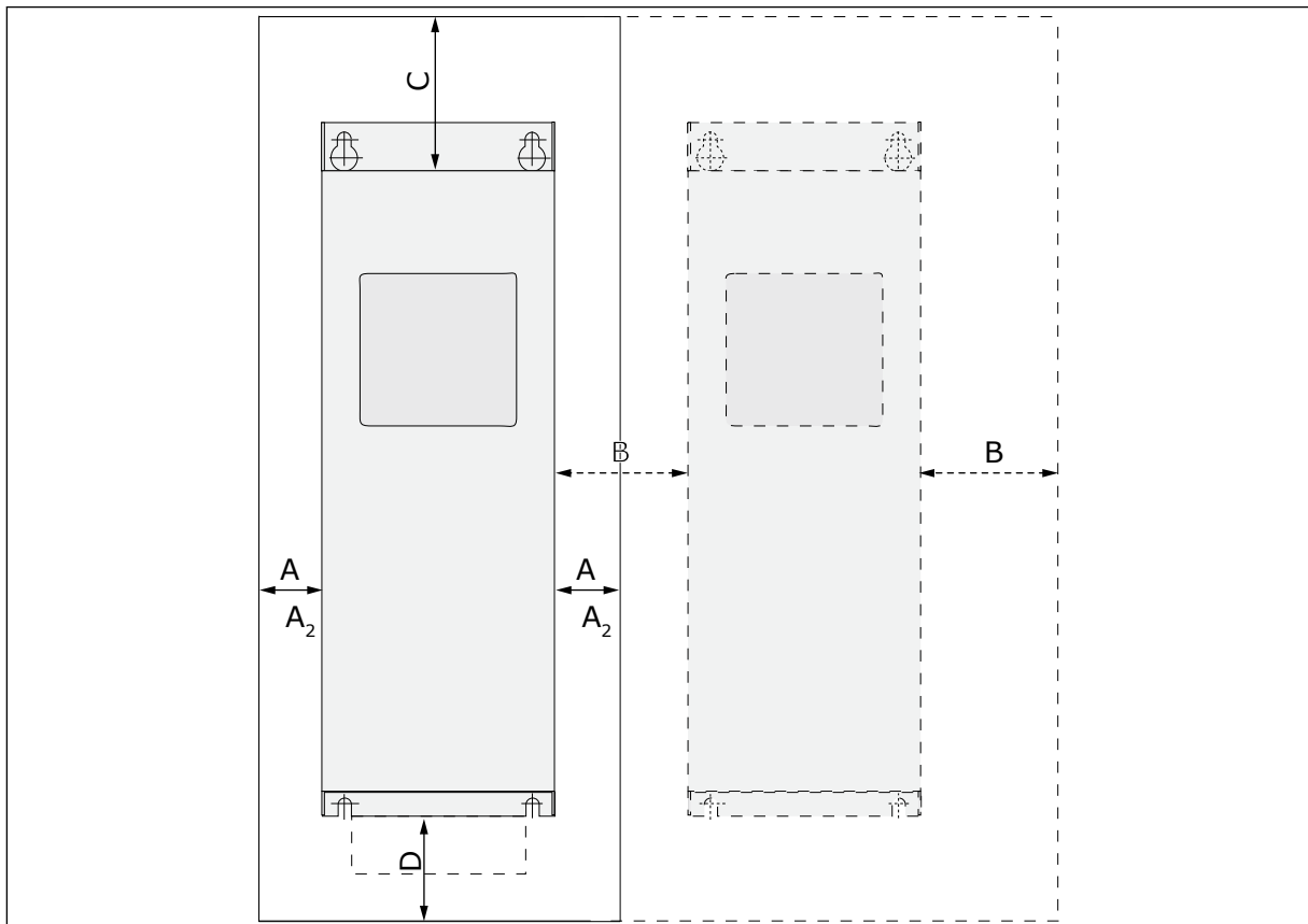
Kuva 15: Asennustila
