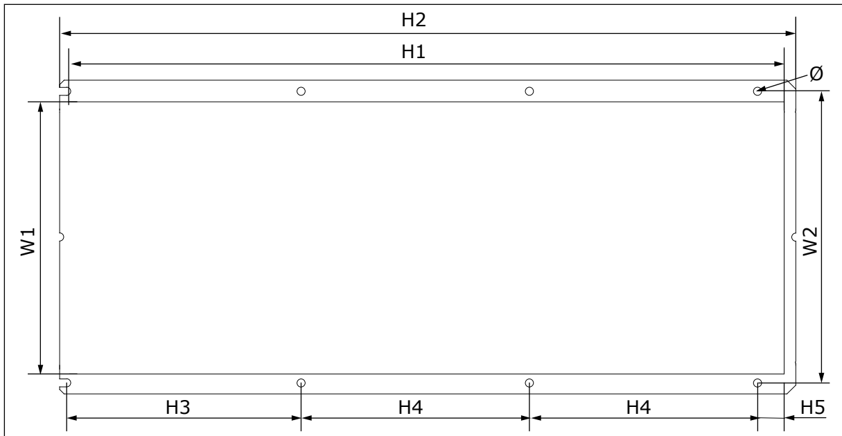
Kuva 12: Aukon ja kauluksella varustetun taajuusmuuttajan ulkokuoren mitat, FR8
