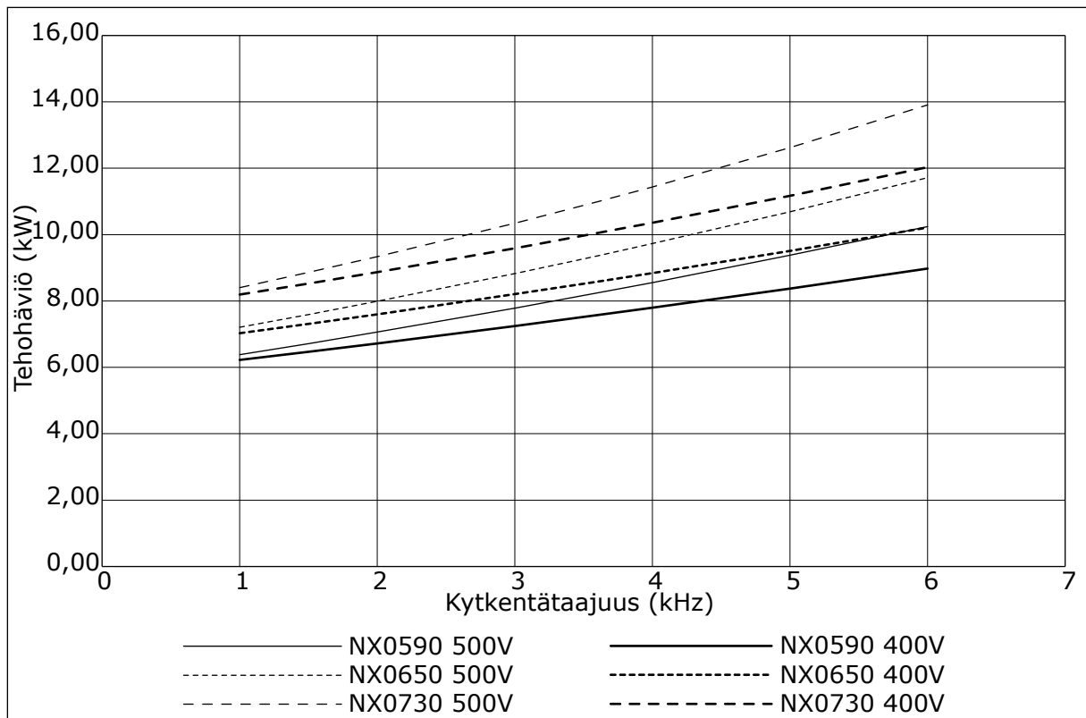
Kuva 41: Tehohäviö kytentätaajuuden funktiona; NXS tai NXP 0590–0730
