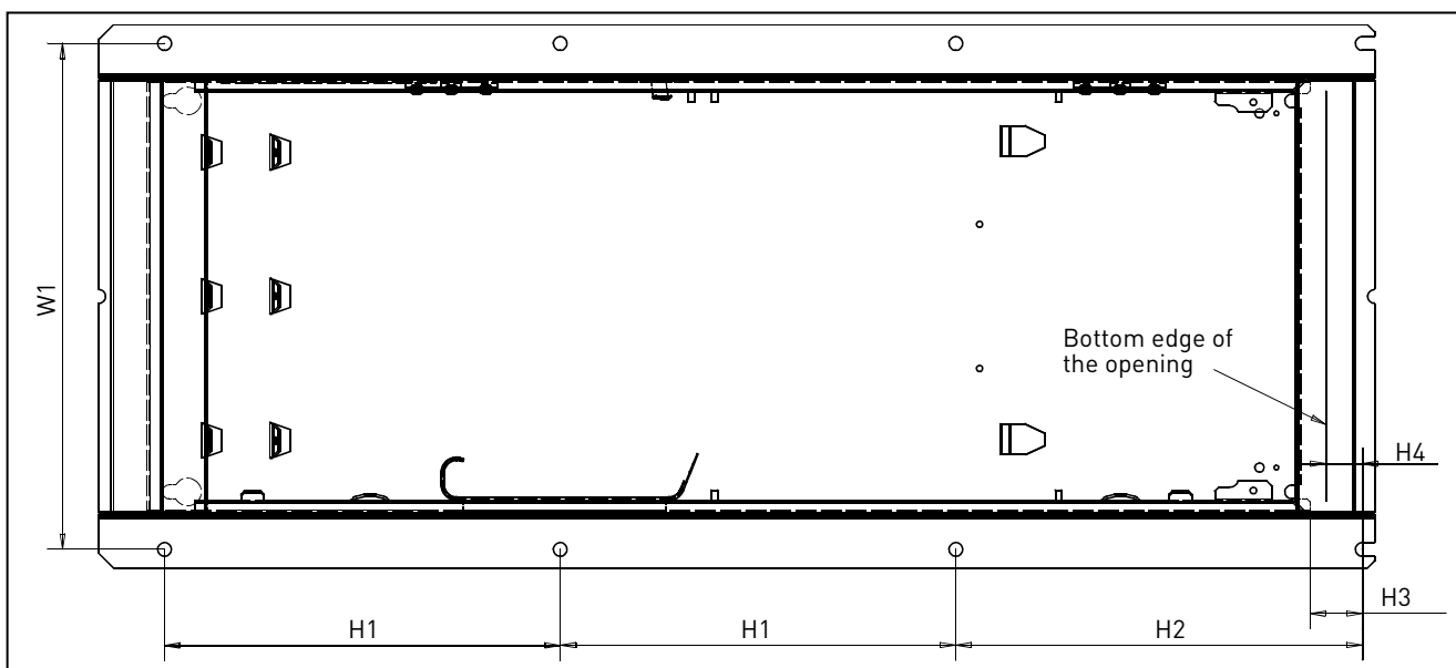
Obr. 5-6. Otvor potrebný pre prírubovú montáž, FR8
