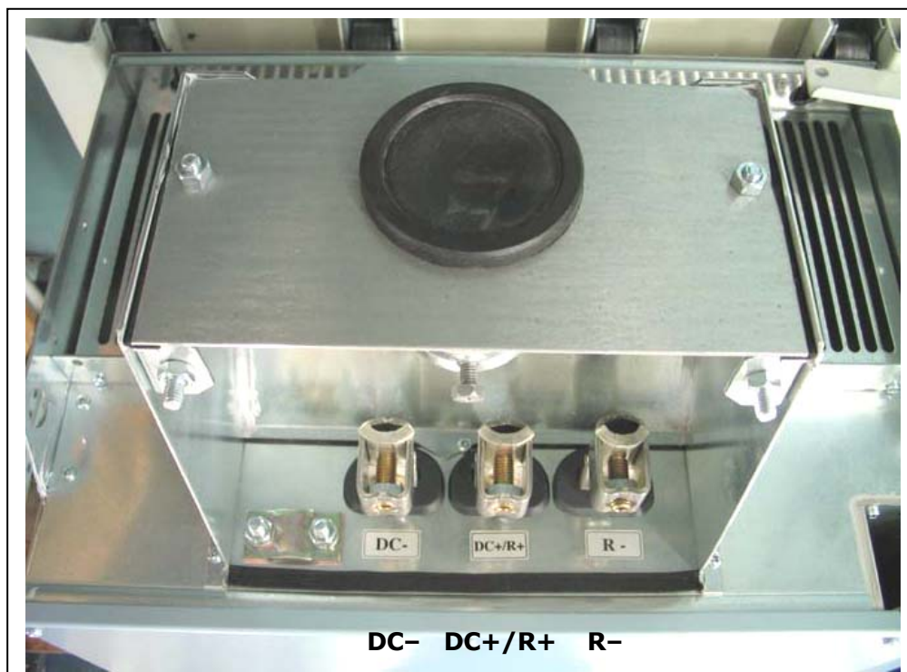
Obr. 6-20. Svorky JS medziobvodu a brzdného odporu pre FR9; Svorky JS medziobvodu sú označené DC- a DC+, svorky brzdného odporu sú označené R+ a R-
