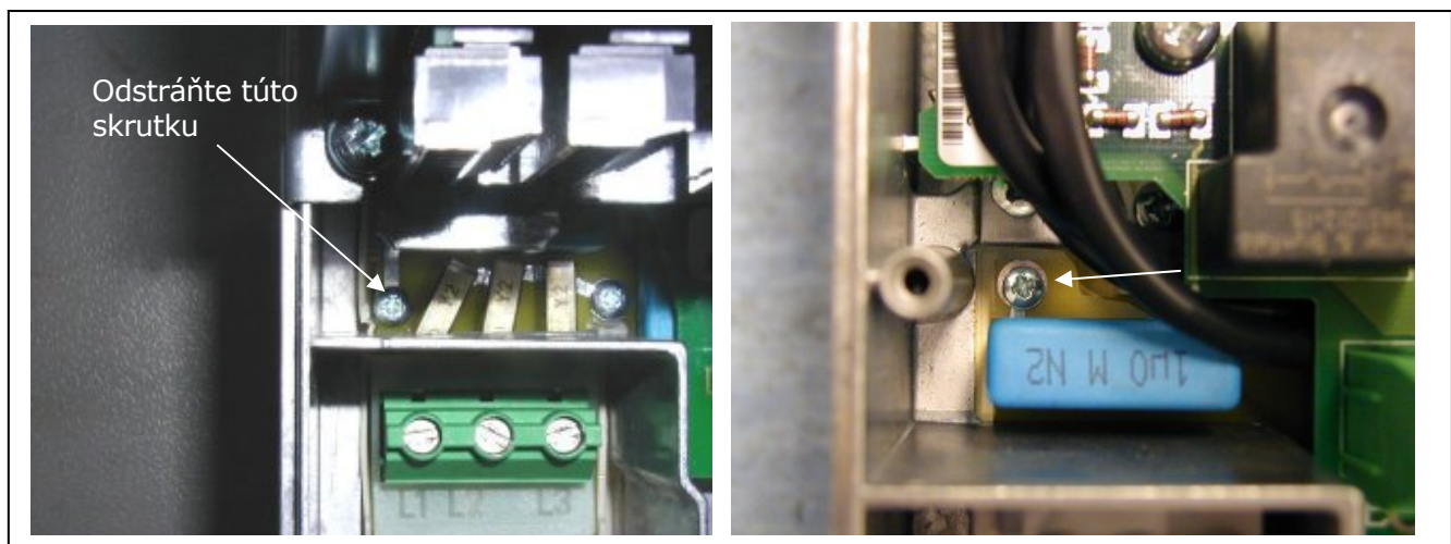
Obr. 6-2. Zmena triedy EMC, FR4 (vľavo) a FR5 (vpravo). Najprv odstráňte kryt káblov.
