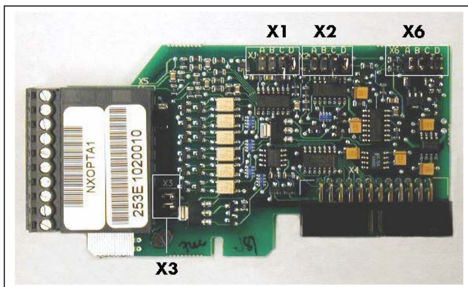
Obr. 6-28. Bloky prepojok na NXOPTA1
