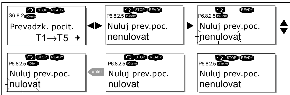
Obr. 7-24. Nulovanie počítadla
