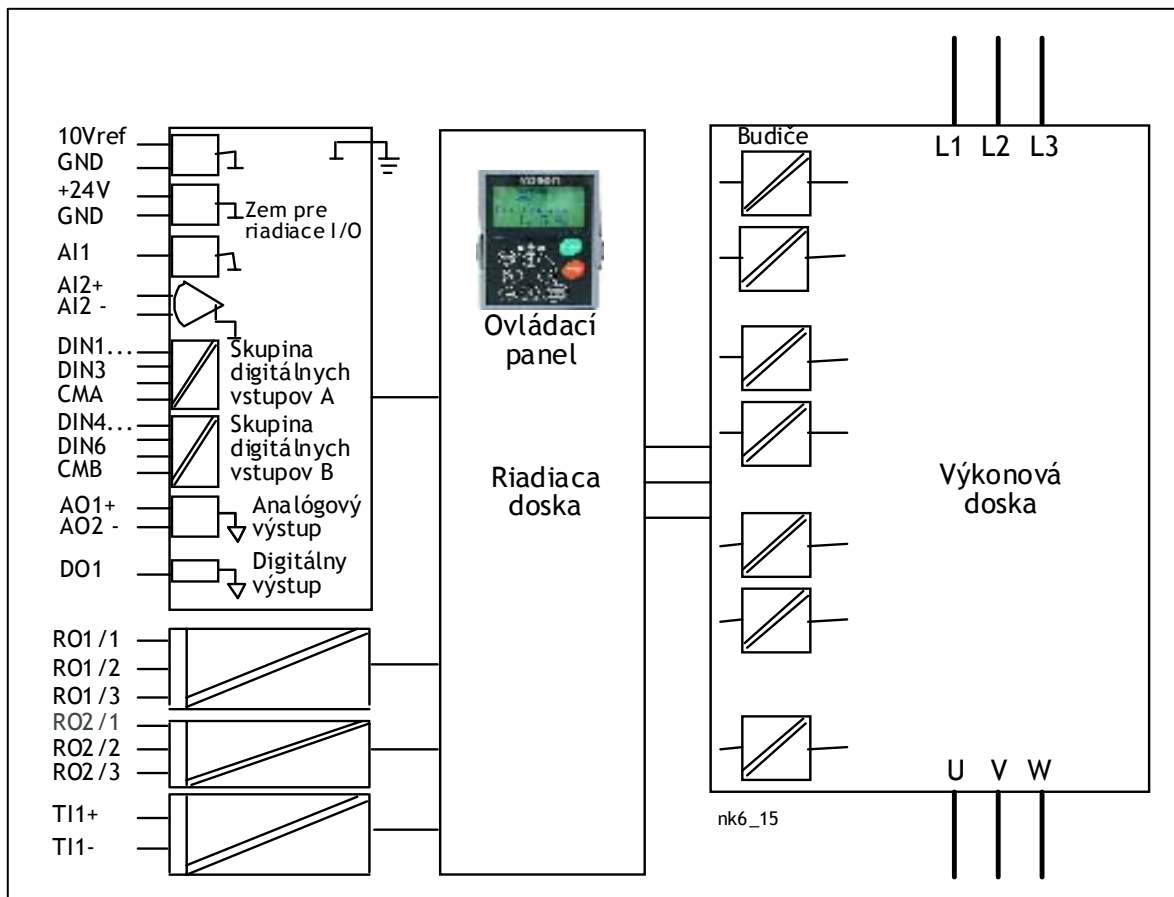
Obr. 6-26. Galvanické oddelenie
