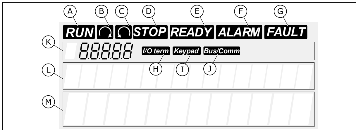
图 29: 显示屏指示
