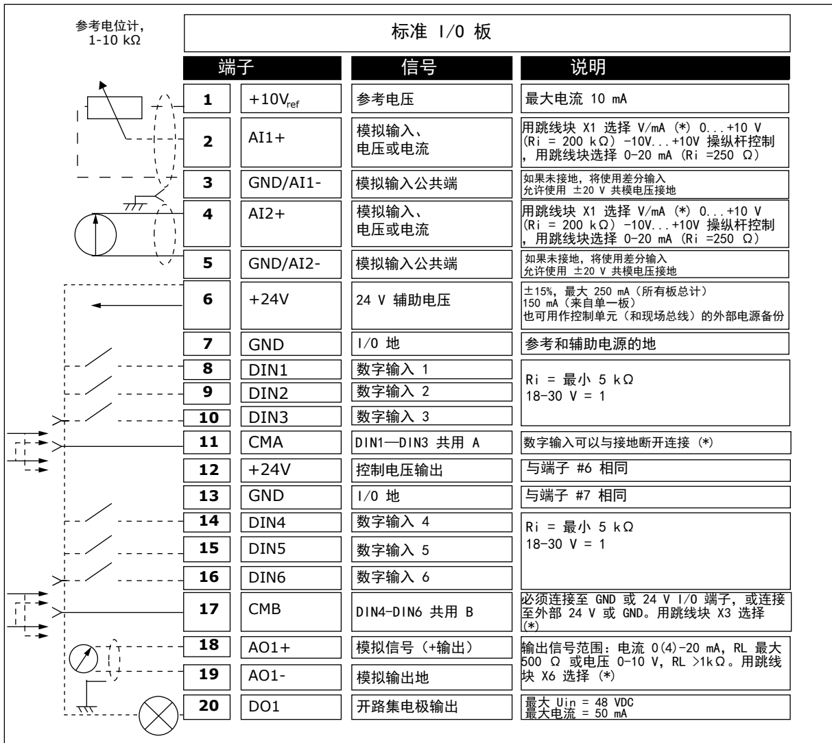
图 22: OPTA1 中的控制端子信号
