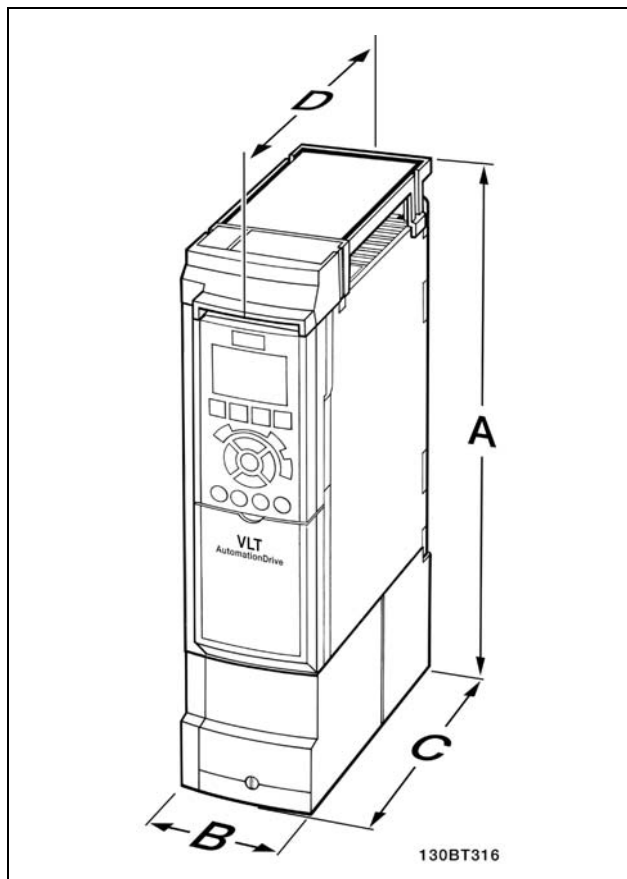
Dimensioni meccaniche del kit contenitore con livello di protezione IP 21/IP 4x/ TIPO 1
