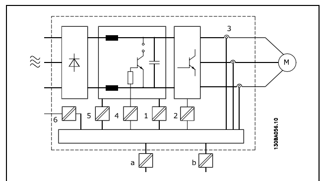
Isolamento galvanico
