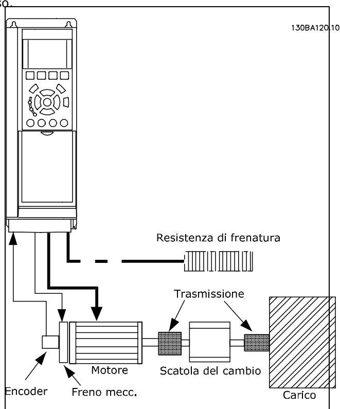
Impostazione di base per la regolazione di velocità ad anello chiuso dell'FC 302
