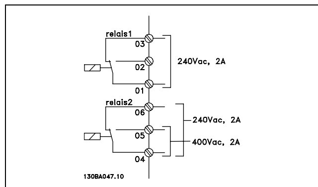
Klemmen voor aansluiten relais.
