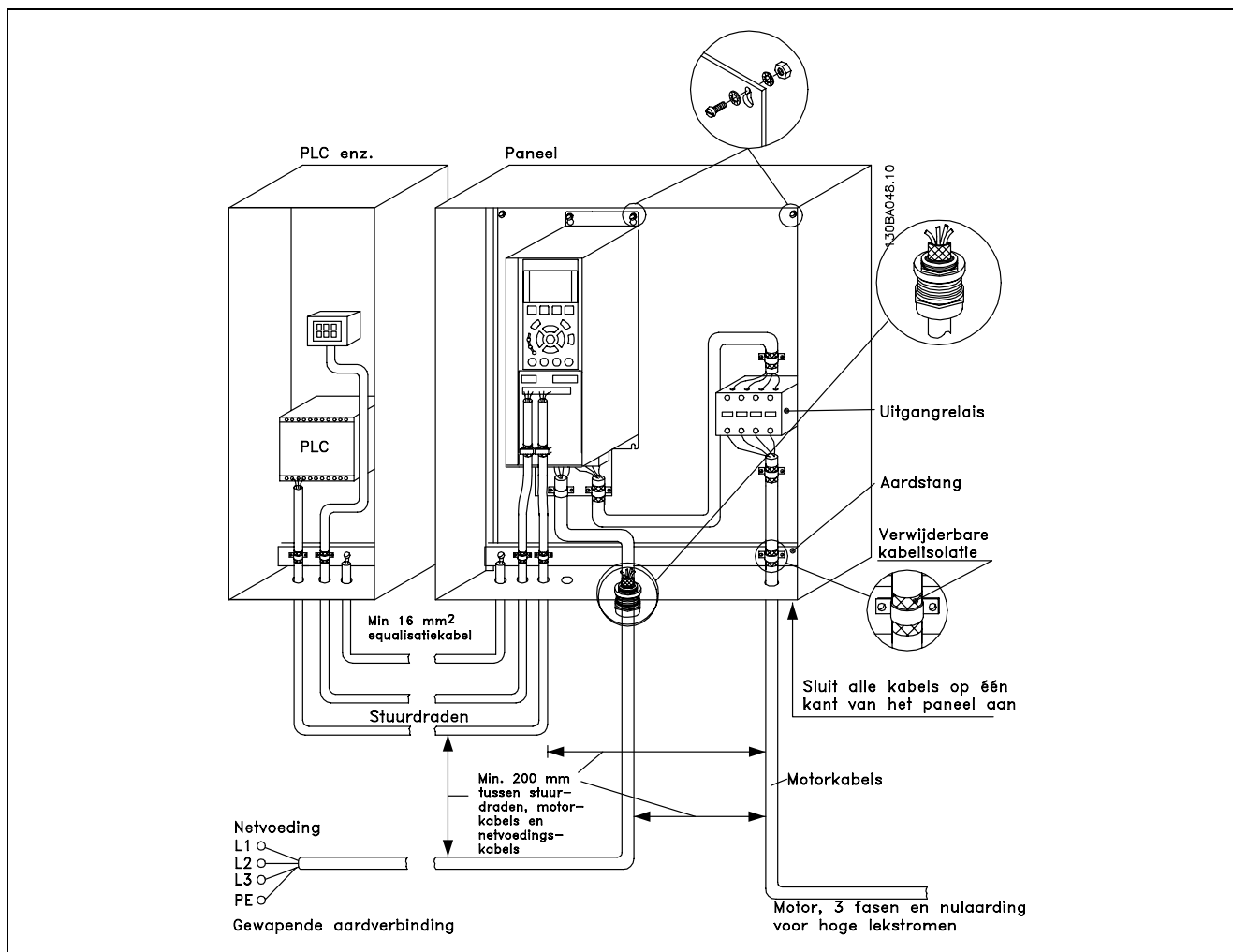
EMC-correcte elektrische installatie van een IP 20-frequentieomvormer.
