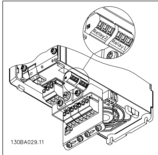
Klemmen voor aansluiten relais.
