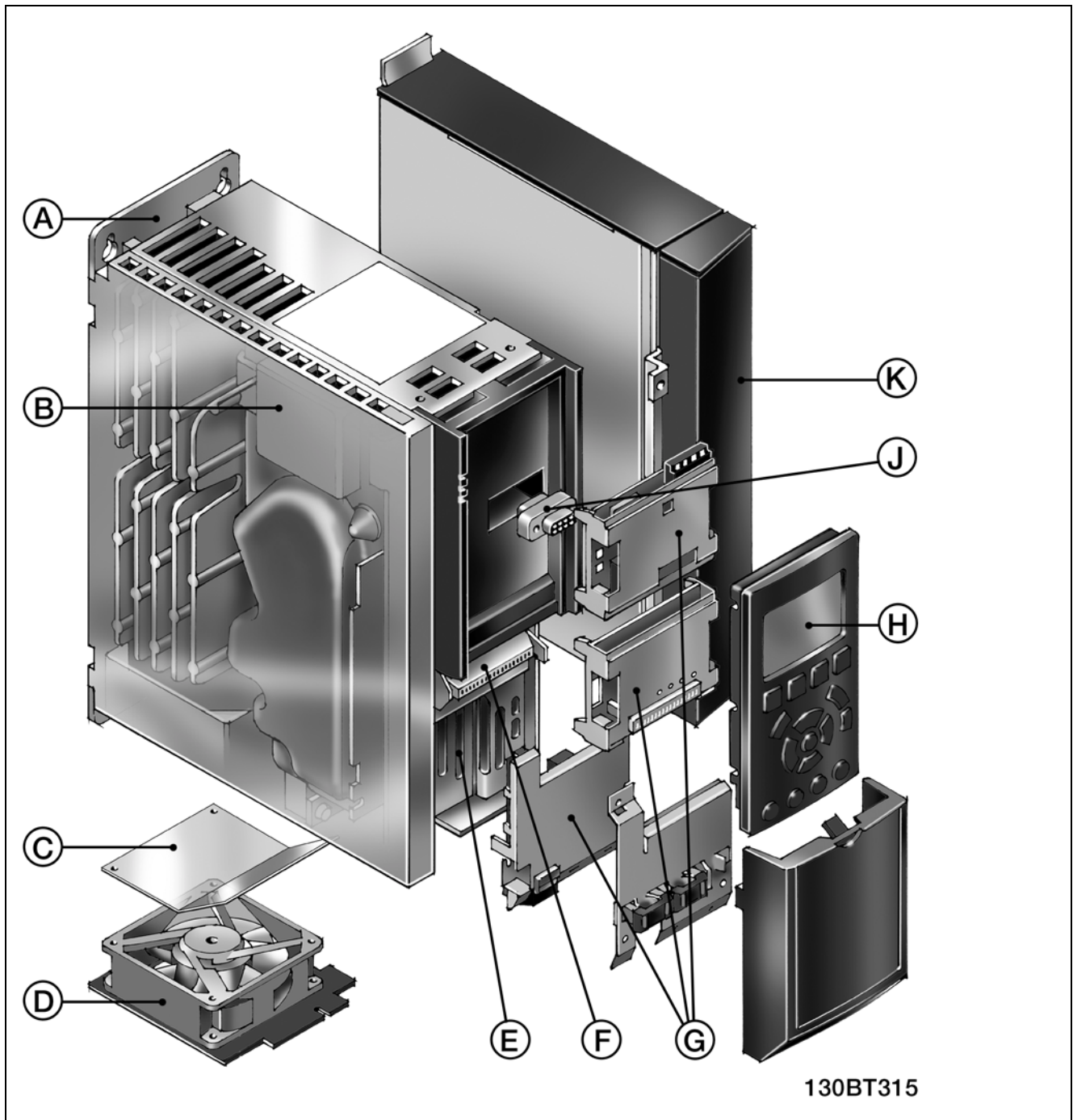
Afbeelding van de mechanische opbouw van de FC 300. De exacte afmetingen van de eenheid staan in hoofdstuk Installeren .
