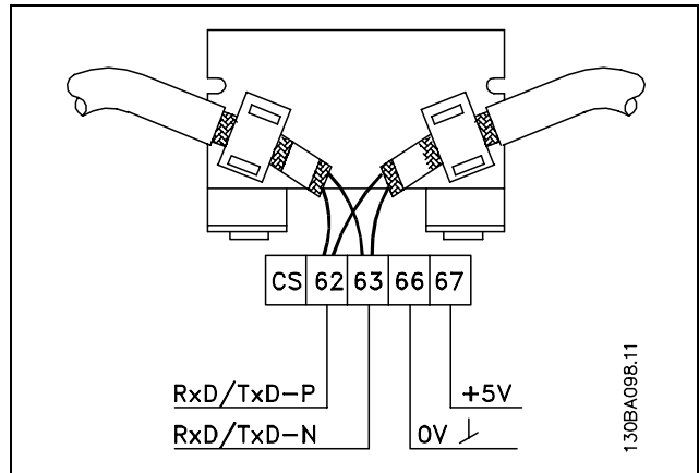
62 = RxD/TxD-P rotes Kabel (Siemens B) 63 = RxD/TxD-N grünes Kabel (Siemens A)
