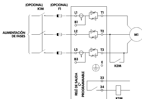
* Par. 38 = 1 (Control Del Contactor Del Freno D.C.)
