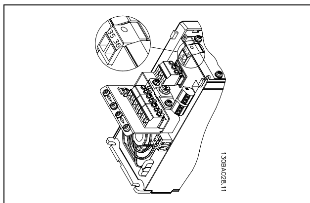
Connexion au fournisseur de back-up de 24 V.
