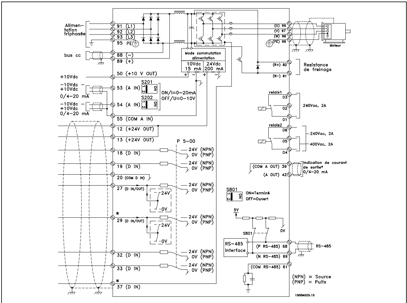
Diagramme présentant toutes les bornes électriques. La borne 37 n'est pas comprise dans le FC 301.
