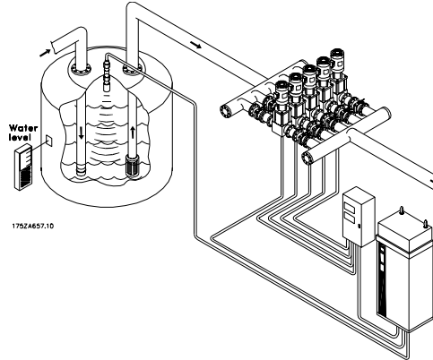
Niveaustyring i standardkaskadestyringsfunktion
