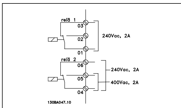
Plintar för reläanslutning.
