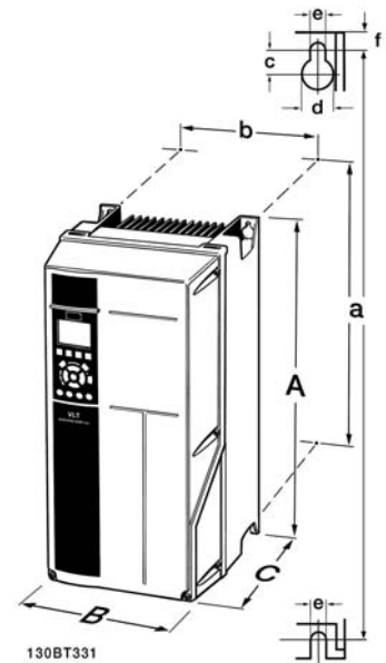
IP 21/IP 4x/ TYPE 1/IP55/TYPE 12 (11-22 kW) 的机械尺寸 A5 + B1 + B2
