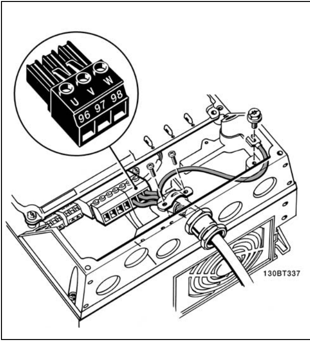
电动机连接 \leq 7.5 kW IP 55/NEMA type 12
