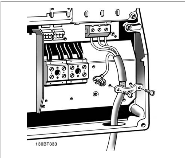
电动机连接 11-22 kW IP 21/NEMA type 1 (B1 和 B2 机箱)
