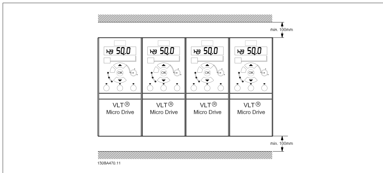
Slika 2.2: Uporedna montaža.
