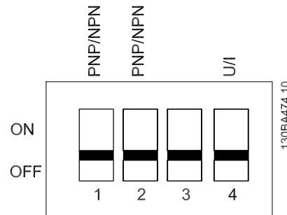
그림 1.4 S200 스위치 1-4
