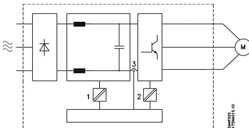
Aislamiento galvánico
