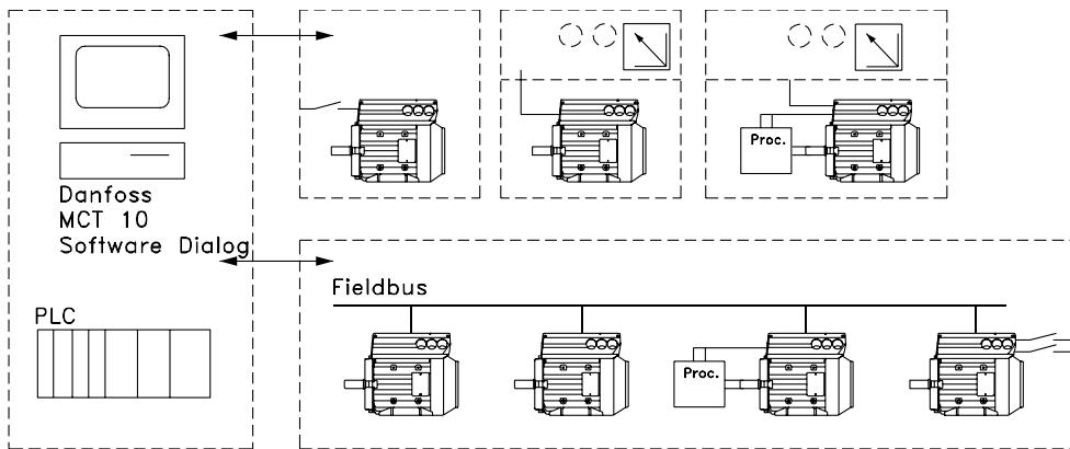
Steuerungsaufbau
