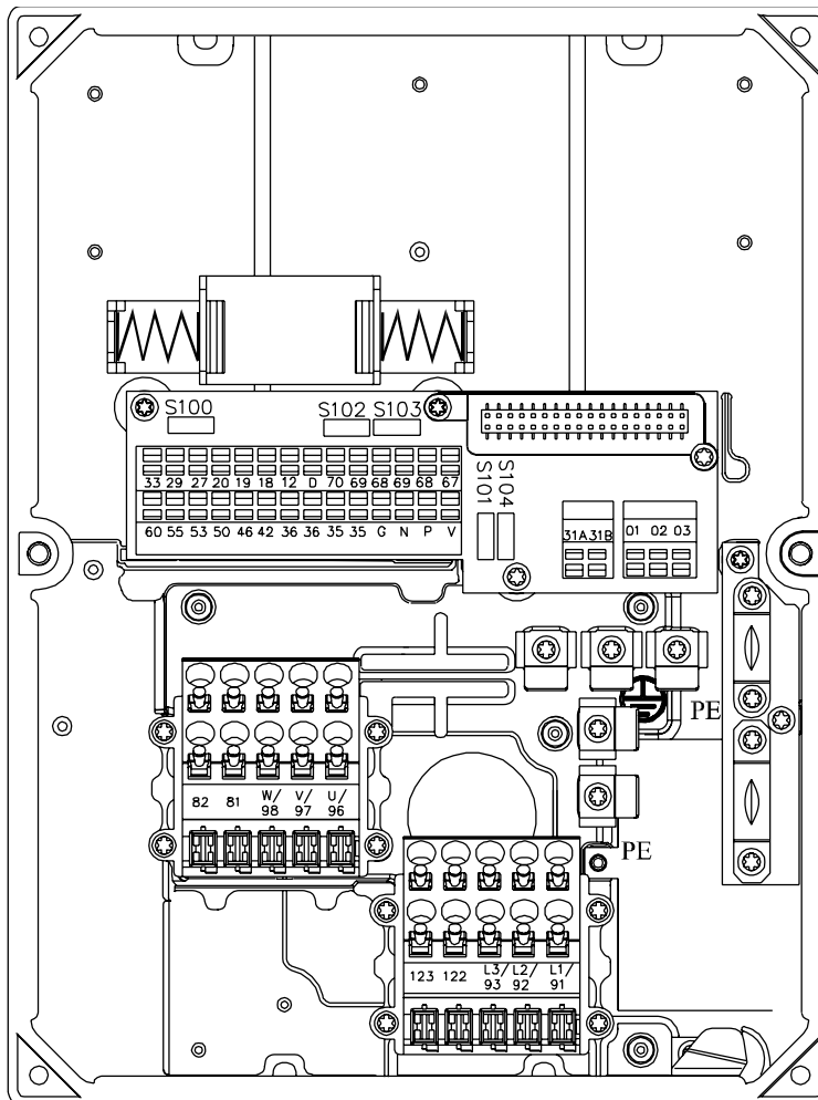
Ilustración 2.4: T12, T16, T52, T56
