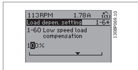
Illustration 6.12: Displayvoorbeeld
