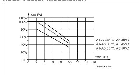
Illustration 8.2: Reductie van I_{out} voor verschillende T_{AMB,MAX} voor behuizing A, bij gebruik van SFAVM
