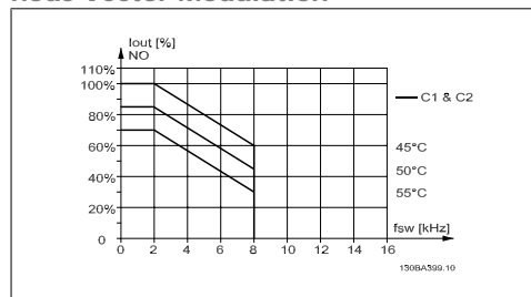
Illustration 8.8: Reductie van I out voor verschillende T AMB,MAX voor behuizing C, bij gebruik van SFAVM en een normaal koppel (overbelastingskoppel van 110%)
