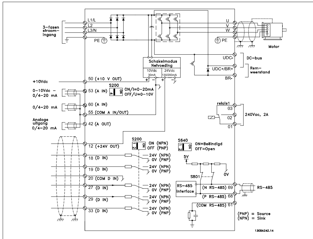
Illustration 4.28: Schema met alle elektrische klemmen. (Klem 37 is enkel aanwezig bij eenheden met de functie Veilige stop.)
