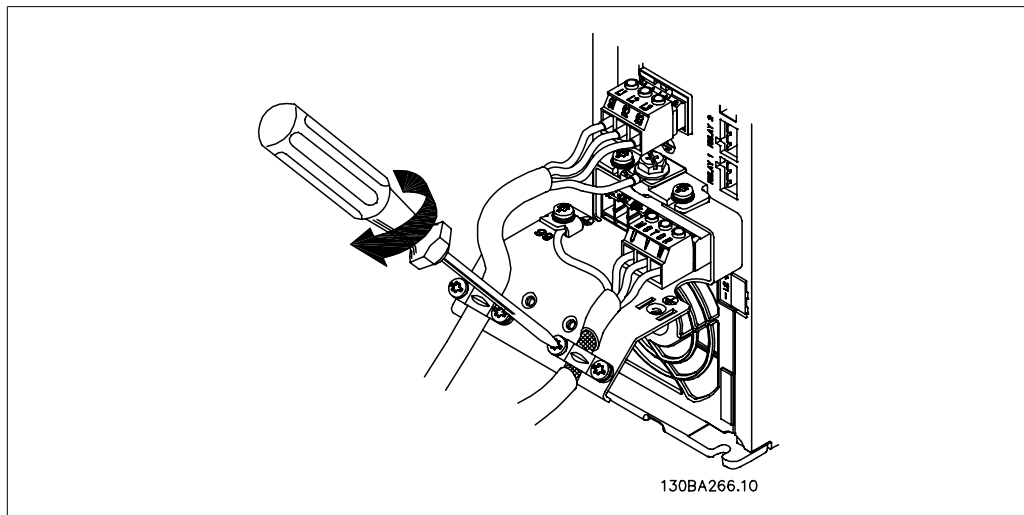
Illustration 4.12: Monteer de kabelklem om te zorgen voor een aansluiting van 360 graden tussen chassis en afscherming. Zorg ervoor dat de buitenste isolatie van de motorkabel onder de kabelklem is verwijderd.
