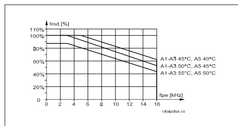
Illustration 8.3: Reductie van I_{out} voor verschillende T_{AMB,MAX} voor behuizing A, bij gebruik van 60 PWM en een motorkabel van maximaal 10 m
