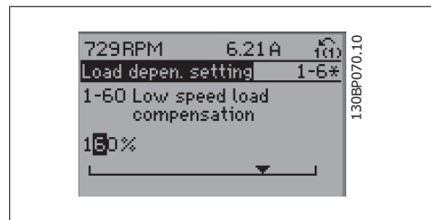
Illustration 6.13: Displayvoorbeeld
