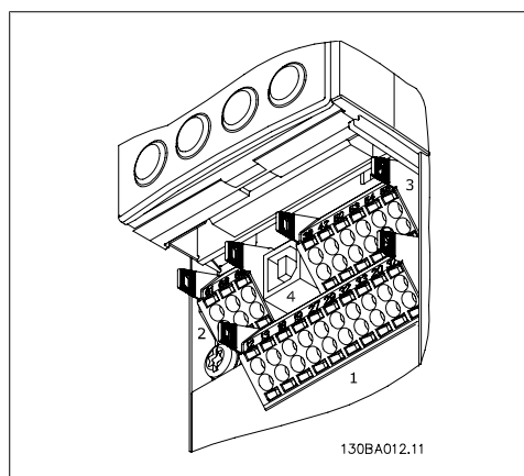
Illustration 4.18: Stuurklemmen (alle behuizingen)
