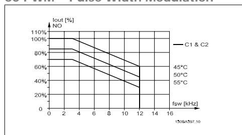
Illustration 8.7: Reductie van I out voor verschillende T AMB,MAX voor behuizing C, bij gebruik van 60 PWM en een normaal koppel (overbelastingskoppel van 110%)
