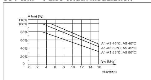
Illustration 8.1: Reductie van I_{out} voor verschillende T_{AMB,MAX} voor behuizing A, bij gebruik van 60 PWM
