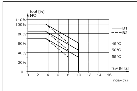
Illustration 8.6: Reductie van I out voor verschillende T AMB,MAX voor behuizing B, bij gebruik van SFAVM en een normaal koppel (overbelastingskoppel van 110%)
