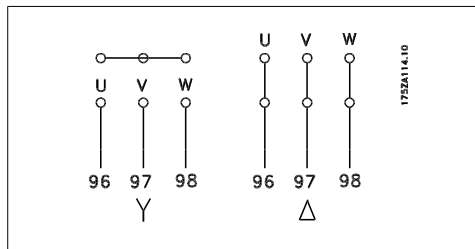
Illustration 4.10: Klemmen voor motoraansluiting
