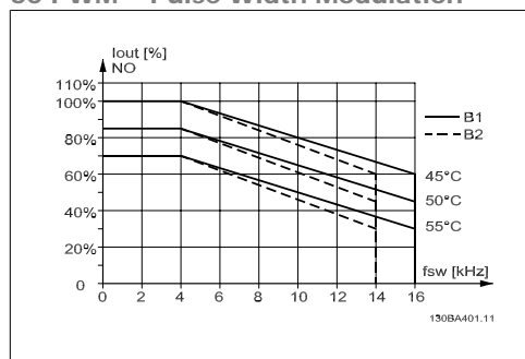
Illustration 8.5: Reductie van I out voor verschillende T AMB,MAX voor behuizing B, bij gebruik van 60 PWM en een normaal koppel (overbelastingskoppel van 110%)
