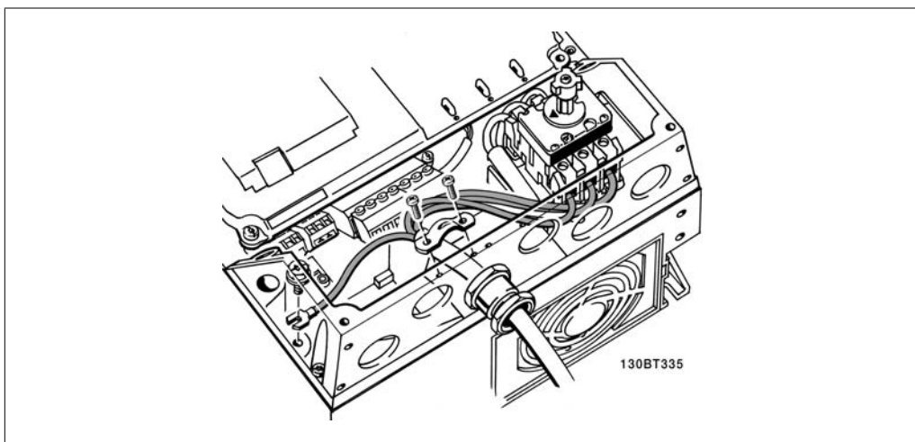
Illustration 4.7: Aansluiting op net en aarding met netschakelaar.
