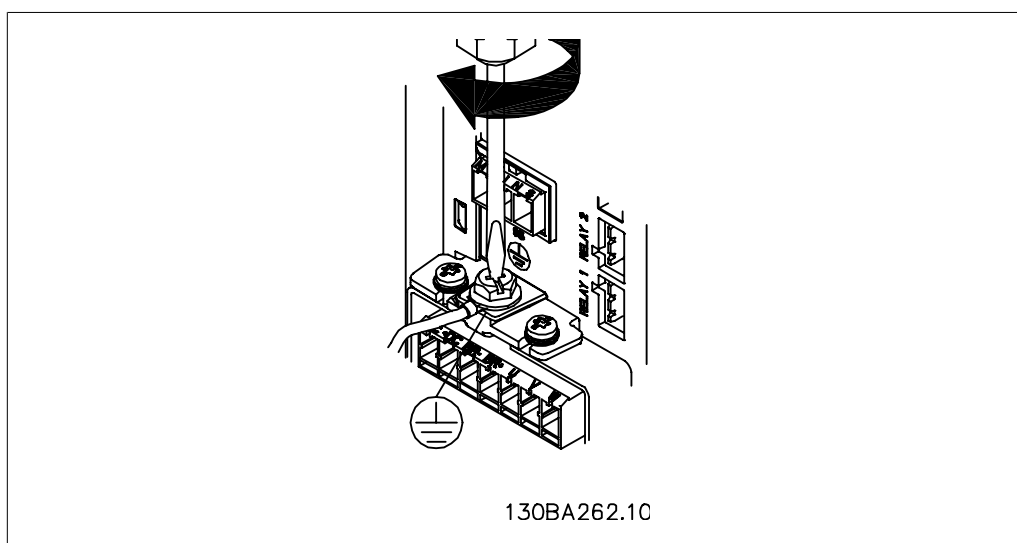
Illustration 4.3: Bij het monteren van kabels dient u eerst de aardkabel te monteren en vast te zetten.
