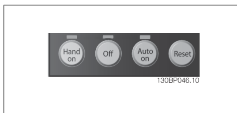
Illustration 5.5: Bedieningstoetsen van het numerieke LCP (NLCP)
