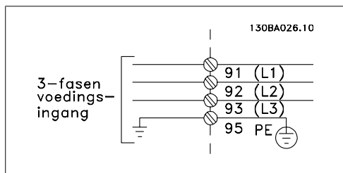
Illustration 4.1: Klemmen voor netvoeding en aarding.
