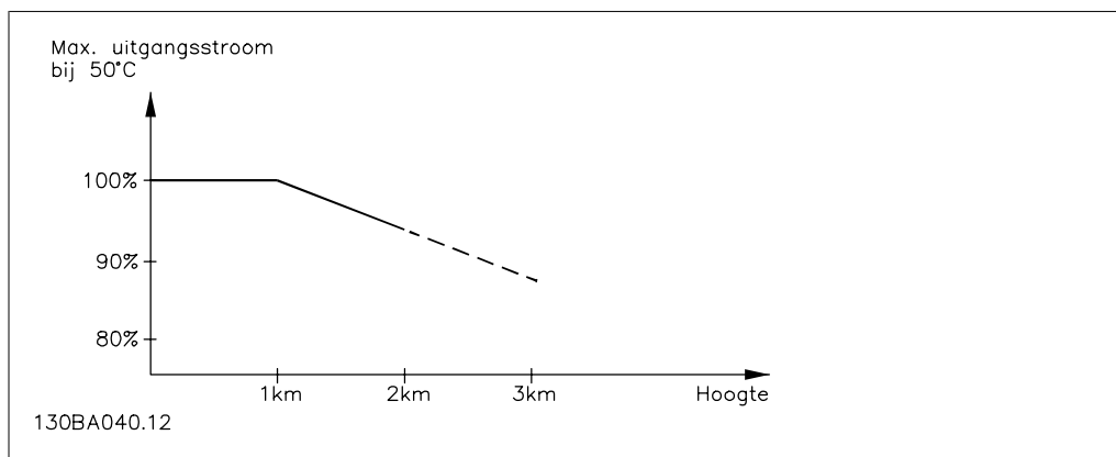
Illustration 8.9: Reductie van de uitgangsstroom t.o.v. de hoogte bij T_{AMB,MAX} . Voor hoogtes boven de 2000 m dient u contact op te nemen met Danfoss Drives in verband met PELV.
