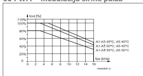
Illustration 8.1: Zmanjšanje zmogljivosti I_{out} za različne T_{AMB, MAX} za ohišje A, ob uporabi 60 PWM
