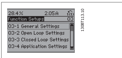
Illustration 6.5: Korak 4: Prikažejo se izbire nastavitvev funkcij. Izberite 03-1 Sploš. nastavitve . Pritisnite [OK].
