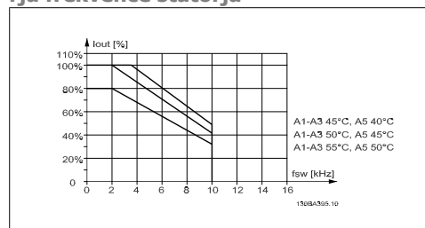
Illustration 8.2: Zmanjšanje zmogljivosti I_{out} za različne T_{AMB, MAX} za ohišje A, ob uporabi SFAVM
