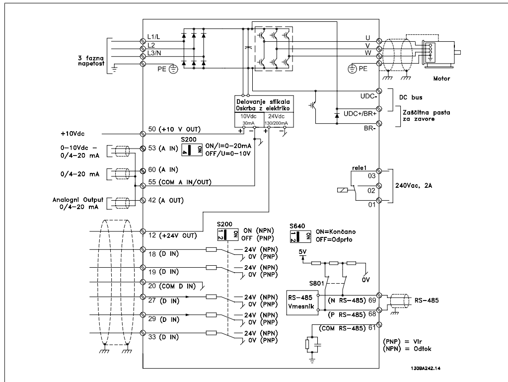
Illustration 4.28: Shema prikazuje vse električne sponke. (Sponka 37 obstaja samo pri enotah s funkcijo za varno zaustavitev.)
