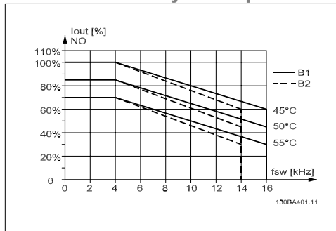
Illustration 8.5: Zmanjšanje zmogljivosti I_{out} za različne T_{AMB, MAX} za ohišje B, ob uporabi 60 PWM z normalnim navorom (110 % nad navorom)
