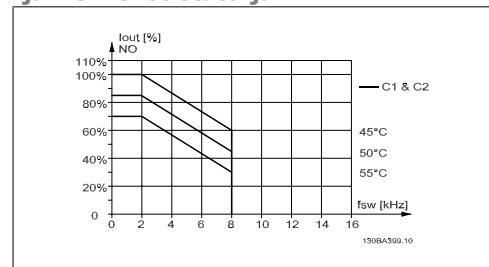
Illustration 8.8: Zmanjšanje zmogljivosti I_{out} za različne T_{AMB, MAX} za ohišje C, ob uporabi SFAVM z normalnim navorom (110 % nad navorom)
