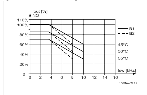
Illustration 8.6: Zmanjšanje zmogljivosti I_{out} za različne T_{AMB, MAX} za ohišje B, ob uporabi SFAVM z normalnim navorom (110 % nad navorom)
