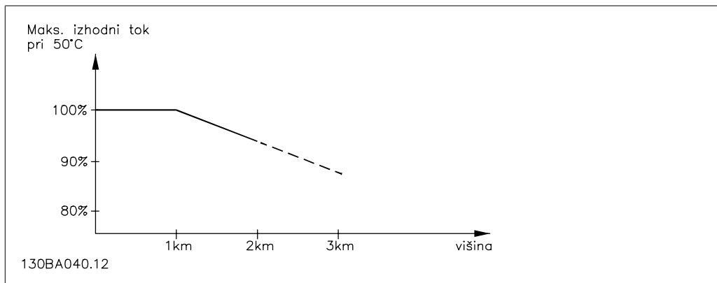
Illustration 8.9: Zmanjšanje izhodnega toka glede na nadmorsko višino pri T_{AMB, MAX} . Pri nadmorskih višinah nad 2 km se obrnite na Danfoss Drives v zvezi s PELV.
