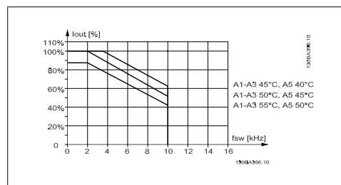
Illustration 8.4: Zmanjšanje zmogljivosti I_{out} za različne T_{AMB, MAX} za ohišje A, ob uporabi SFAVM in največ 10 m kabla za motor.
