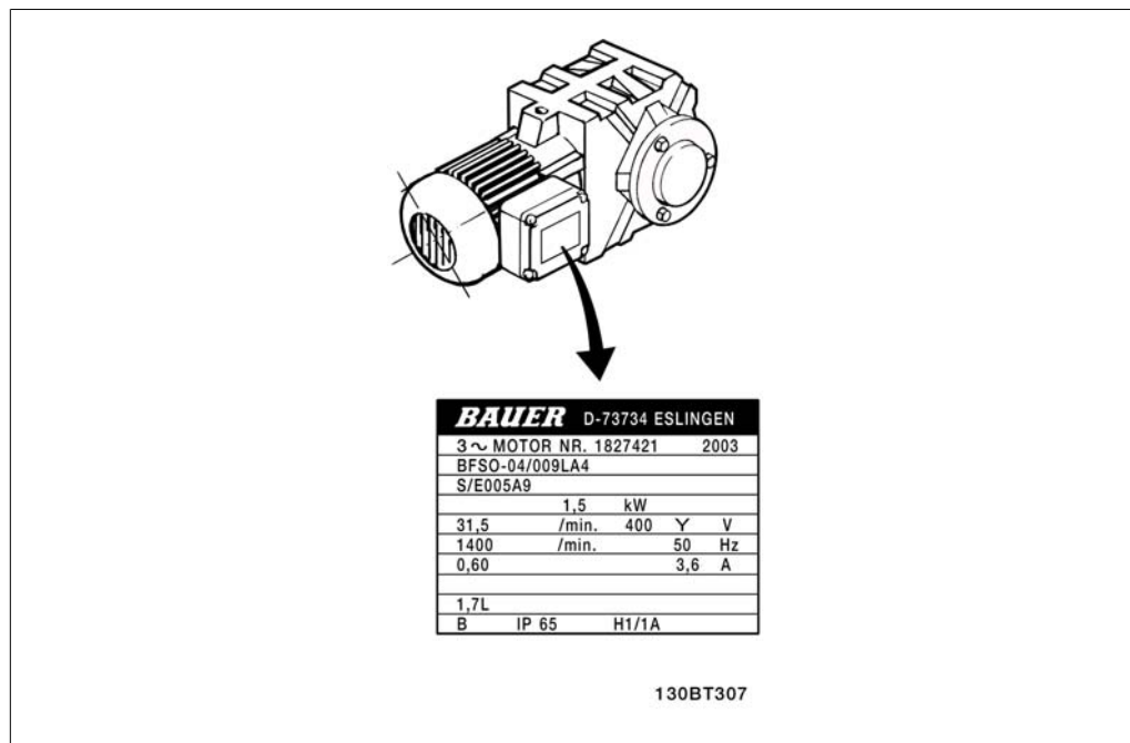
Illustration 4.31: Primer tipske ploščice motorja
