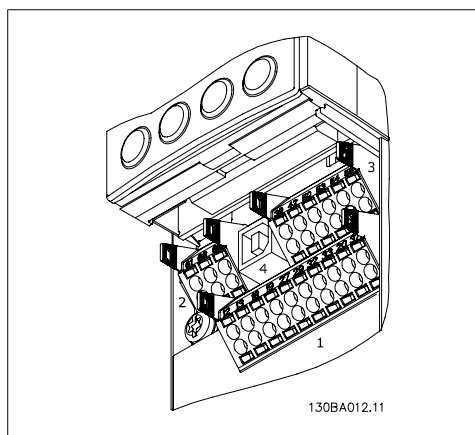
Illustration 4.18: Krmilne sponke (vsa ohišja)
