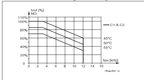
Illustration 8.7: Zmanjšanje zmogljivosti I_{out} za različne T_{AMB, MAX} za ohišje C, ob uporabi 60 PWM z normalnim navorom (110 % nad navorom)
