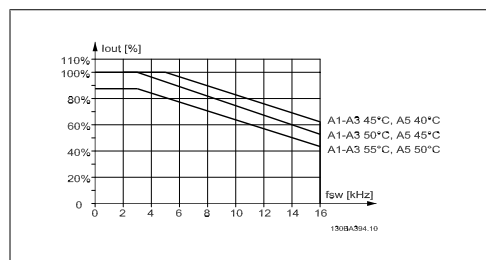
Illustration 8.3: Zmanjšanje zmogljivosti I_{out} za različne T_{AMB, MAX} za ohišje A, ob uporabi 60 PWM in največ 10 m kabla za motor.
