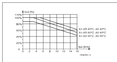
Illustration 8.3: Snížení proudu I_{out} pro různou T_{AMB,MAX} pro krytí A, při použití 60 PWM a max. 10metrového kabelu motoru
