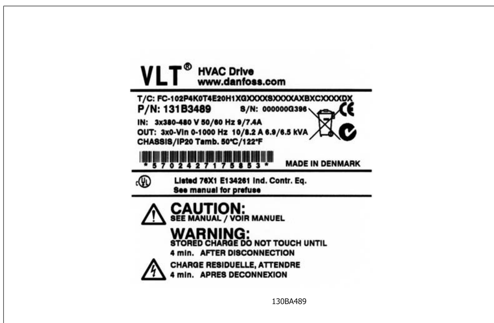
Illustration 2.1: Příklad identifikačního štítku.
