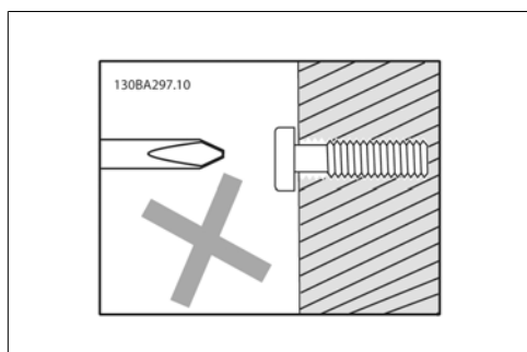
Illustration 3.12: Chybné umístění šroubů
