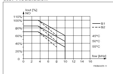
Illustration 8.6: Snížení proudu I_{out} pro různou T_{AMB, MAX} pro krytí B, při použití SFAVM v režimu normálního momentu (110 % momentu)
