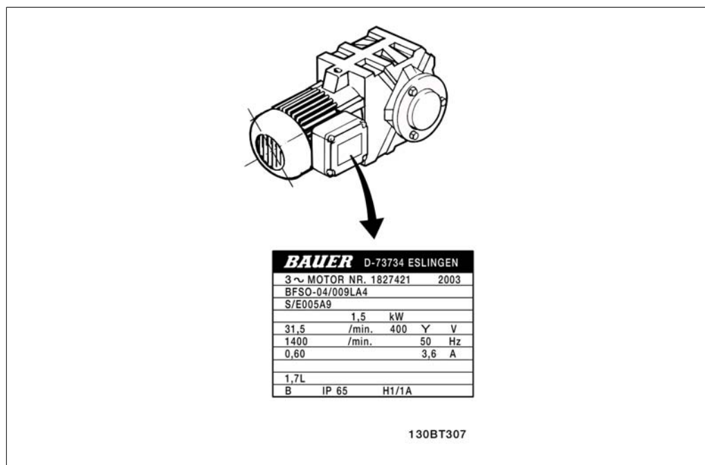
Illustration 4.31: Příklad typového štítku motoru
