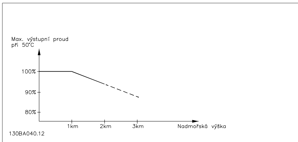
Illustration 8.9: Snížení výstupního proudu v závislosti na nadmořské výšce při T_{AMB, MAX} . V případě nadmořských výšek nad 2 km se ohledně PELV obraťte na společnost Danfoss Drives,
