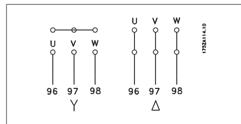
Illustration 4.10: Svorky pro připojení motoru
