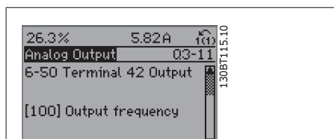
Illustration 6.7: Krok 6: Zvolte parametr 6-50 Svorka 42, výstup . Stiskněte tlačítko [OK].
