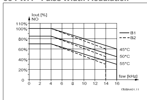
Illustration 8.5: Snížení proudu I_{out} pro různou T_{AMB, MAX} pro krytí B, při použití 60 PWM v režimu normálního momentu (110 % momentu)
