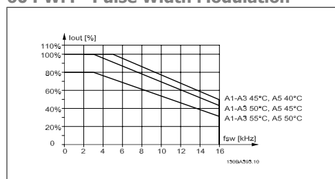
Illustration 8.1: Snížení proudu I_{out} pro různou T_{AMB,MAX} pro krytí A, při použití 60 PWM
