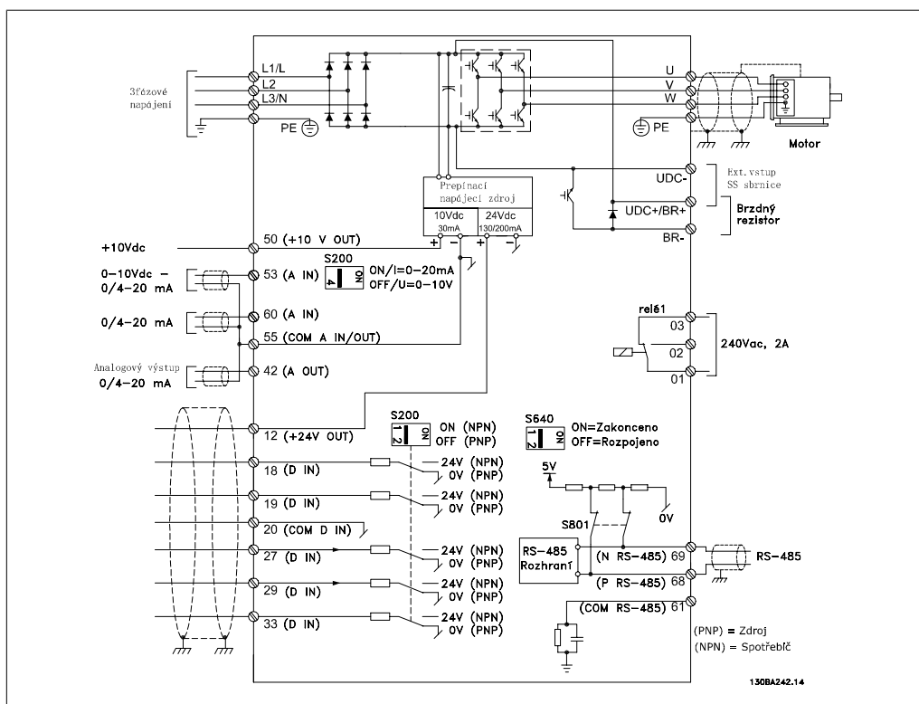
Illustration 4.28: Na schématu jsou zobrazeny všechny elektrické svorky. (Svorka 37 je obsažena pouze v jednotkách s funkcí Bezpečného zastavení.)
