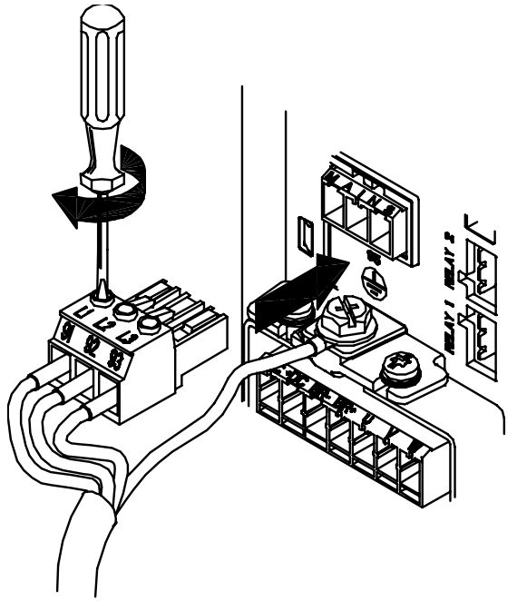
그림 4.4: 그 다음 주전원 플러그를 설치하고 와이어를 조이십시오.
