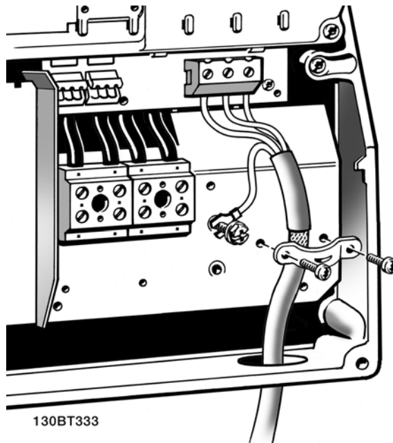
그림 4.14: 먼저 모터 접지를 차단한 다음, 모터 U, V 및 W 와이어를 단자에 놓고 조이십시오. EMC 클램프 아래로 모터 케이블의 외부 절연이 제거되었는지 확인하십시오.
