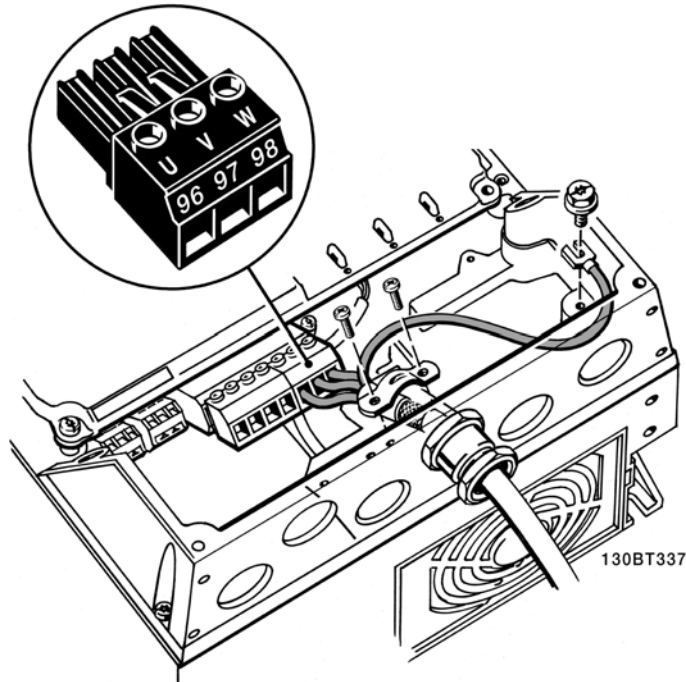
그림 4.13: 먼저 모터 접지를 차단한 다음, 모터 U, V 및 W 와이어를 단자에 놓고 조이십시오. EMC 클램프 아래로 모터 케이블의 외부 절연이 제거되었는지 확인하십시오.
